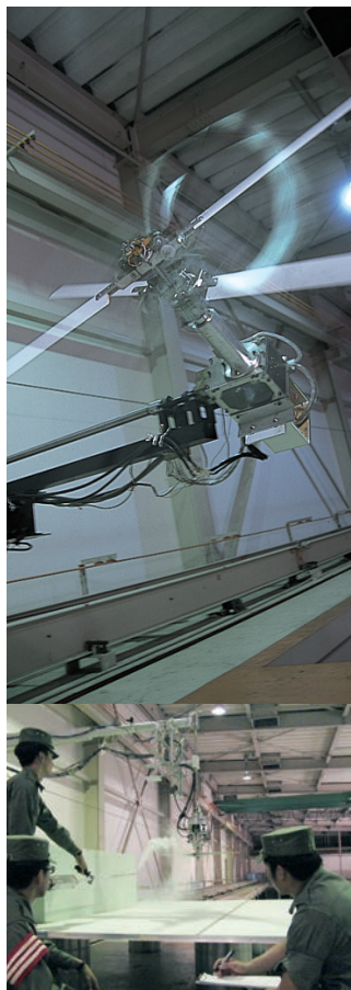
卒業研究（ヘリコプタ実験室）：ヘリコプタ・ロータの力学や流れの様子を飛行特性測定装置により理解する。
