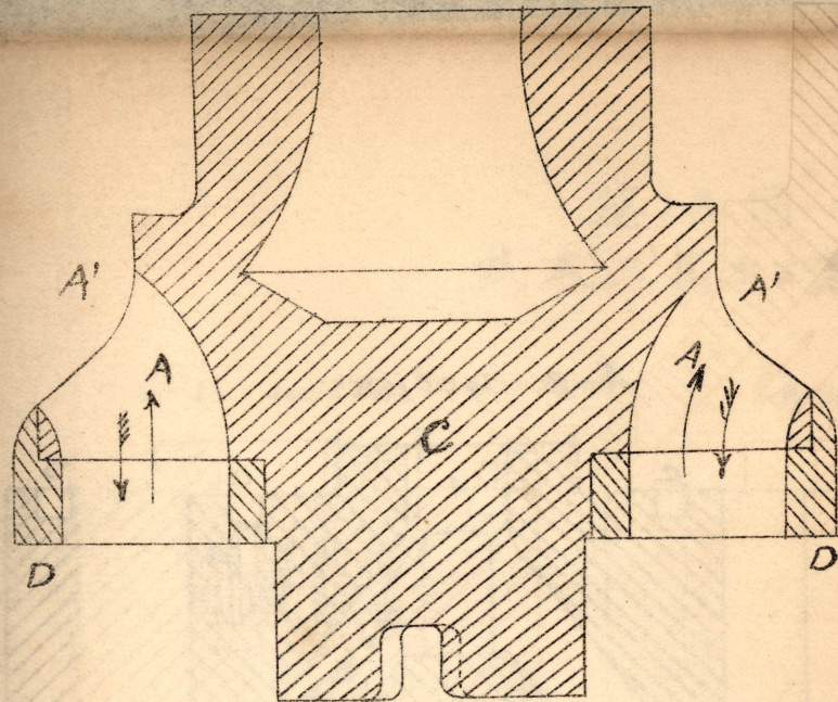
回轉弁面
