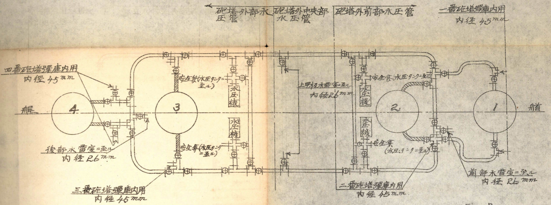
第4圖(一) 軍艦陸奧水壓管裝置
