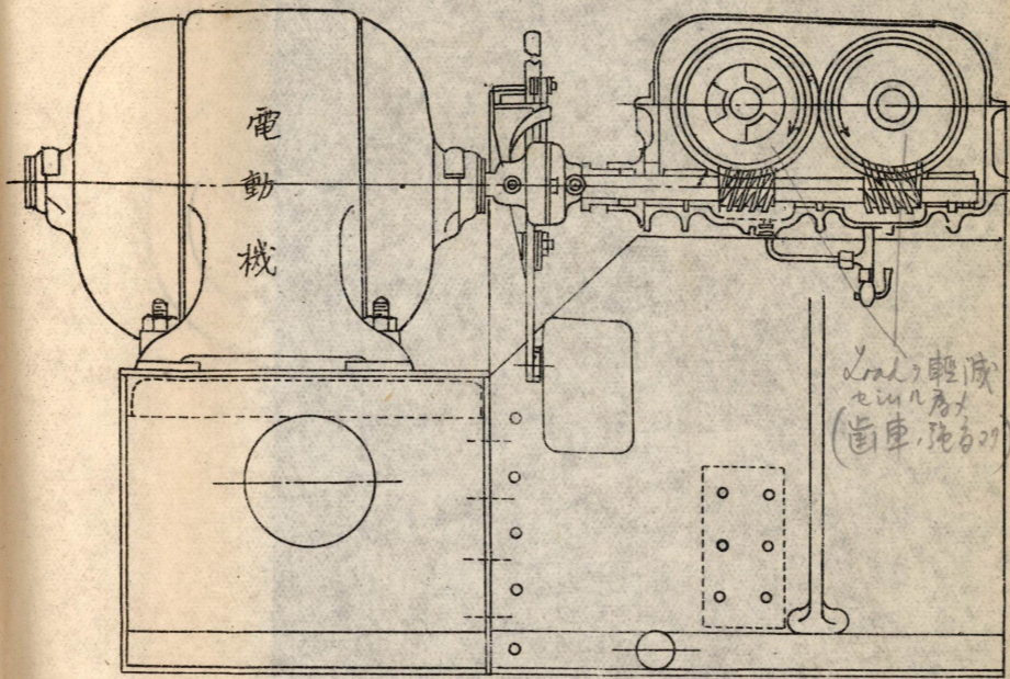
第3圖，一 手動兼電動水壓唧筒機械
