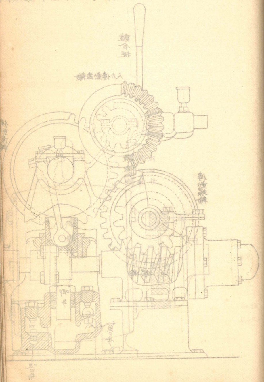
三、圖(二) 軍艦陸奧水壓管裝置
