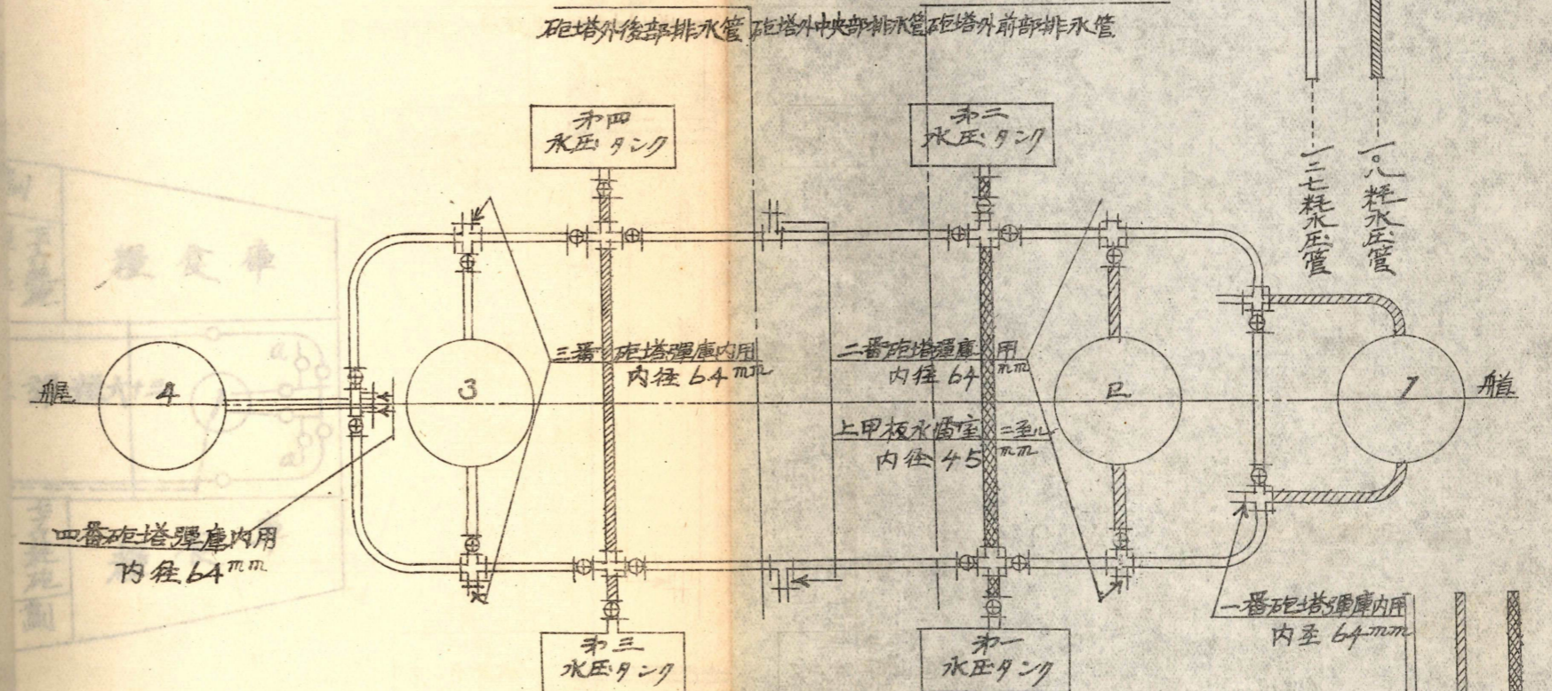
軍艦陸奧 排水管裝置
