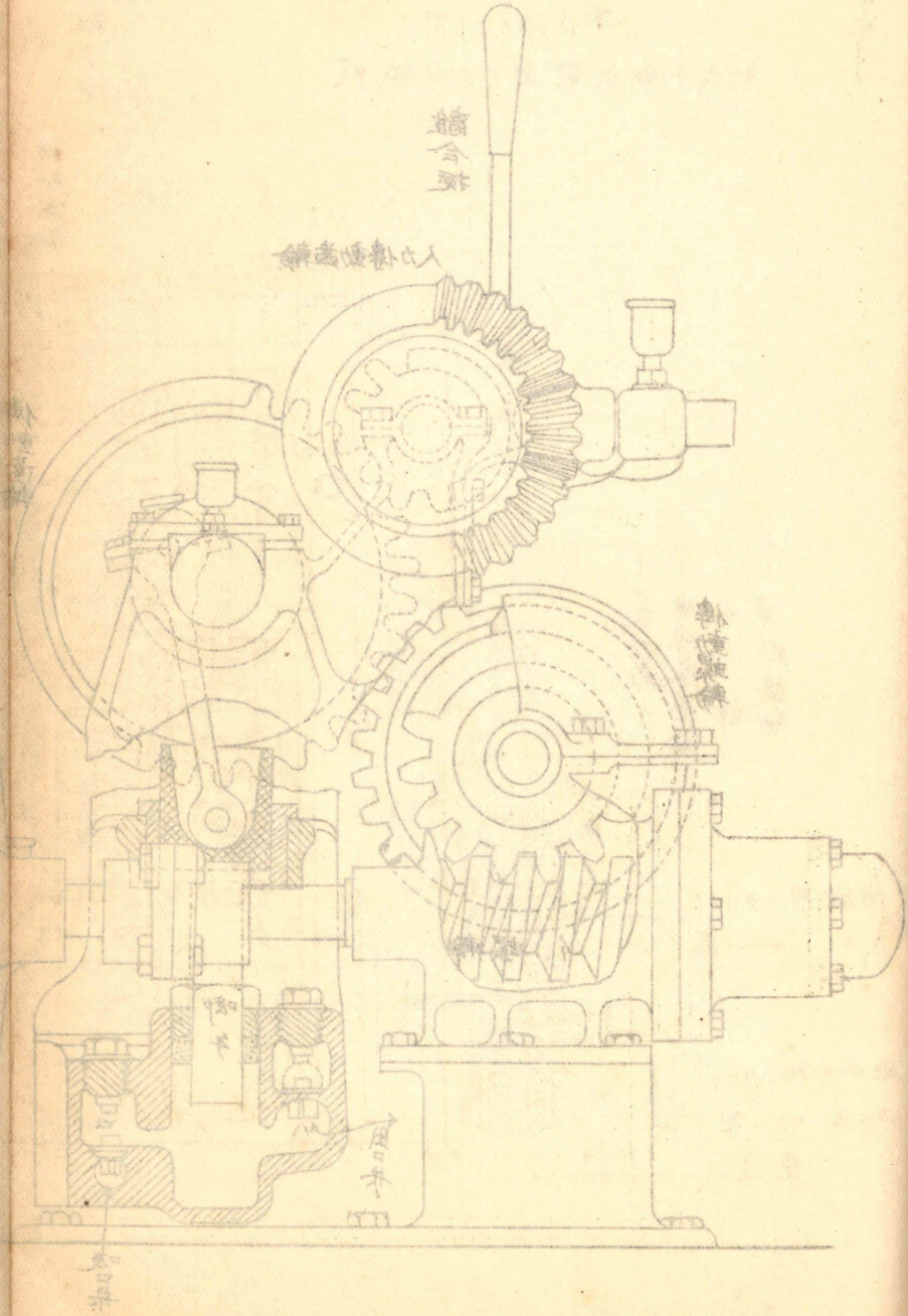
图 6 第 弹壳退壳机构
