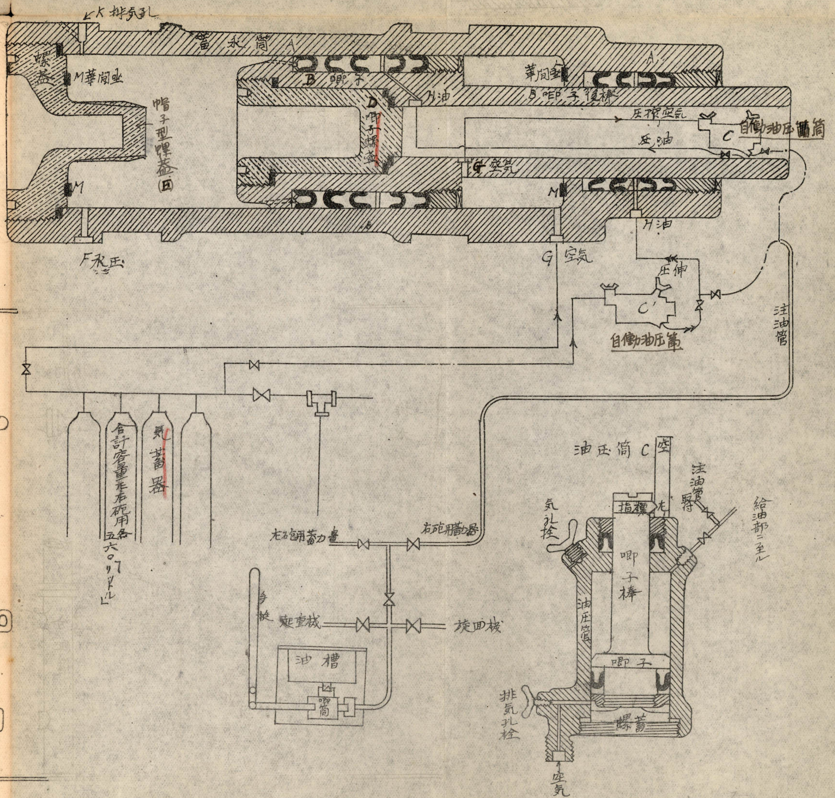
第2图 水庄蓄勢器要領图
