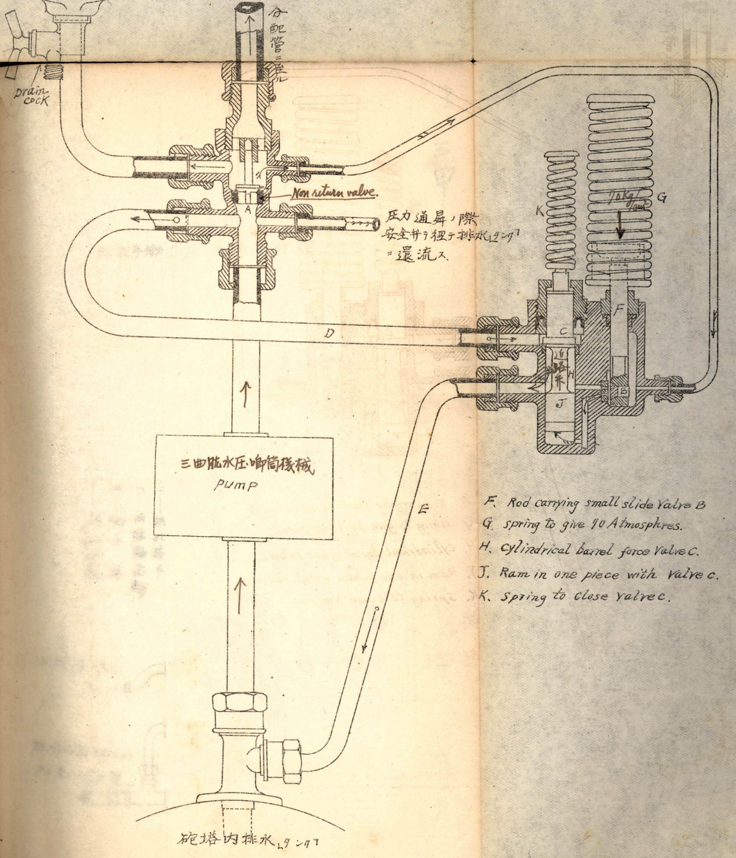
第 3 圖 二 電動唧筒用水壓調節器
