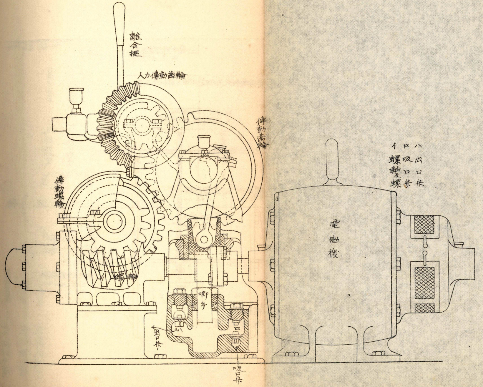
第3圖, 三, 乙 新式電動兼手動唧筒機械
