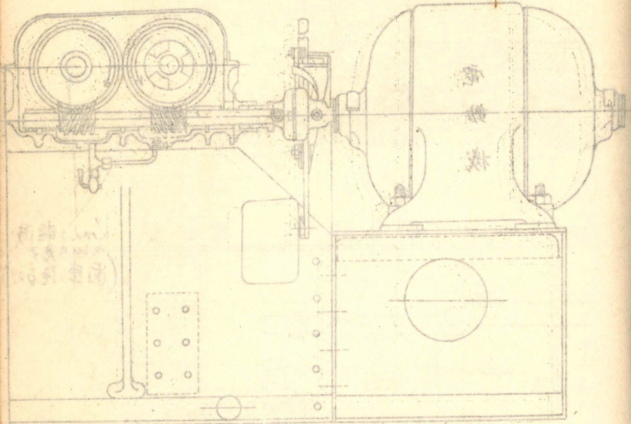
圖 1 三曲肱水壓唧筒機
