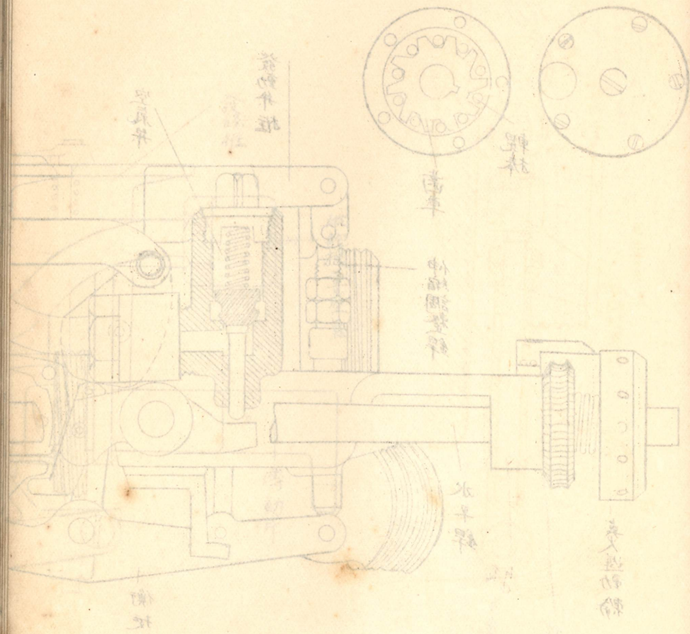
圖八第 置裝動發
