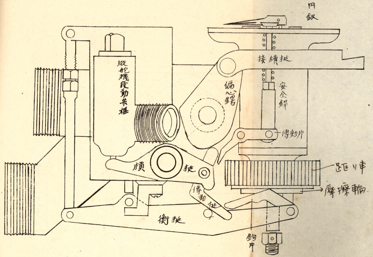
縱舵機發動裝置
