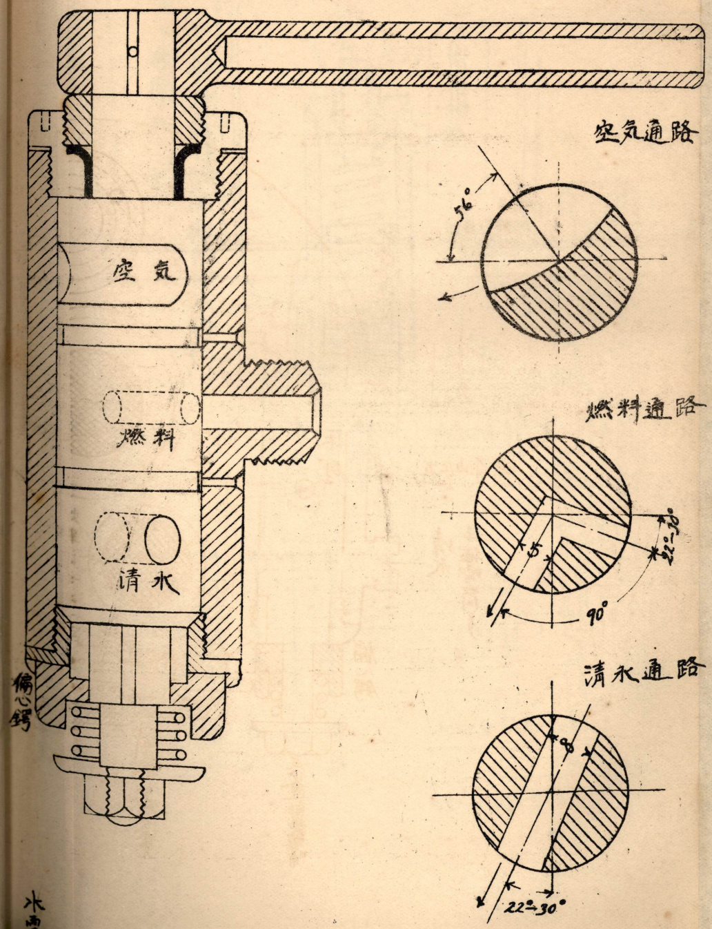
點火遲動用複道嘴及調定輪
