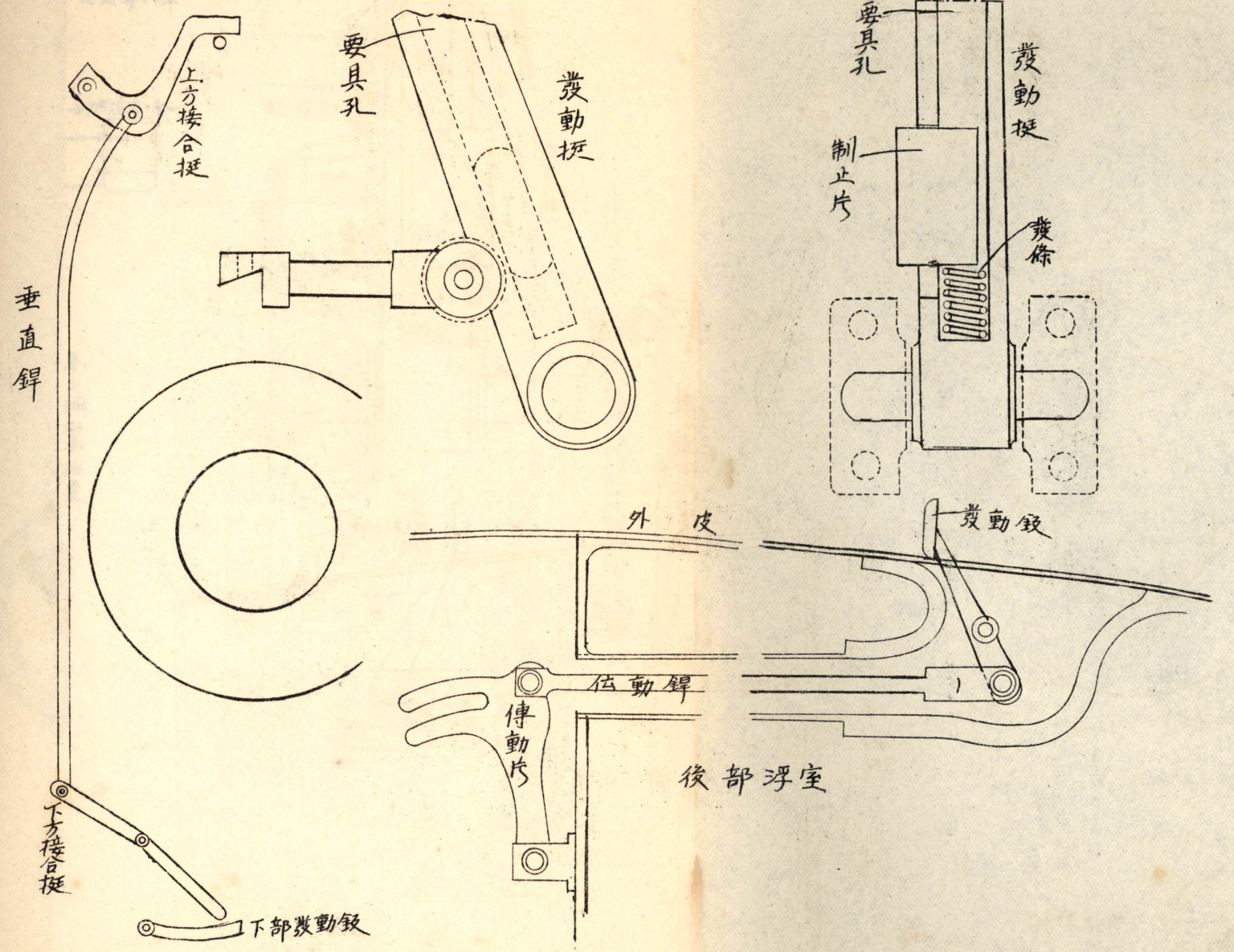
第十二圖 發動挺及發動鉸
