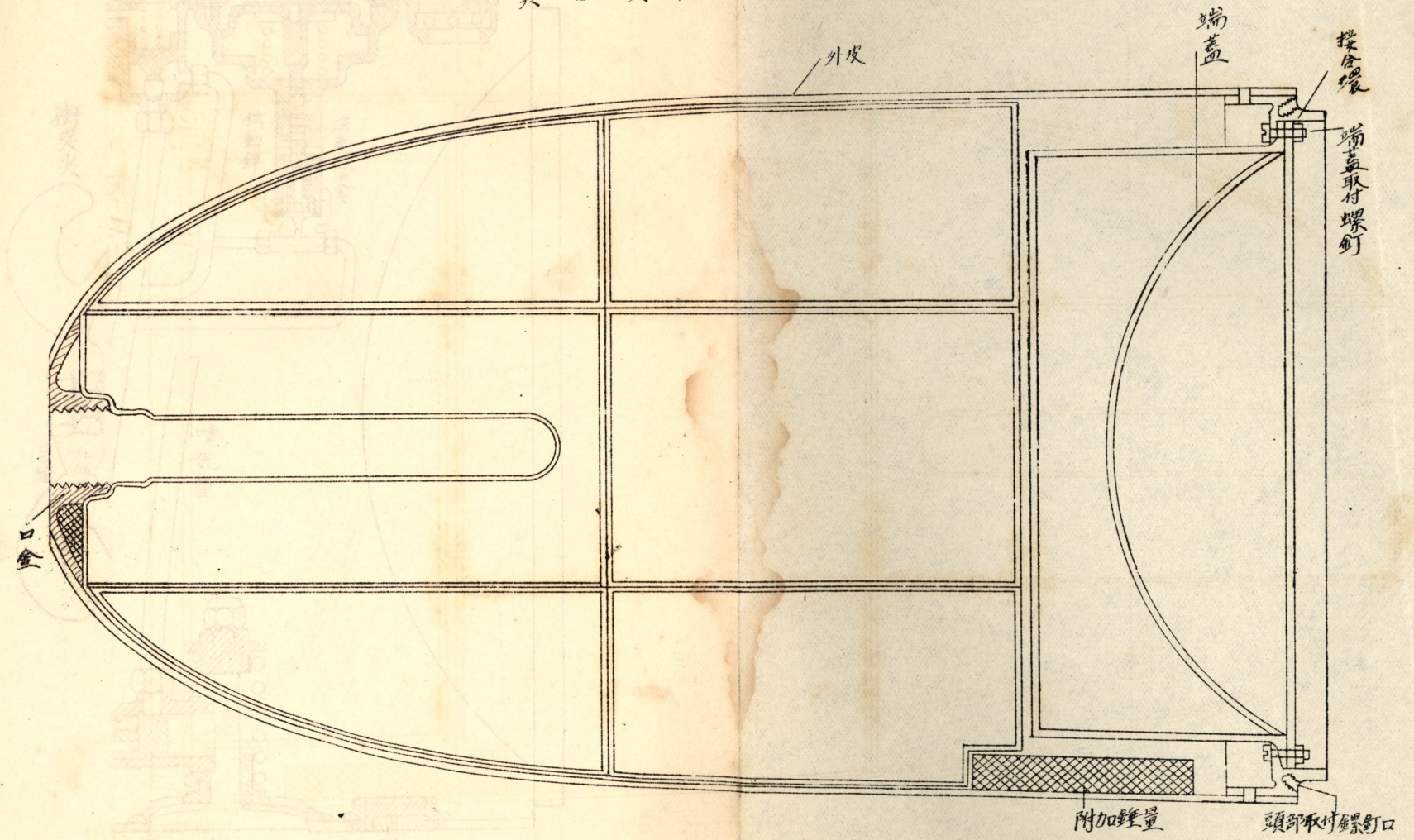
第三圖 實用頭部
