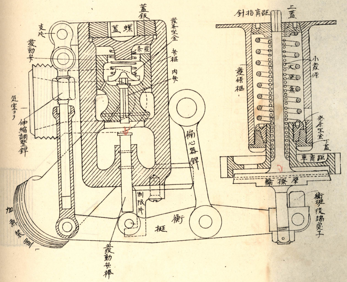
發停裝置
