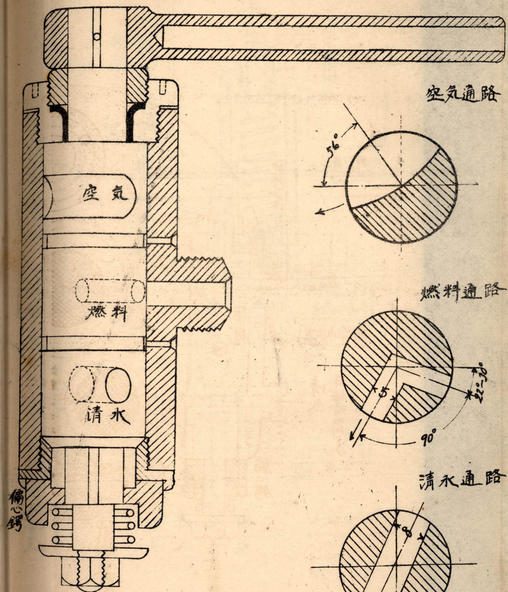
點火運動用複道嘴及調定輪
