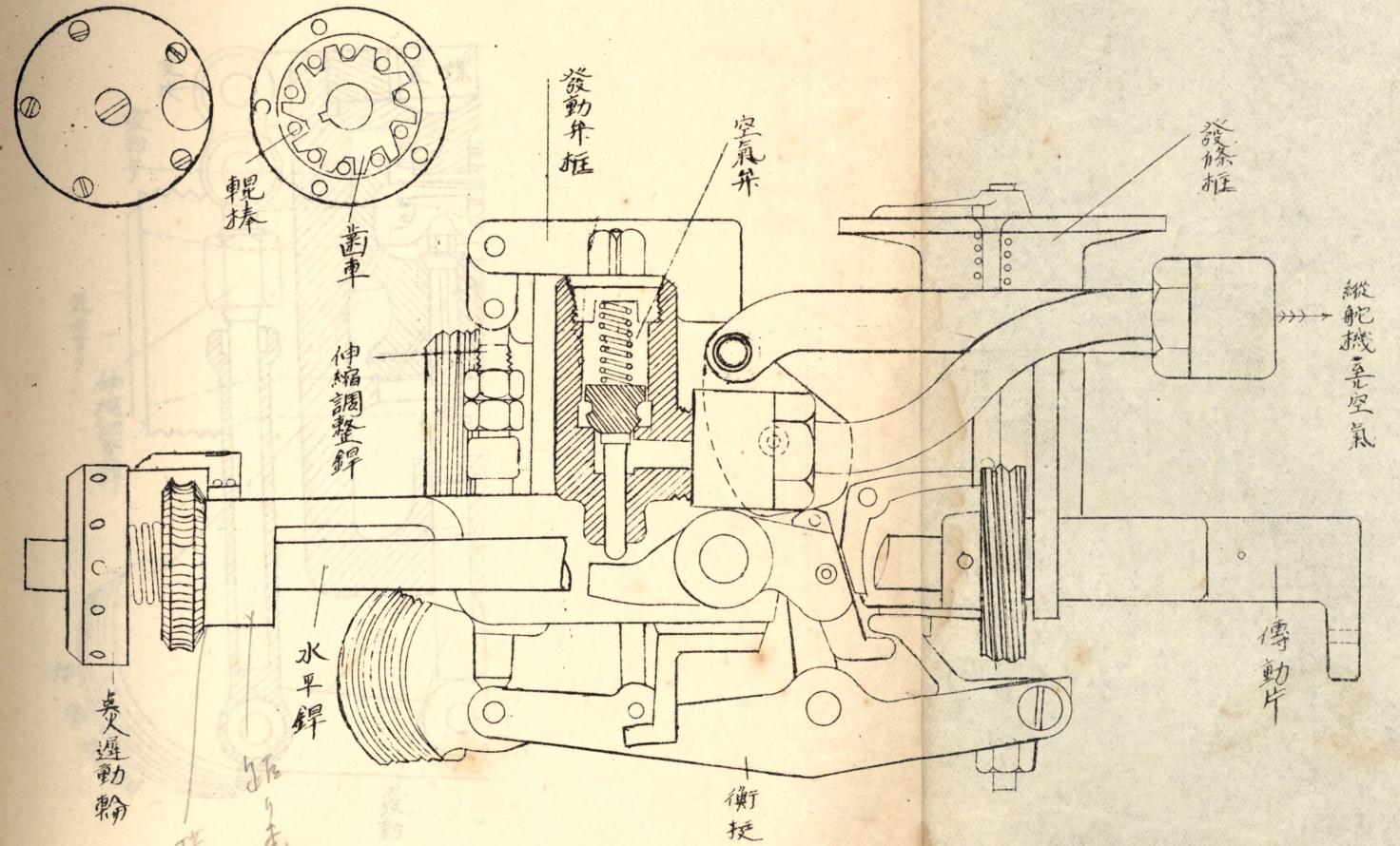
第八圖 發停裝置
