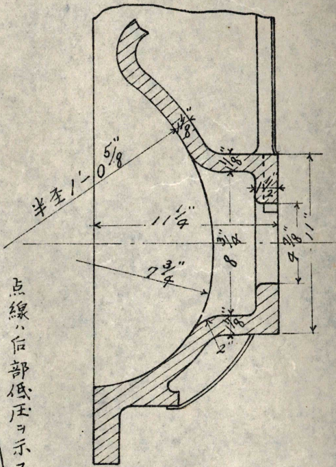
EF 切断
