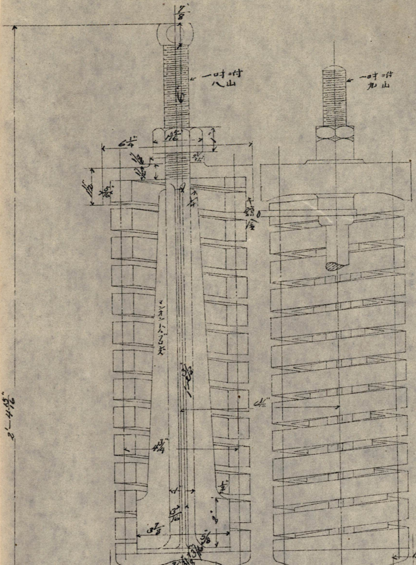
C.D切斷面
