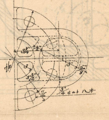
AB切斷面
