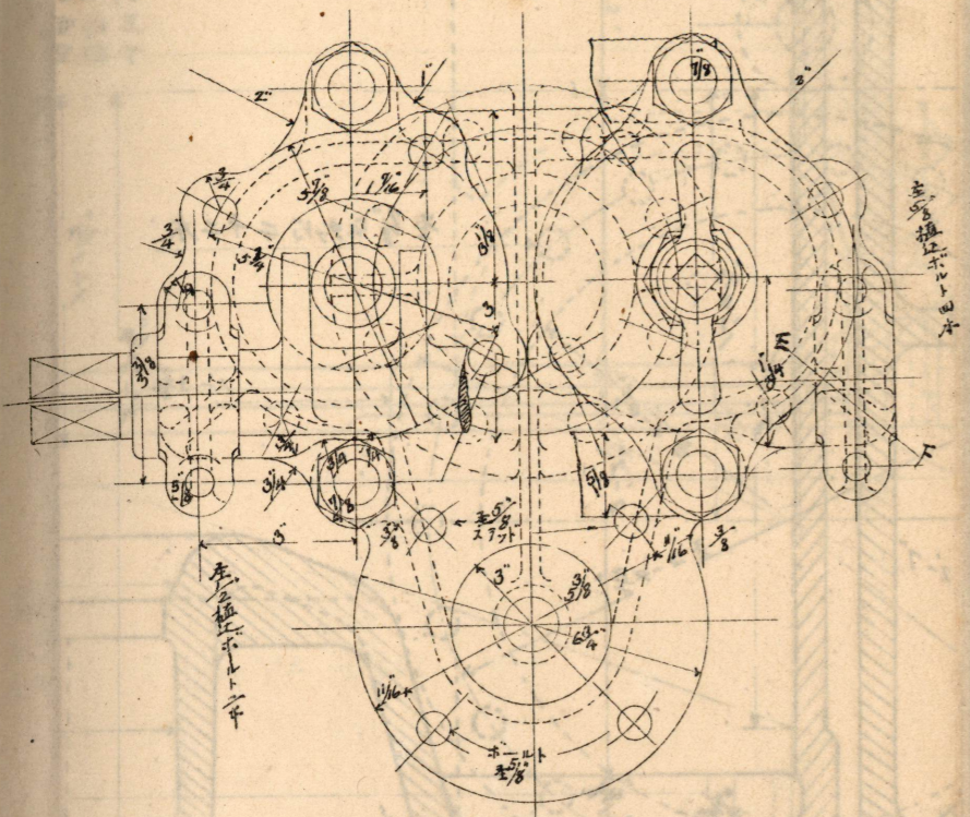
AB切斷面
