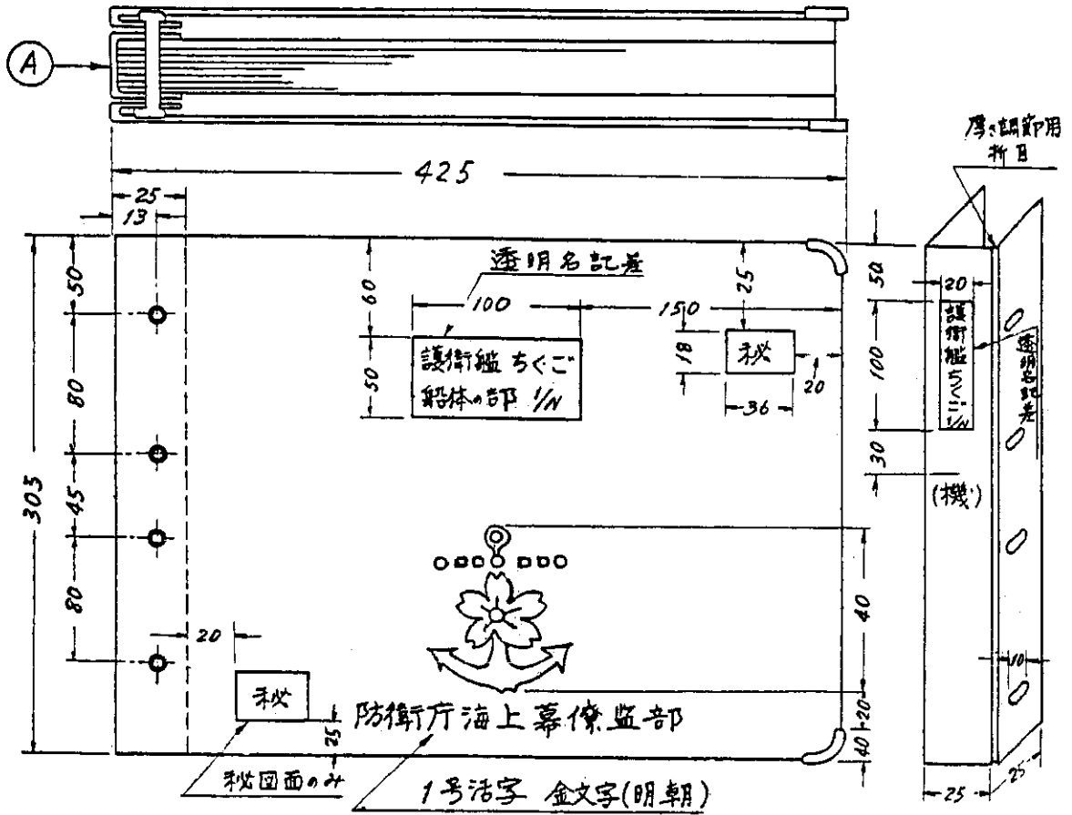
図1 製本表紙の要領
