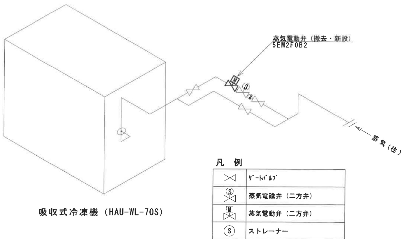
幹部学生隊舎配管等角図 S=NO SCALE
