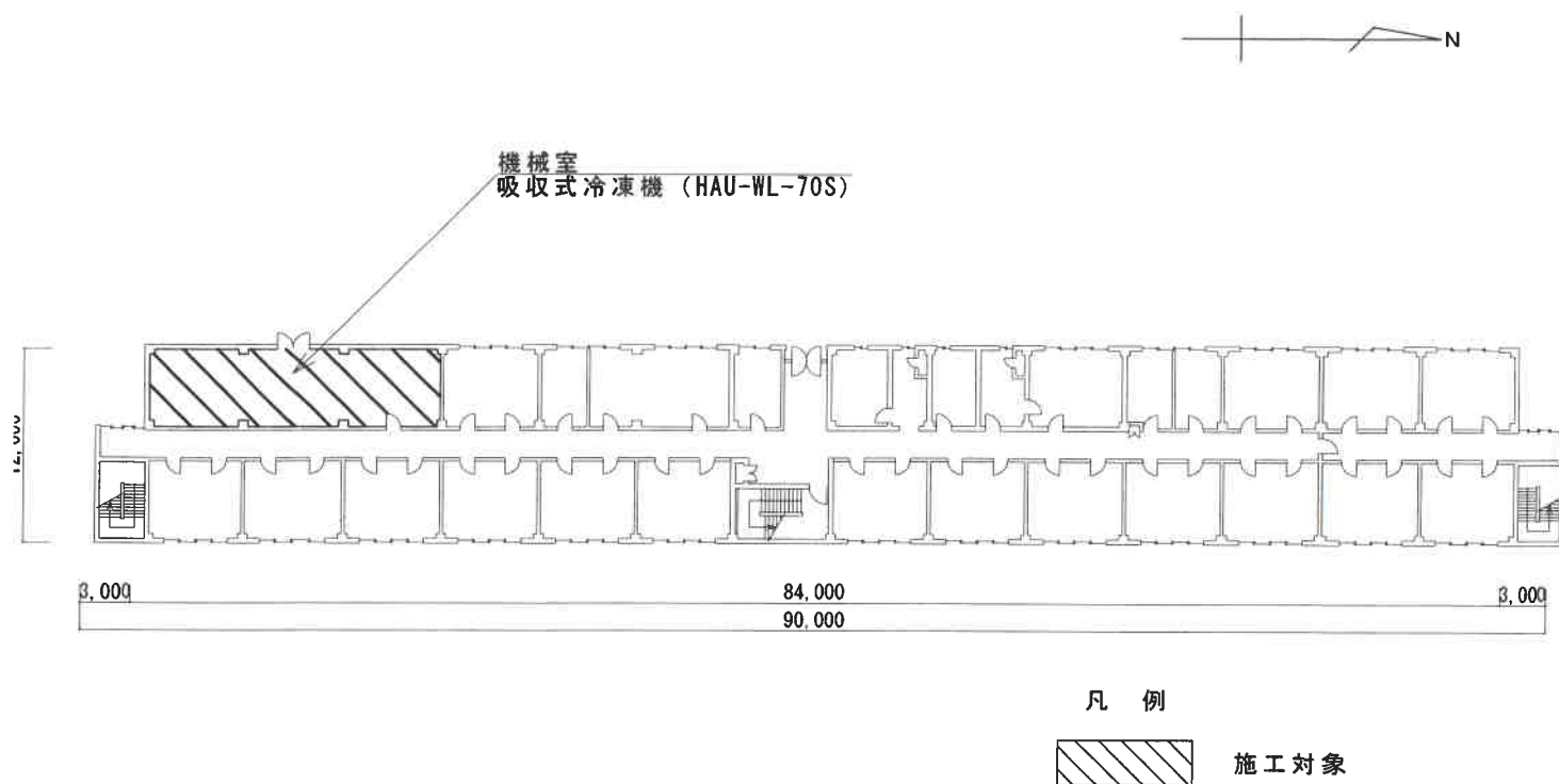
幹部学生隊舎1F平面図 S=NO SCALE
