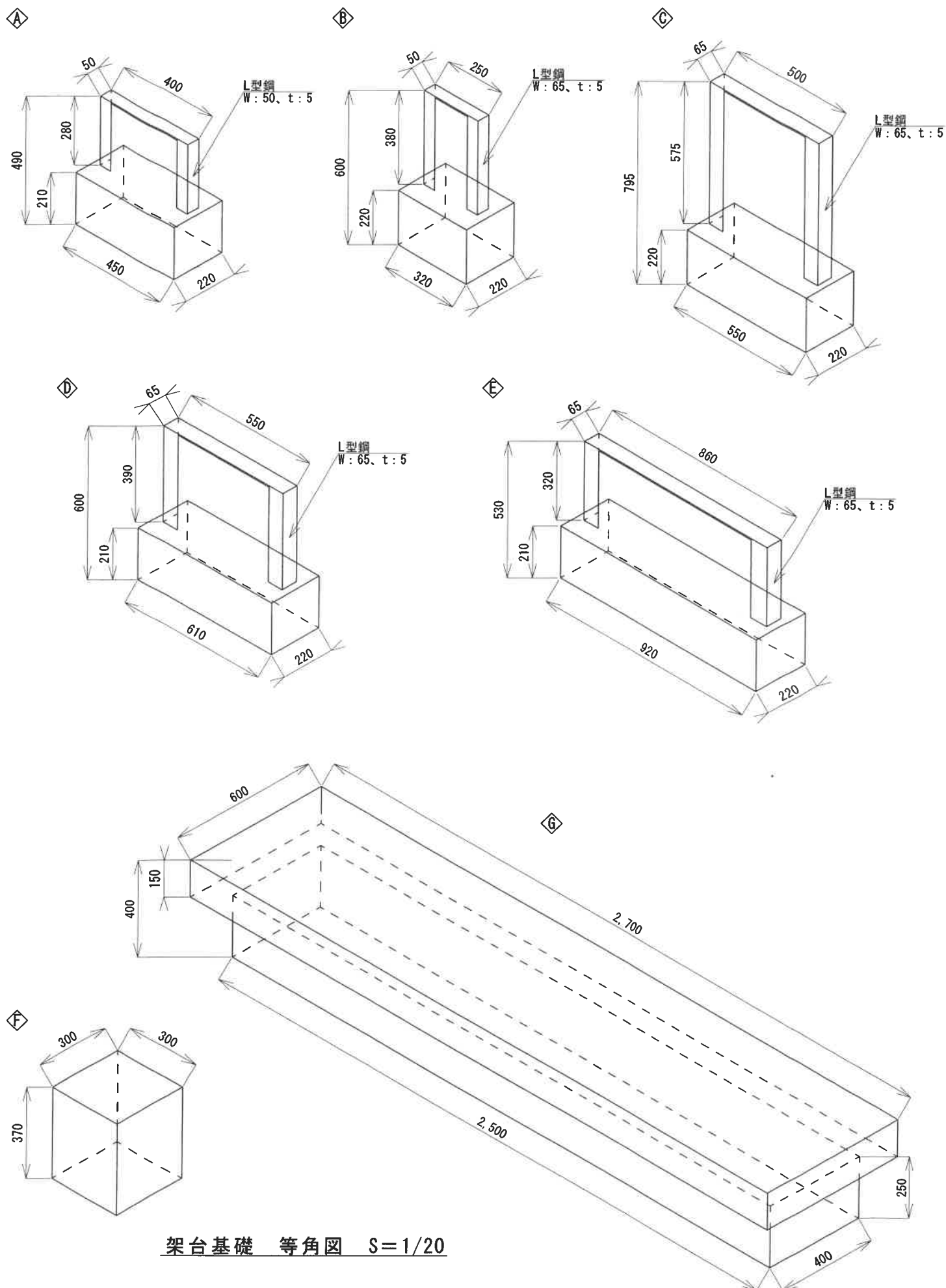
付図6—架台基礎（幹部学生隊舎）
