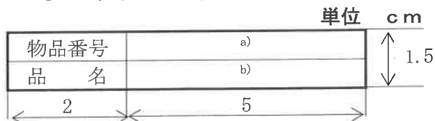
図1—銘板
