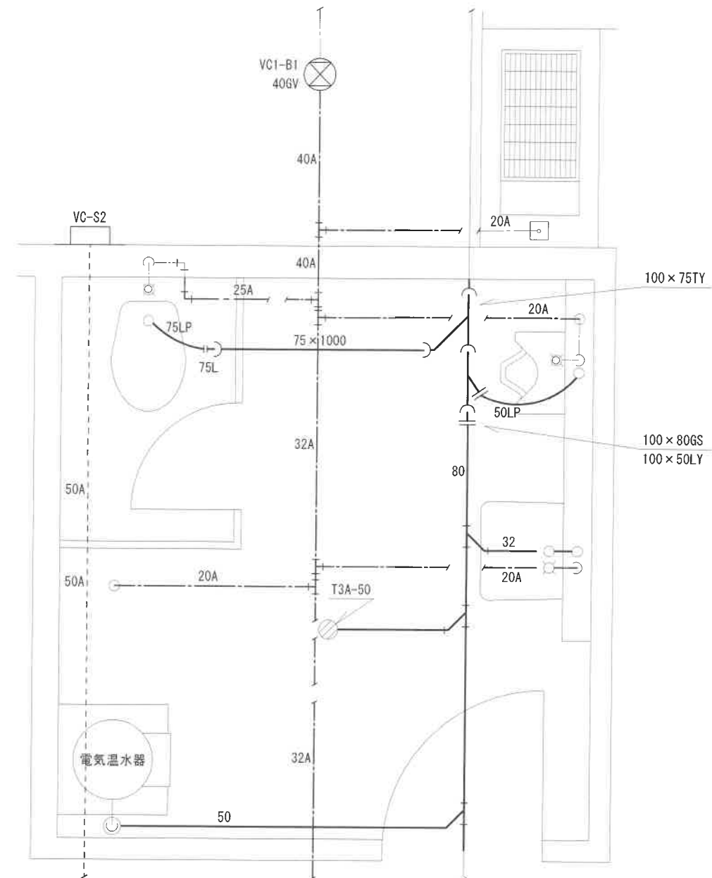
便所 給排水管 平面図 S=1/30
