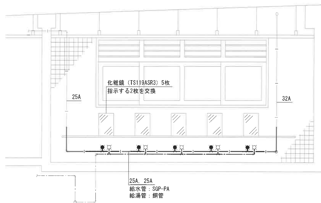
施工場所 標準立面図 S=1/50
