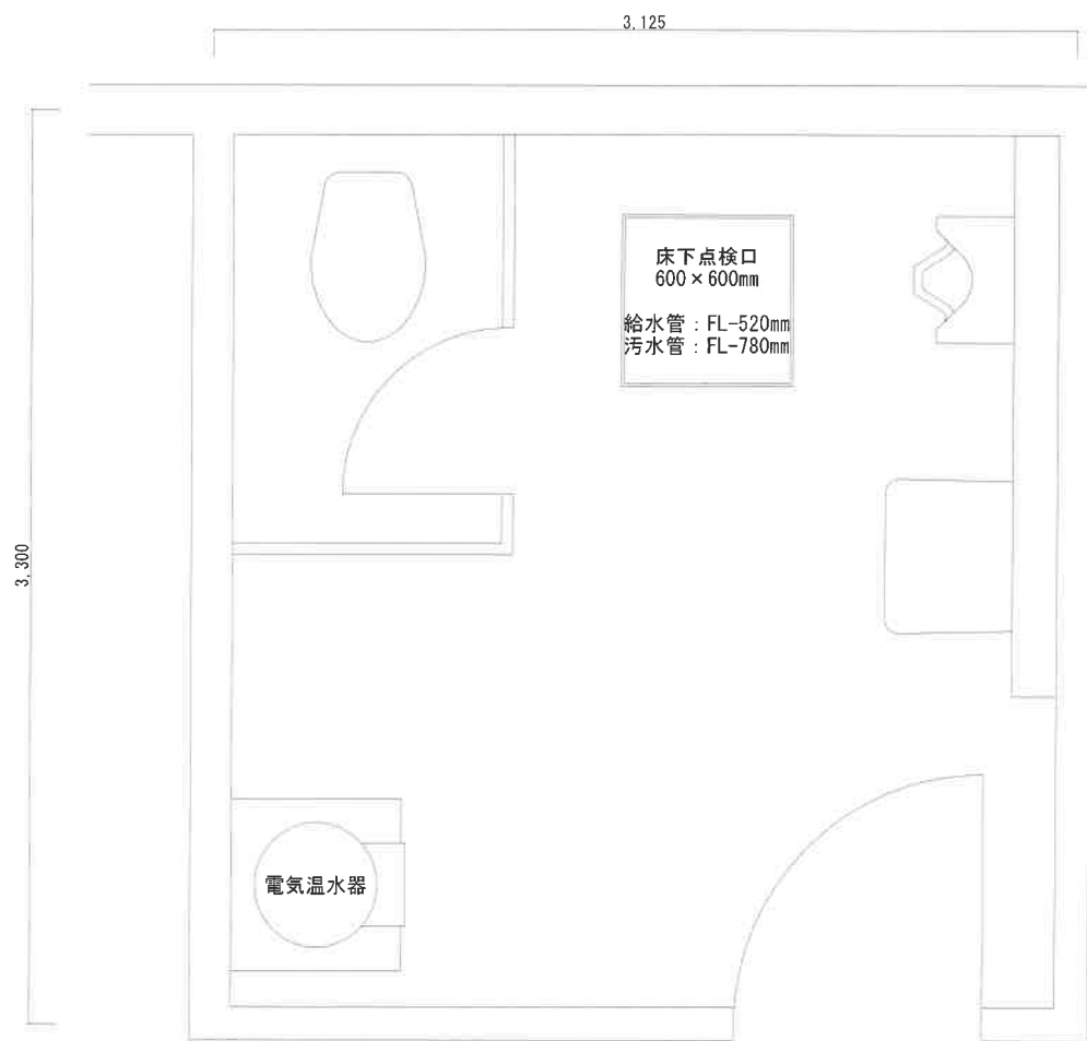
便所 平面図 S=1/30
