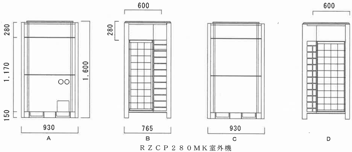
付図 2 - 履行場所等 (室外機配置図)
