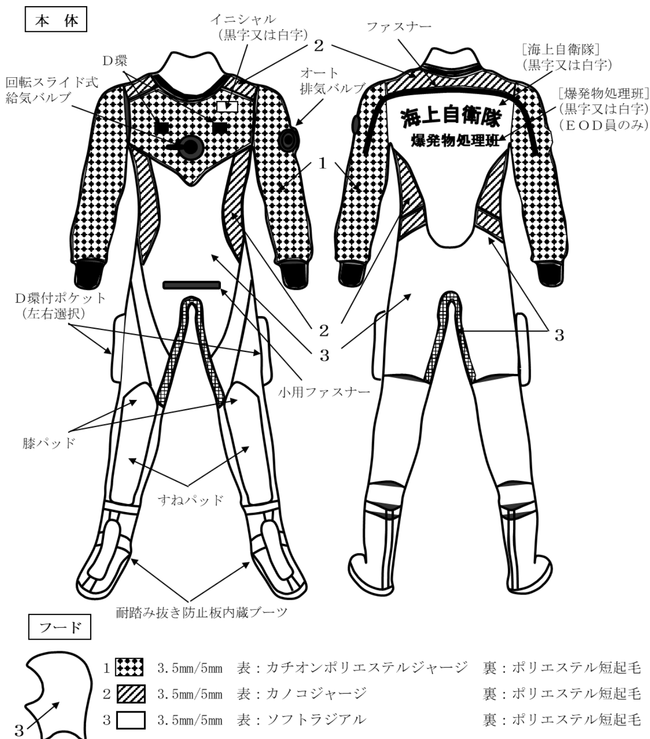
付図4 ドライスーツ, EOD用
