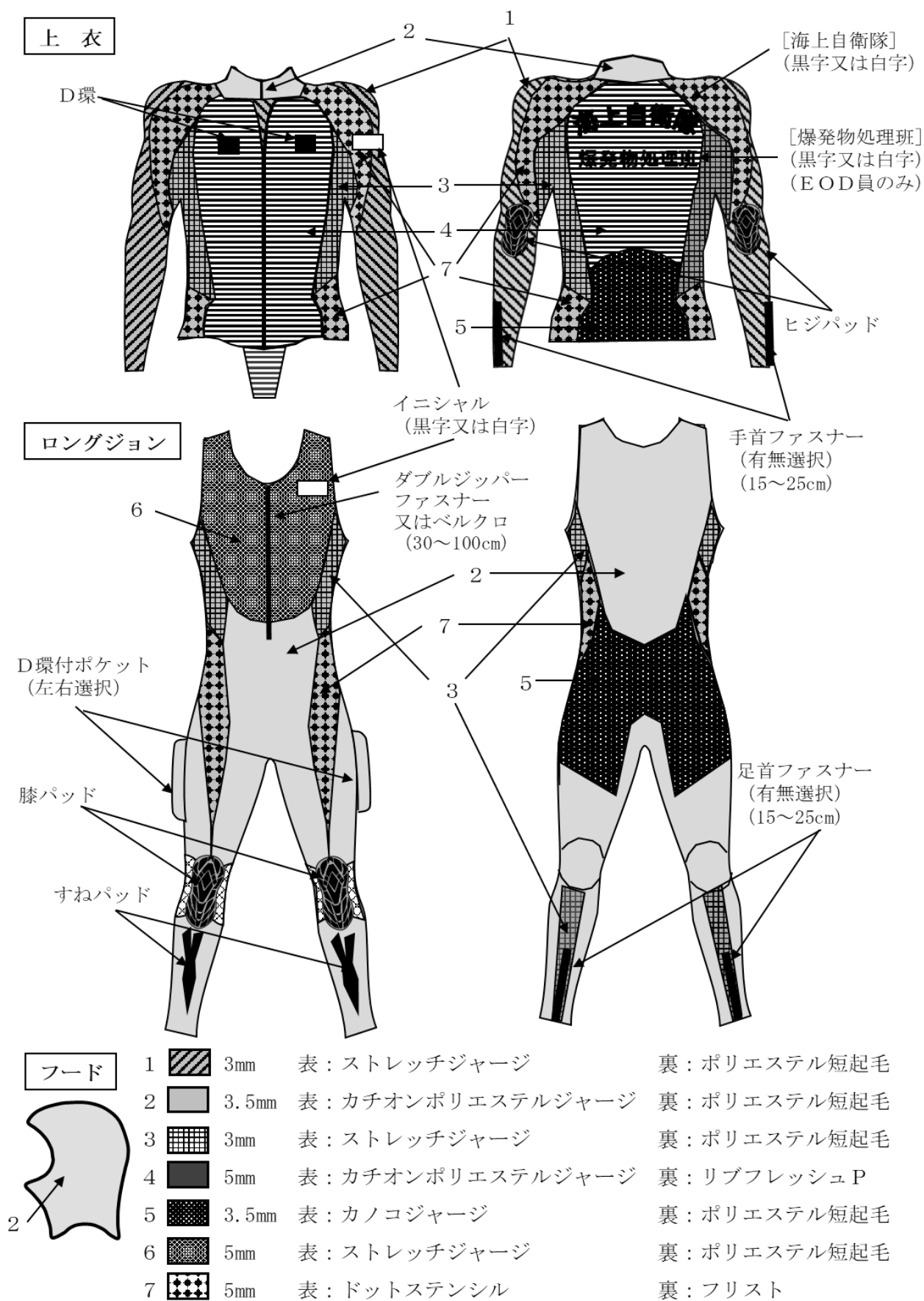
付図3ーウェットスーツ, EOD用, 5mm
