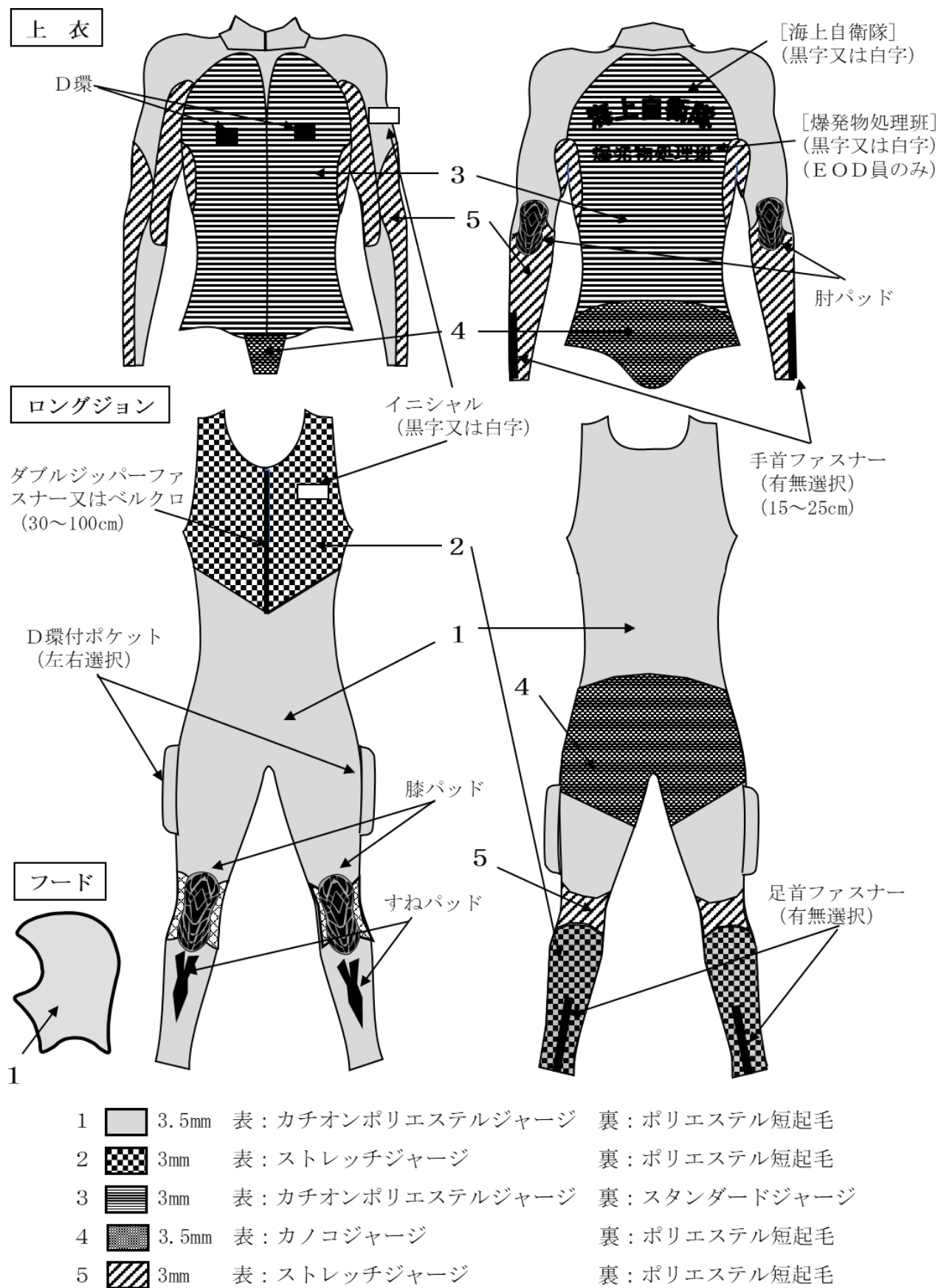
付図2ーウェットスーツ, EOD用, 3mm, セパレート
