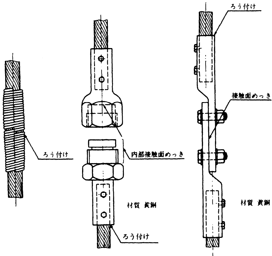
試験端子の一例
