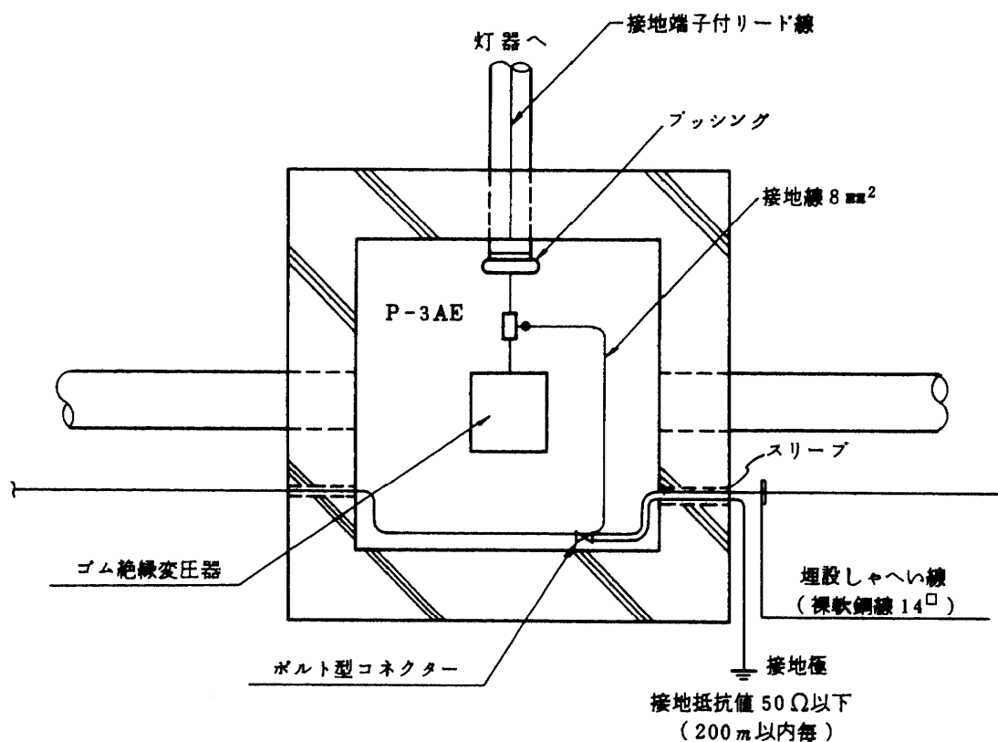
しやへい線設置要領図(2) (ハンドホール内の場合)
