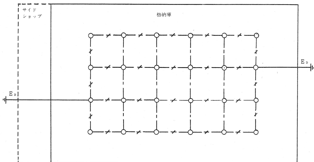
接地端子函参考図
