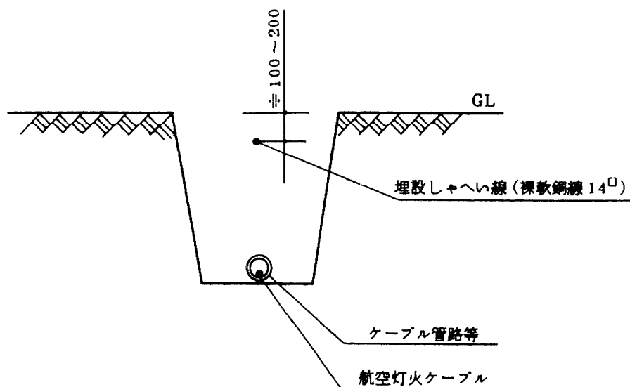
しやへい線設置要領図(1) (ケーブル管路の場合)
