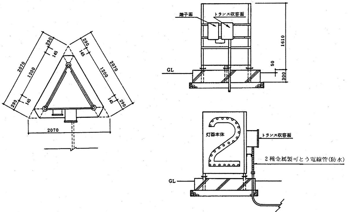
図 2 - 2 2 滑走路距離灯の灯器基礎 (単位 : mm)
