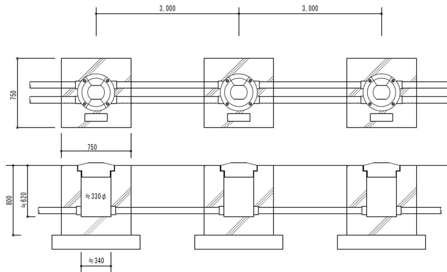
図 2 - 1 0 滑走路末端灯（埋込型）の基礎
