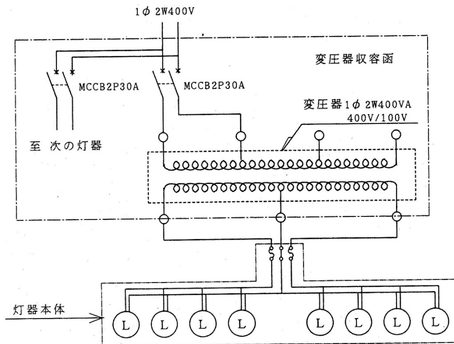
図4－13 滑走路距離灯の灯器配線
