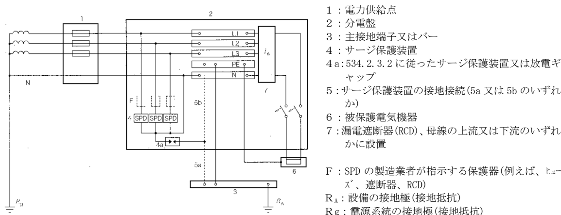
図 7-1 SPD の設置例 (JIS C 5381-12:2014 より抜粋)
