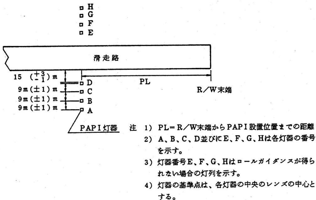
図2-31 PAPI方式の灯器配置
