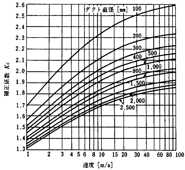
図 6 - 1 ( a ) 絶対粗さ ( \varepsilon=3.0\text{mm} ) に対する補正係数*
