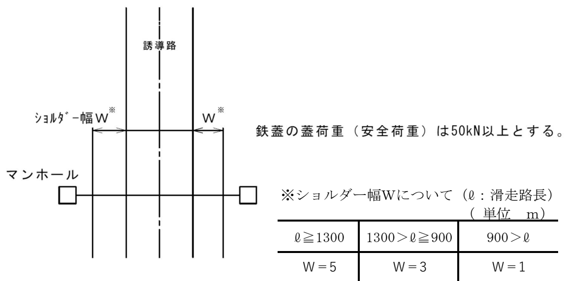
図 4 - 2 誘導路下横断管路等設置位置
