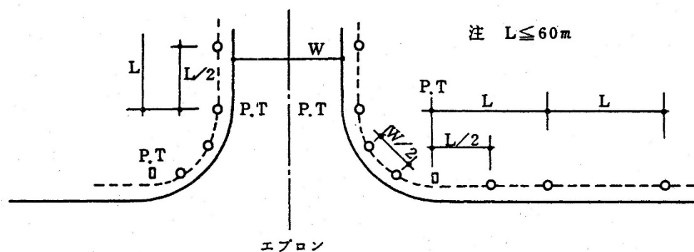
図 2-25 誘導路灯の配置 (3) (エプロンと交差する場合)
