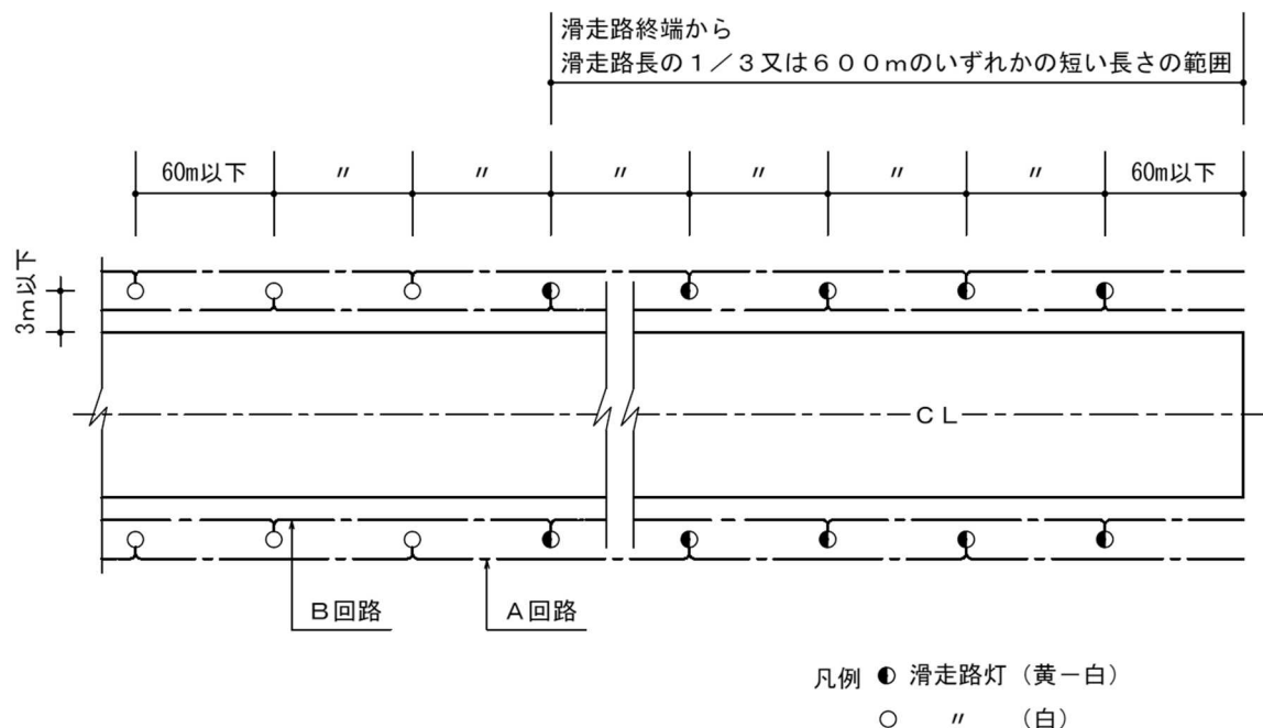
図 2-1 滑走路灯の配置
