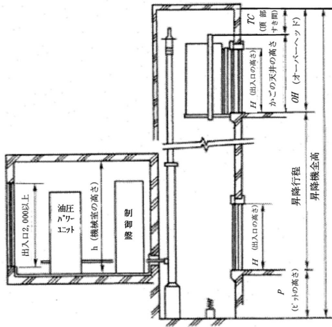
図 1 - 2 間接式油圧エレベーターの昇降路（参考）
