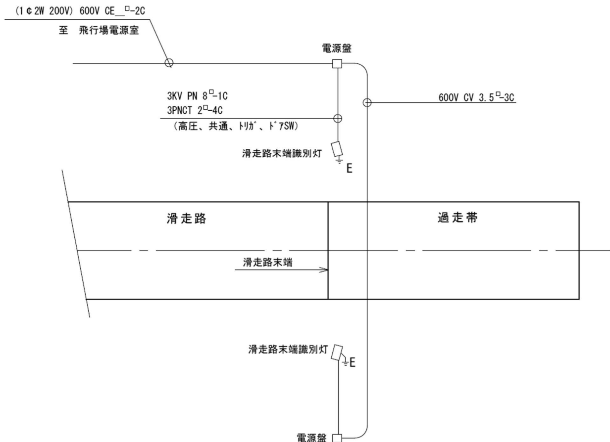
図 4-28 滑走路末端識別灯配線図
