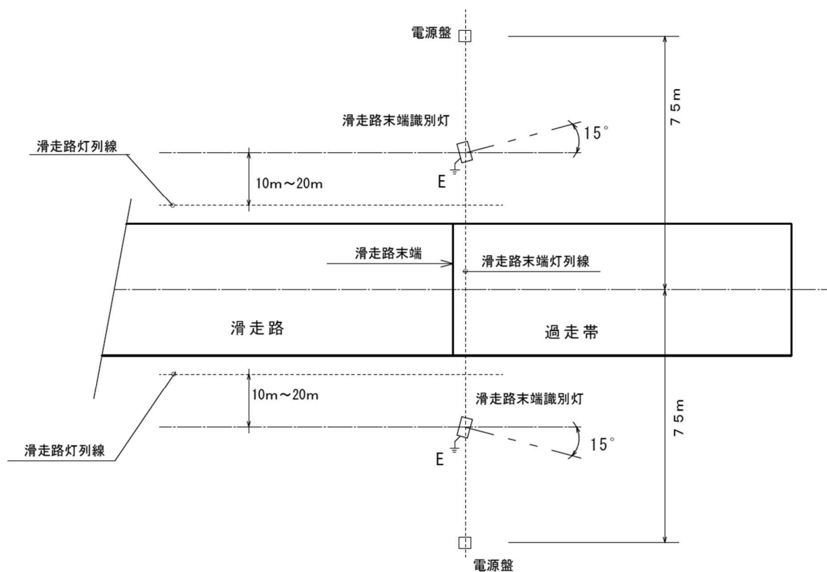
図 2 - 7 1 標準配置 (滑走路末端識別灯)
