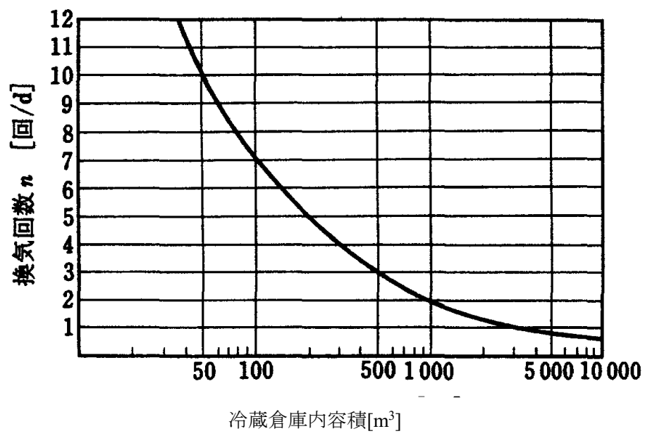
図 7 - 1 冷蔵庫換気回数 (n 回/24 時間)
