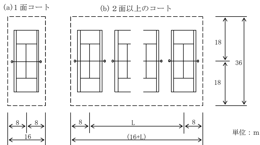
図9-2 テニスコートの照明範囲
