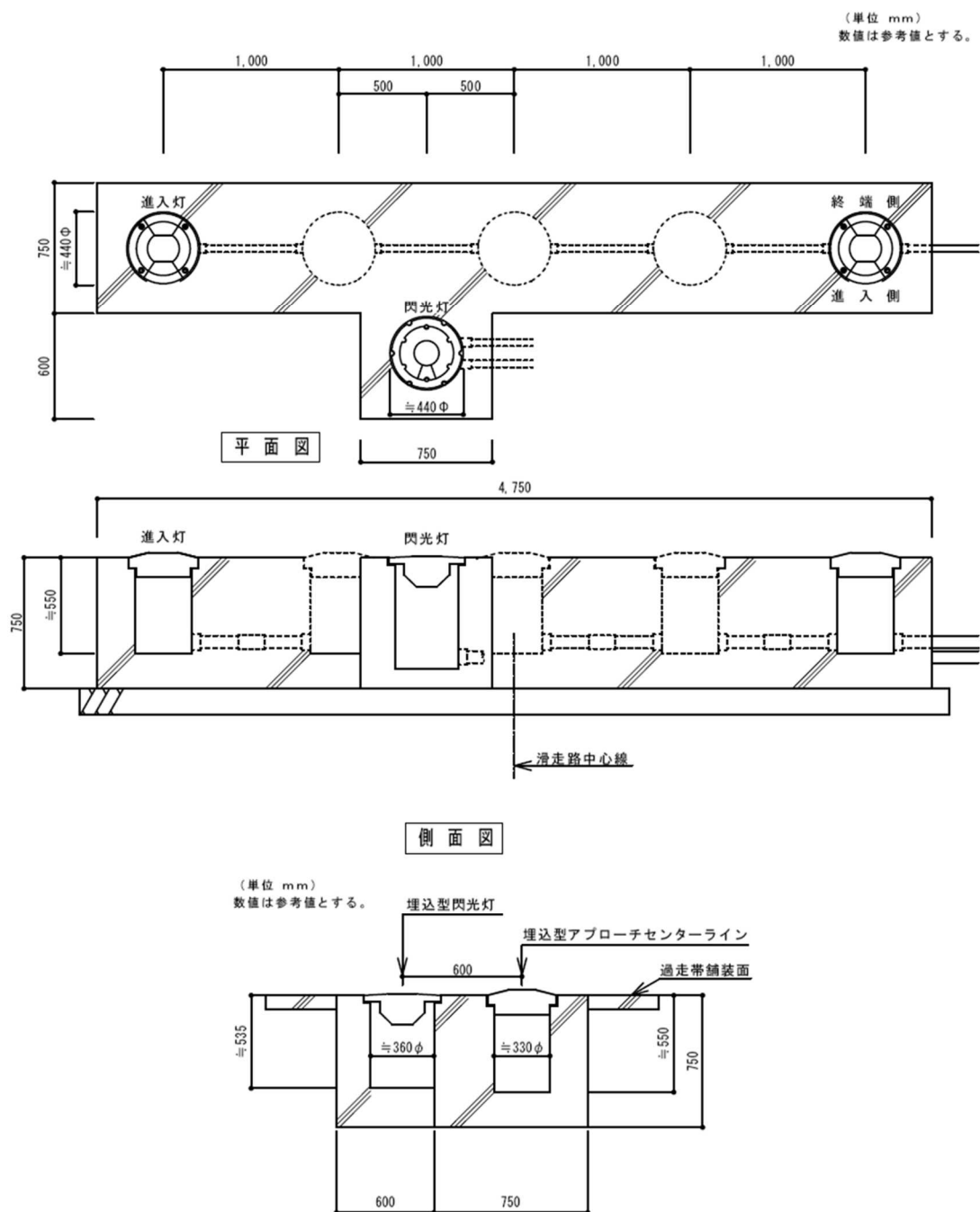
図 2-67 埋込型アプローチセンターライン及び連鎖式閃光灯の灯器基礎
