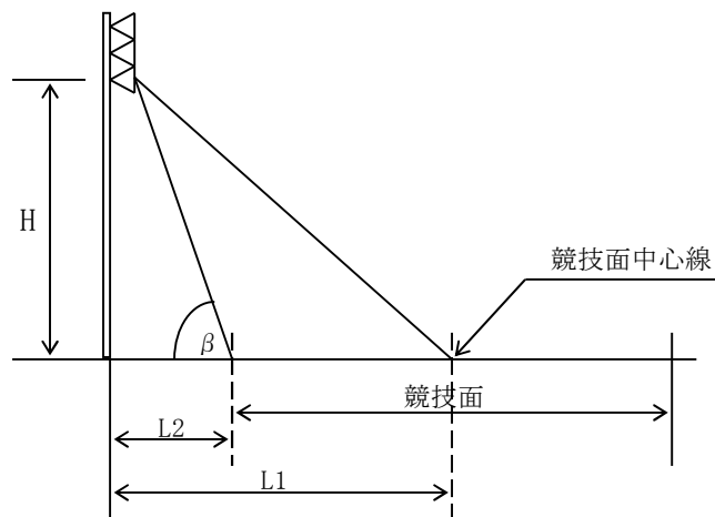
図 9－10 照明器具の取り付け高さ
