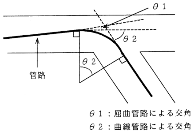
図5.2 交角算出図
