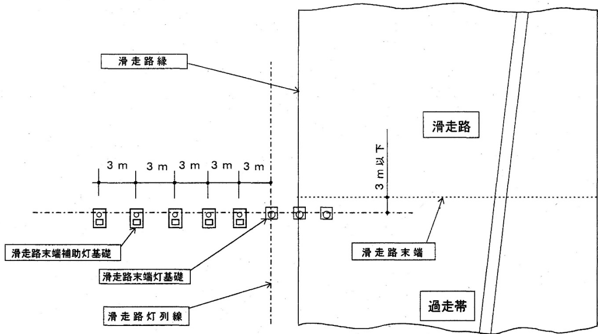
図2-13 滑走路末端補助灯（露出型）基礎の配置
