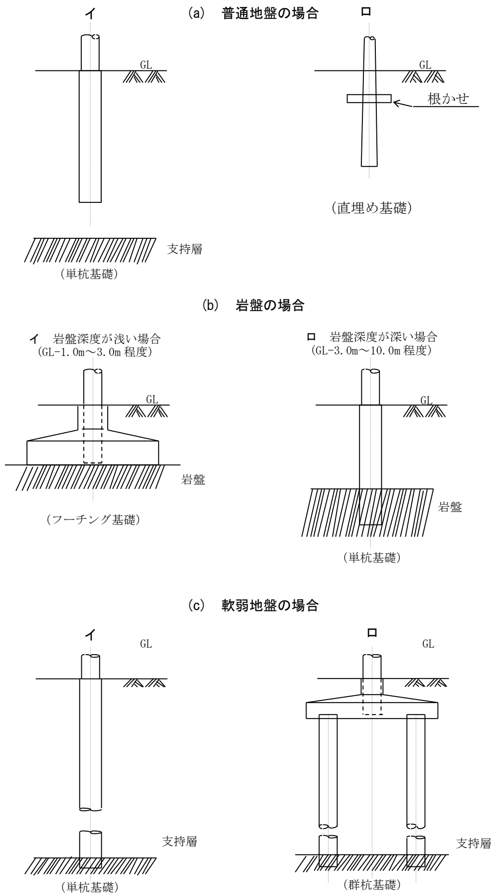
図9-14 基礎形式例
