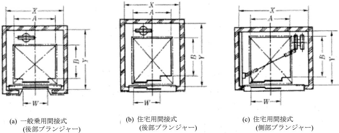
図 1 - 1 間接式油圧エレベーターの昇降路平面図
