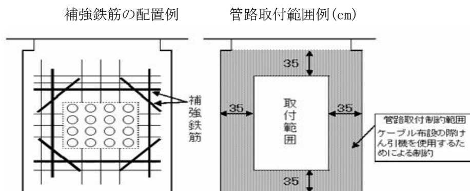
図4.2 開口部補強例及び取付範囲例
