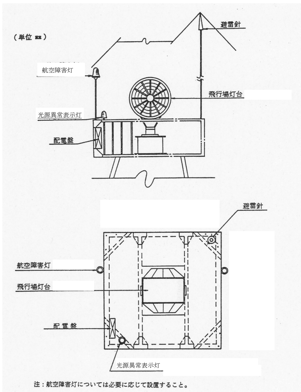
図 2 - 7 7 飛行場灯台の設置台（参考）
