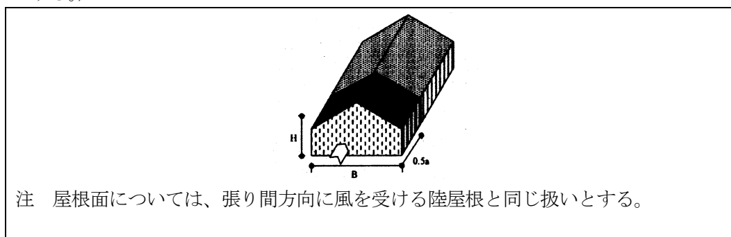
図二 閉鎖型の建築物（けた行方向に風を受ける場合。表一、表二及び表五を用いるものとする。）
