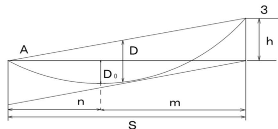
図10.2 電線支持点に高低差のある場合の径間とち度
