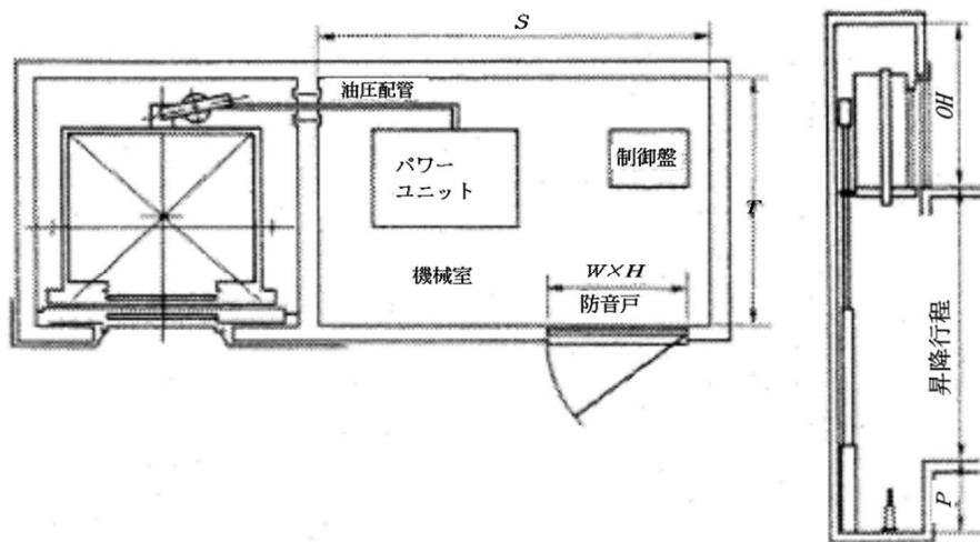
図 1 - 3 間接式油圧エレベーターの機械室平面図（参考）
