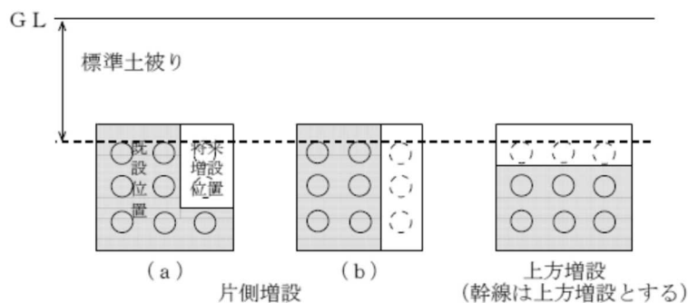
図2.5 管路の増設位置
