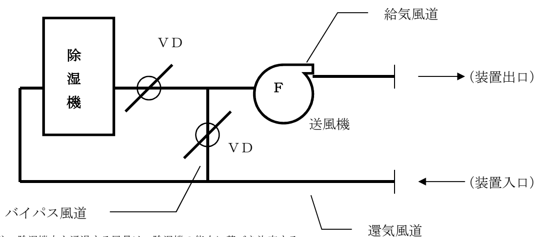
図 8 - 1 除湿機廻り風道要領図
