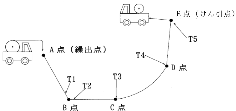
図5.1 光ファイバケーブル ルート図 (例)
