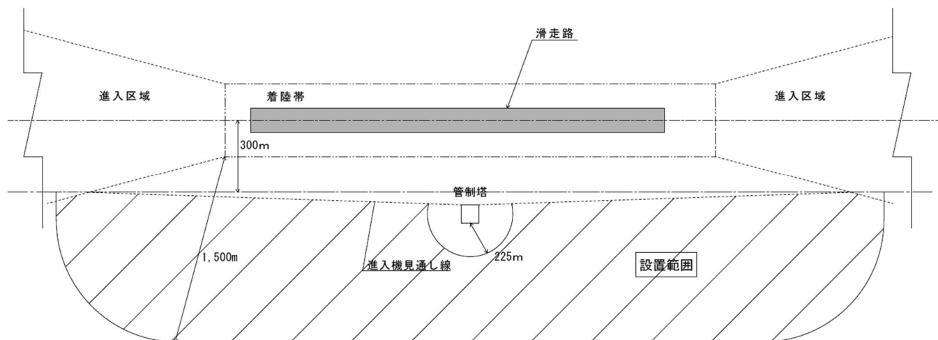
図 2-76 飛行場灯台設置範囲
