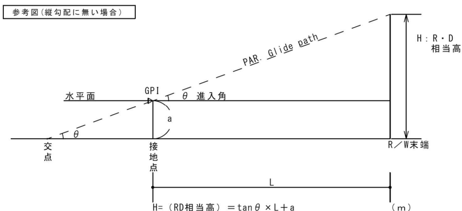
図 2-35 着陸援助施設が GCA の場合
