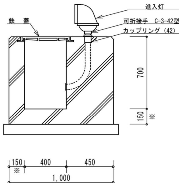
図 2 - 6 2 露出型灯器基礎 (進入灯)
