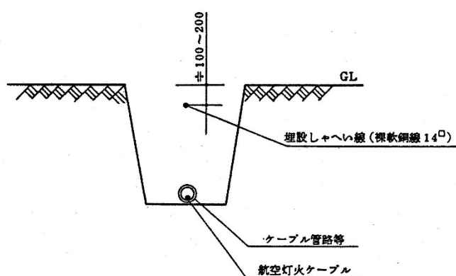
図4-33 シャヘい線設置要領図(1)(ケーブル管路の場合)
