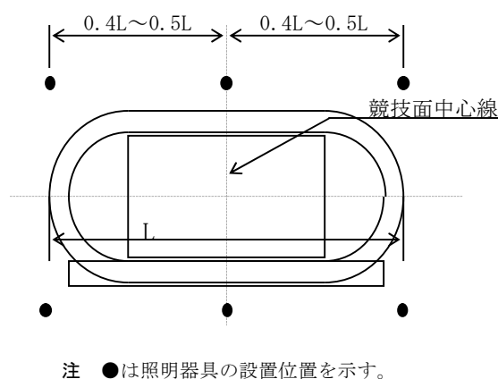
図9-9 陸上競技場及び複合競技施設（陸上競技場・サッカー場・ラグビー場）の照明器具の配置（6か所配置の場合）
