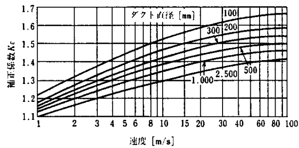
図 6 - 1 ( b ) 絶対粗さ ( \varepsilon=0.9\text{mm} ) に対する補正係数*
