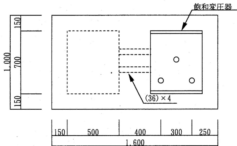
図 4 - 1 0 飽和変圧器基礎
