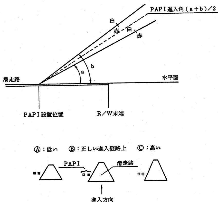
図2-48 APAPI方式の灯火信号情報
