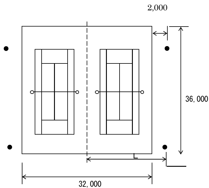
図-9 テニスコート平面図
