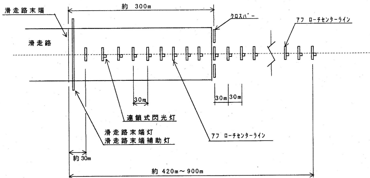
図2-51 進入灯配置図（標準式）
