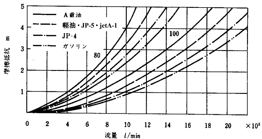
図 3-5 ローディングアームの摩擦抵抗
