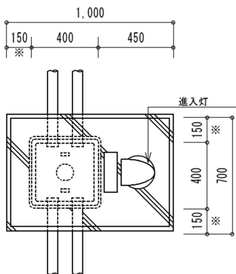
図 2 - 6 2 露出型灯器基礎 (進入灯)
