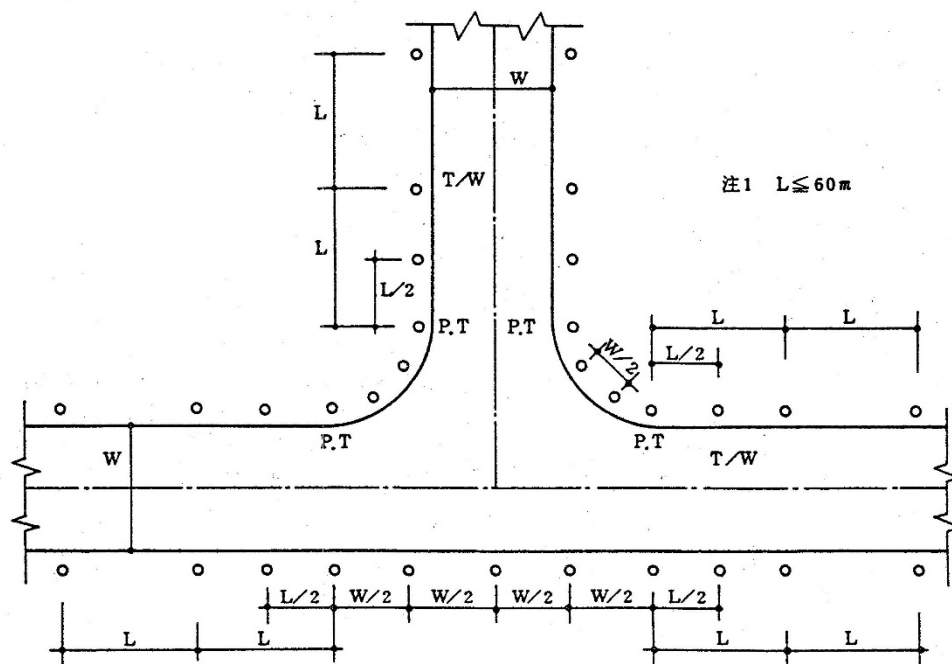
図 2-24 誘導路灯の配置 (2) (他の誘導路と交差する場合)
