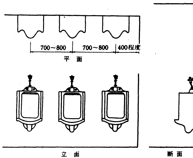
2 小便器
