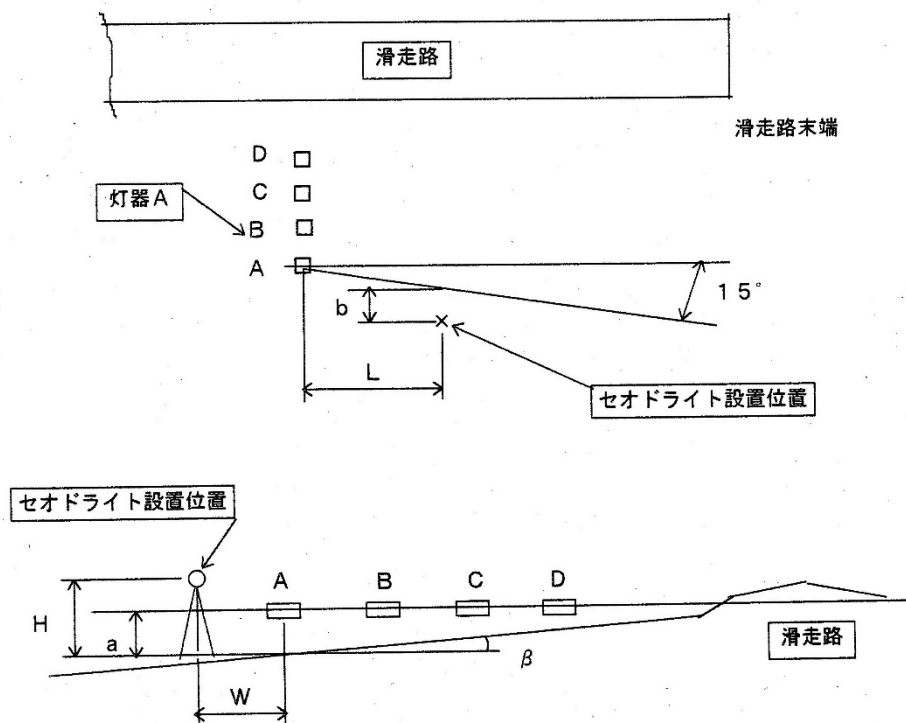
図 2-4-1 セオドライト設置位置
