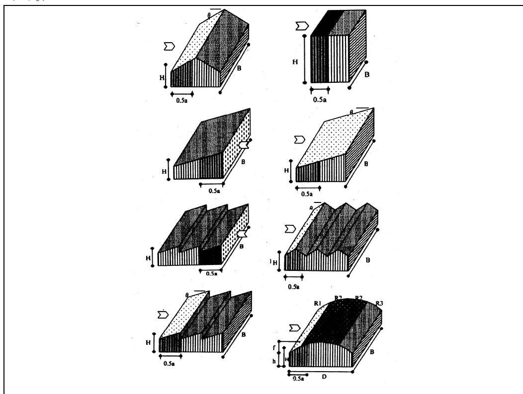
図一 閉鎖型の建築物（張り間方向に風を受ける場合。表一から表五までを用いるものとする。）
