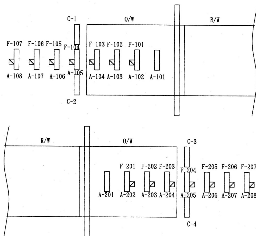
図 2-58 灯器番号例
