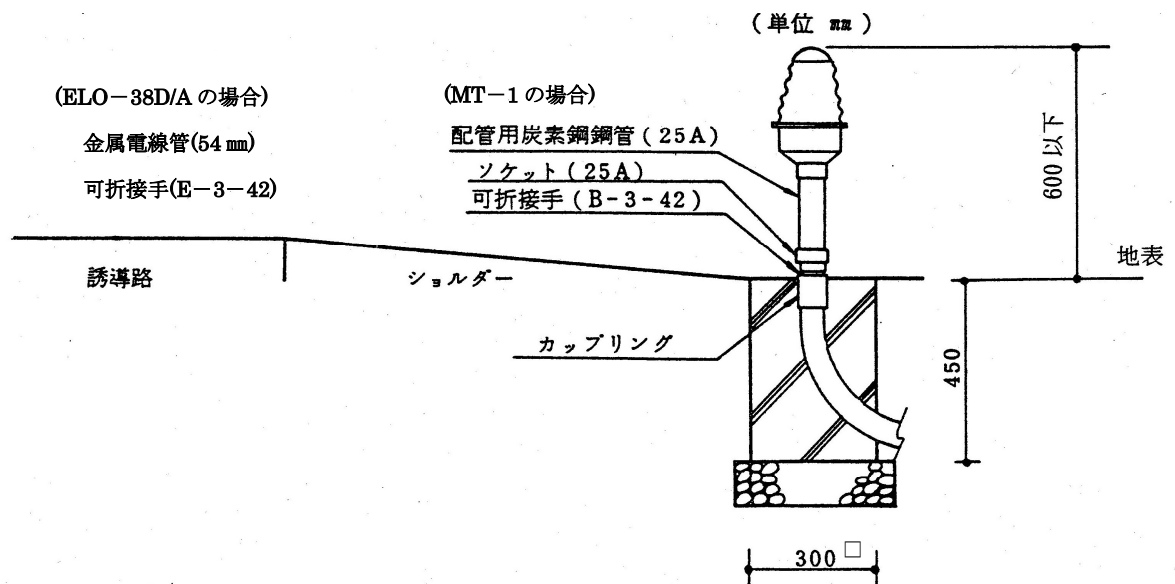
図 2 - 2 9 積雪地の場合の灯器基礎
