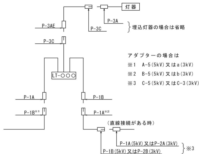
図 4-6 滑走路灯の配線接続要領
