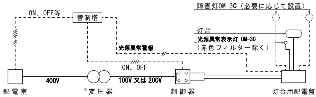
図 4-3 2 飛行場灯台の配線系統
