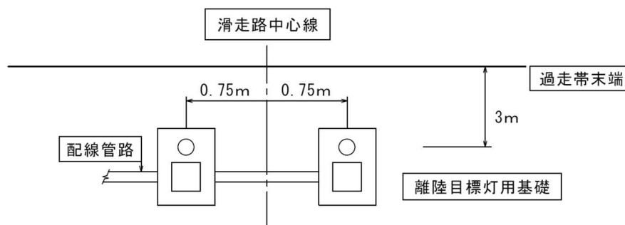
図2-19 離陸目標灯の基礎の配置
