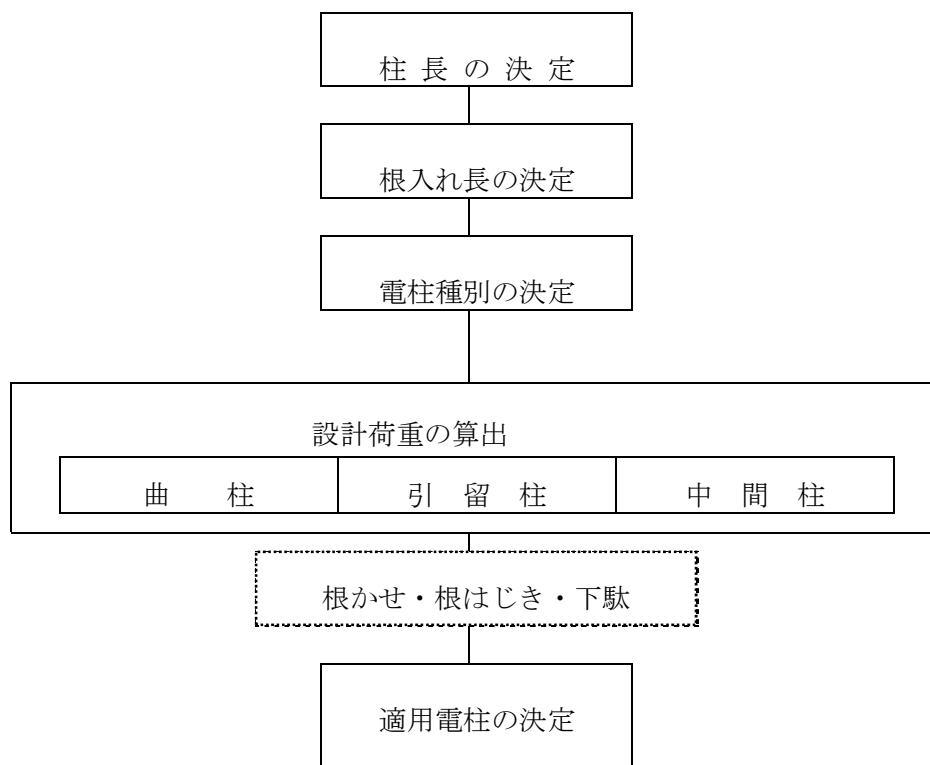
図3.2 電柱設計の流れ
