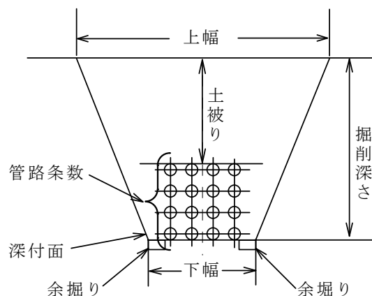
図2.2 掘削寸法
