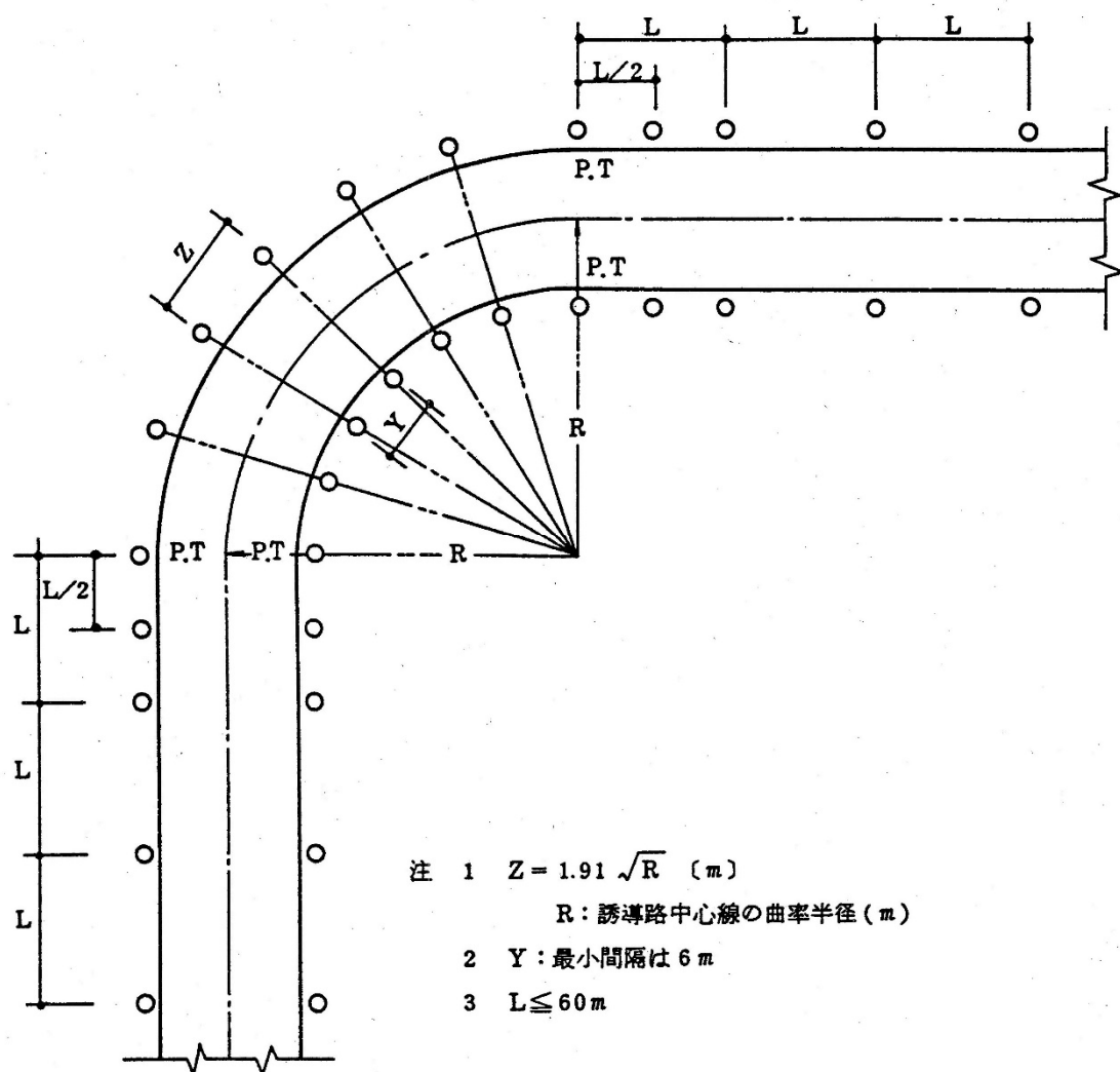
図 2-27 誘導路灯の配置 (5) (単独曲線誘導路の場合)
