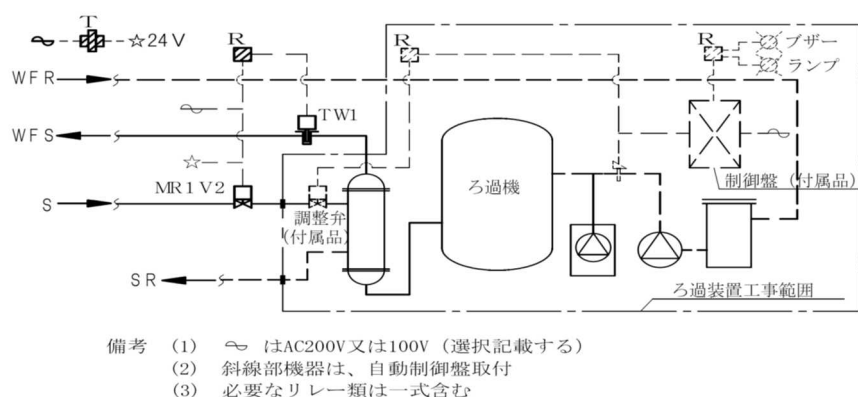
図3-1 循環ろ過装置系システム図
