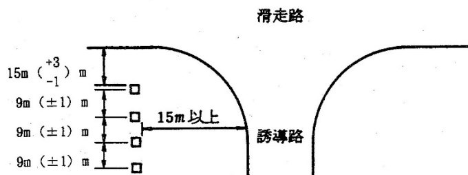
図2-32 滑走路及び誘導路との間隔
