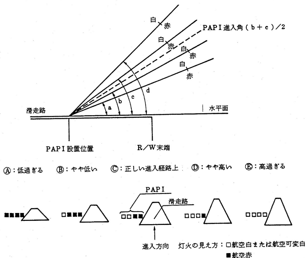
図2-30 PAPI方式の灯火信号
