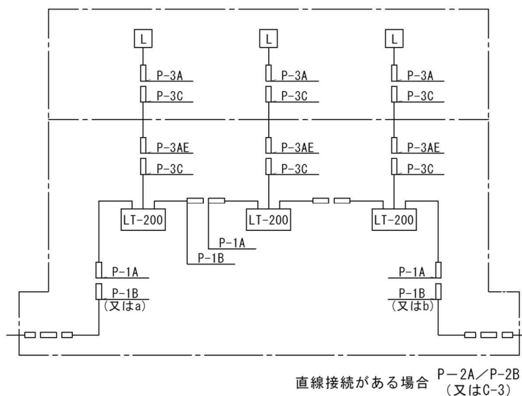
図４－１７ 進入角指示灯の配線接続要領（1台分）（電球式）
