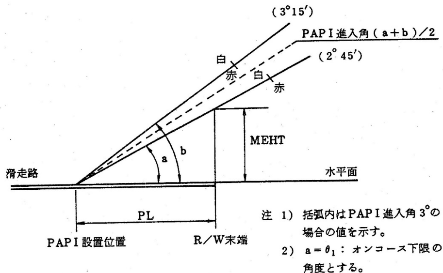
図 2-50 APAPI 方式設定仰角
