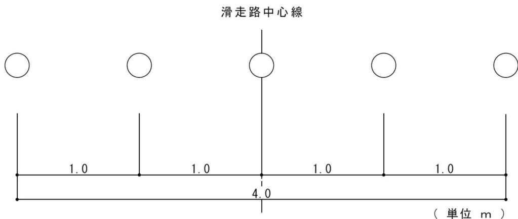
図2-55 アプローチセンターラインの灯器配置
