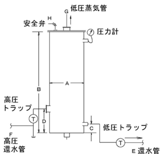
図5-2 フラッシュタンク
