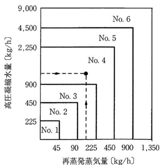
図5-3 フラッシュタンクの選定
