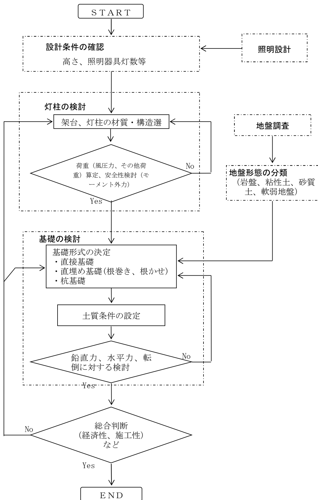
図 9 - 1 灯柱及び基礎の標準設計フロー
