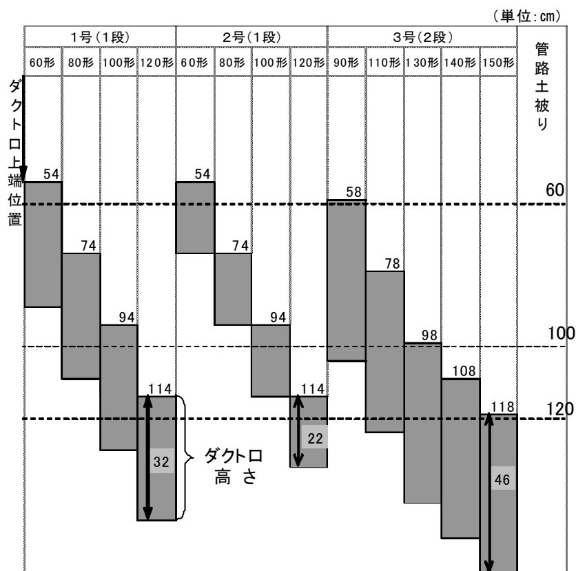
図2.8 ハンドホールダケ外口位置
