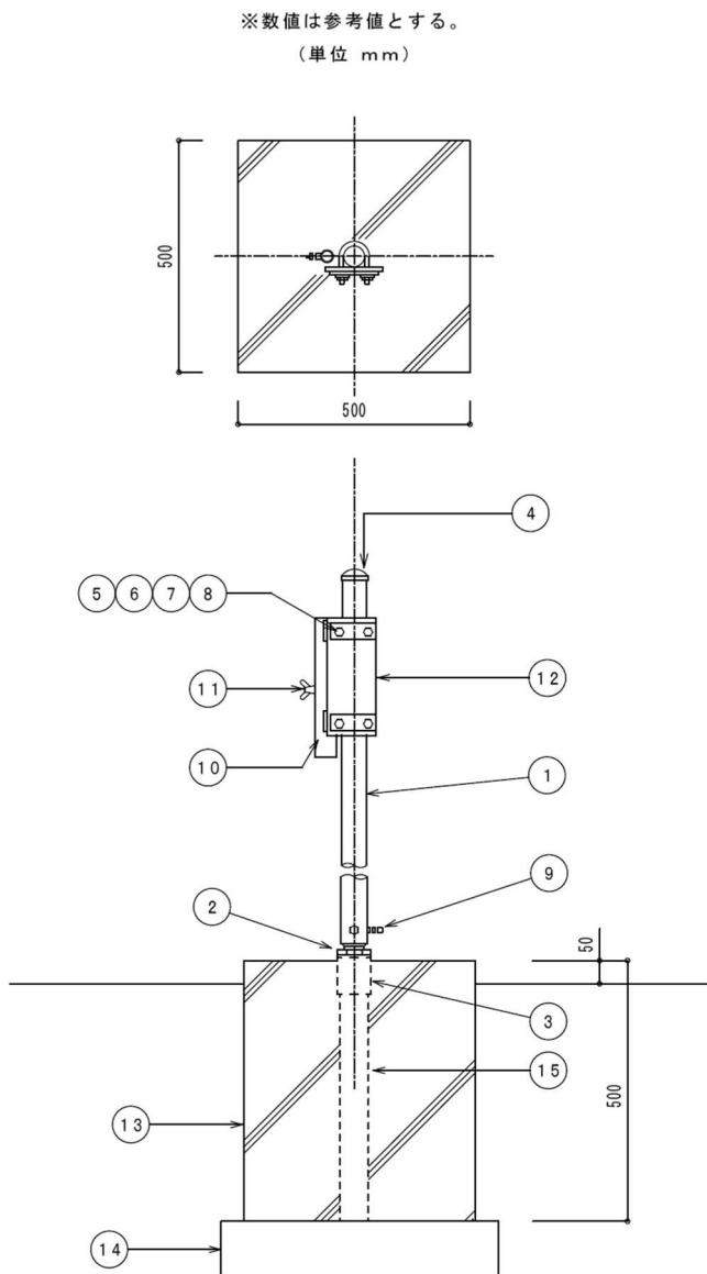
図 2－4 6 仰角点検台基礎
