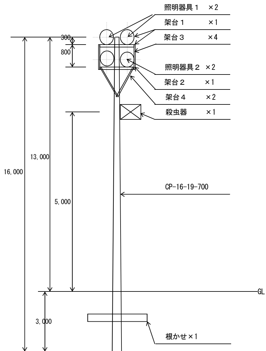
図－１２ 照明灯柱姿図
