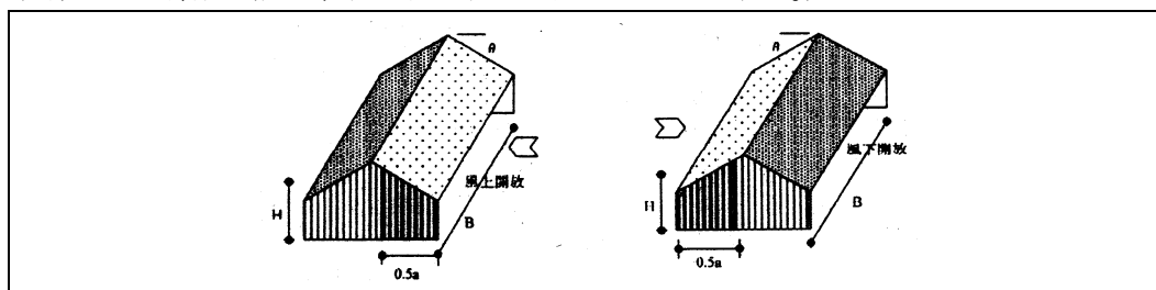
図三 開放型の建築物（表一、表三及び表五を用いるものとする。）
