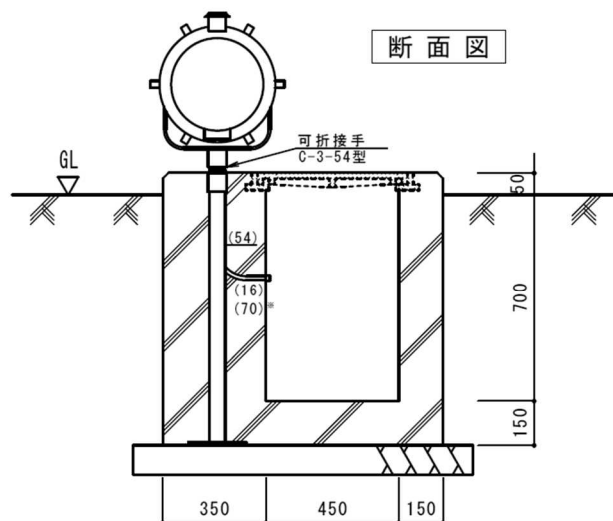
図 2 - 6 1 露出型灯器基礎 (閃光灯発光部)
