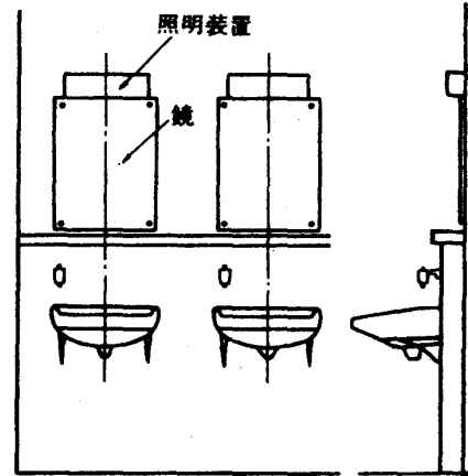
立面
