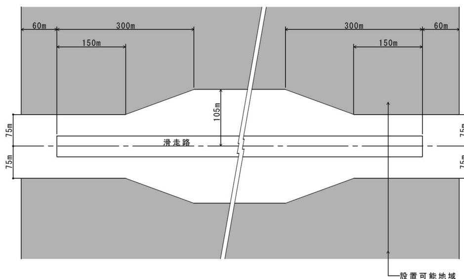
図 2 - 7 3 着陸方向指示灯及び風向灯の設置可能区域
