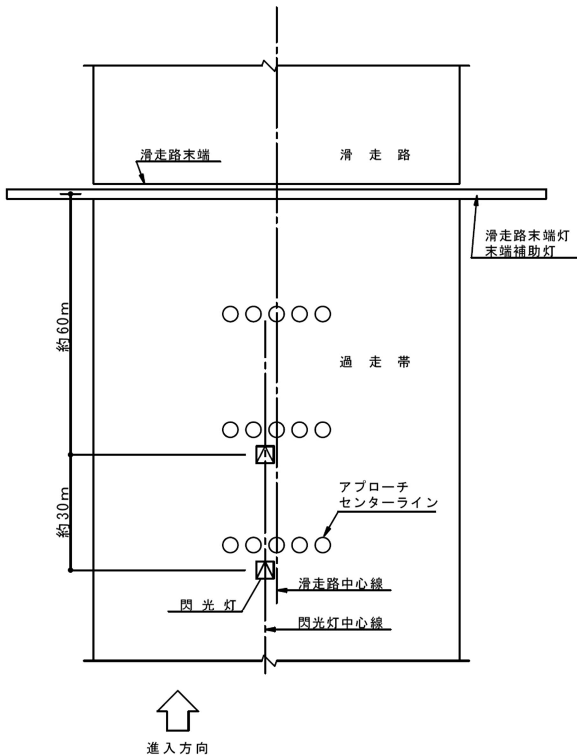
図 2 - 5 7 閃光灯の配置
