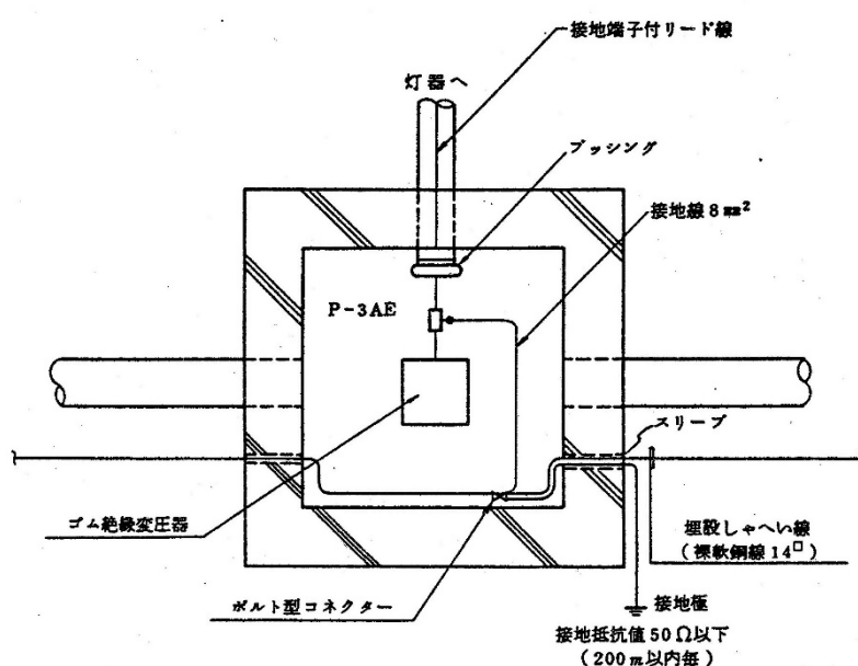
図4-34 シャヘい線設置要領図(2)(ゴム絶縁変圧器収容函内の場合)
