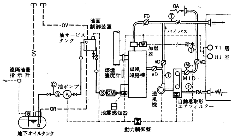
図 1-2 システム図
