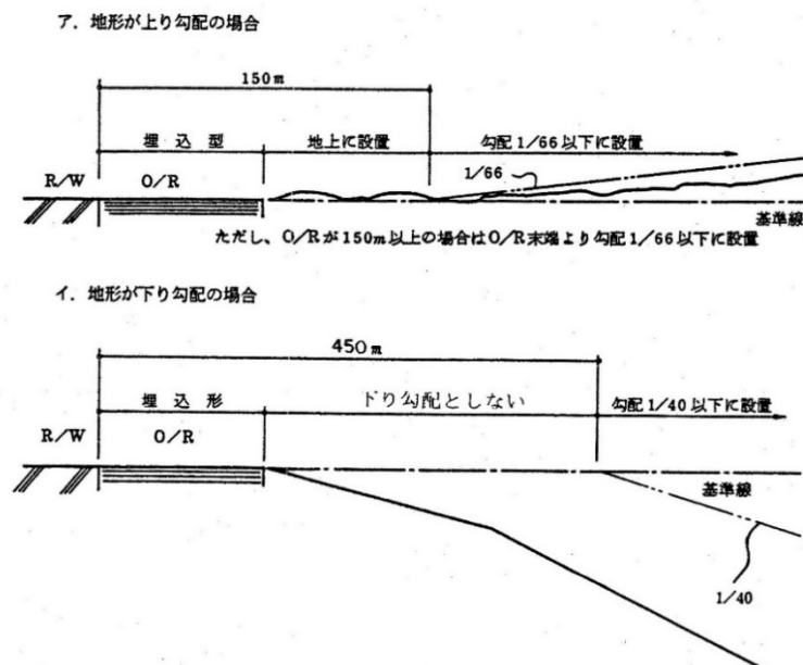
図 2-53 地形条件による設置裕度（縦断面）
