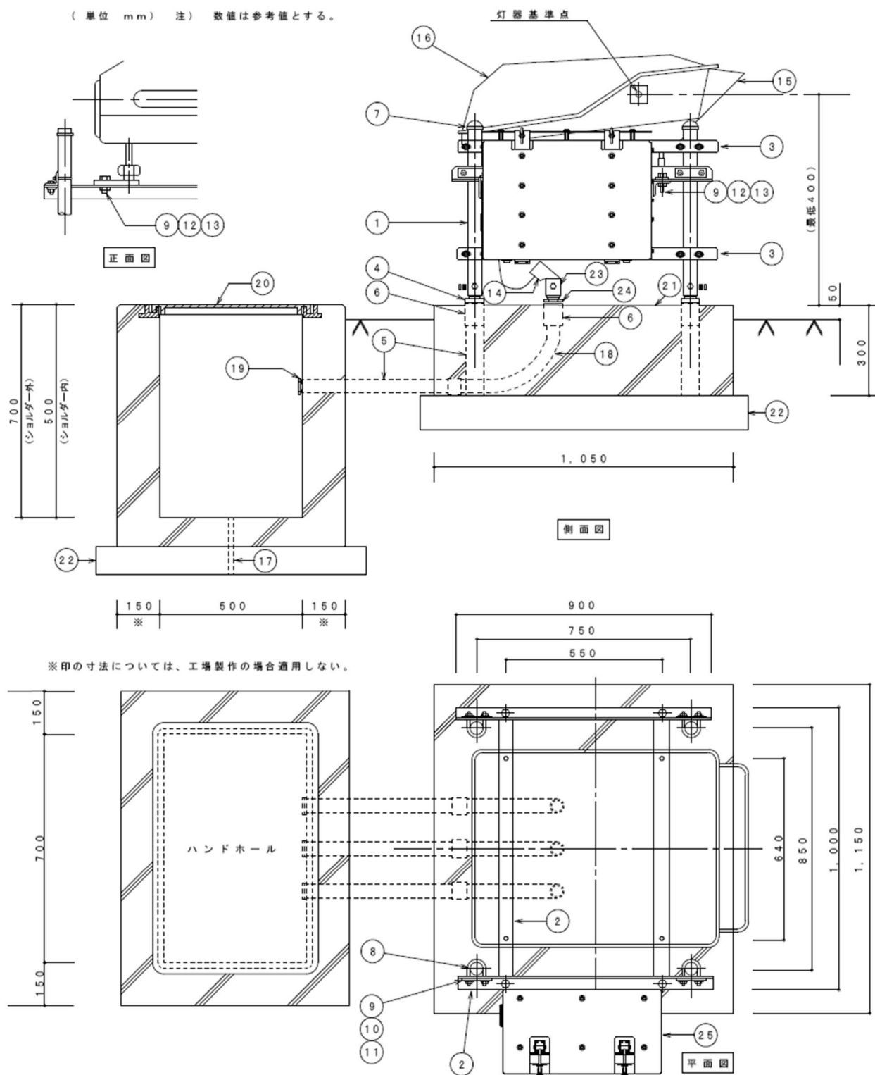
図2-44 進入角指示灯（LED式）の灯器基礎
