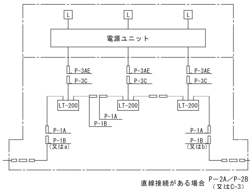
図４－１８ 進入角指示灯の配線接続要領（1台分）（LED式）
