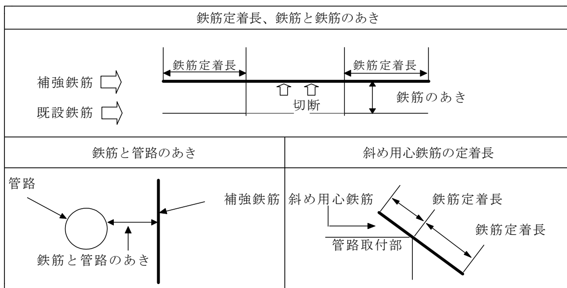
図 4.3 鉄筋定着長等の定義
