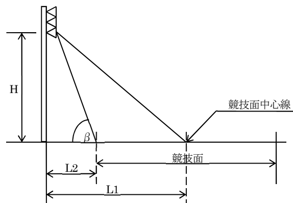
図-3 器具取付高さ
