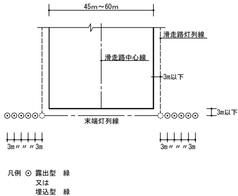
図2-9 滑走路末端補助灯の配置
