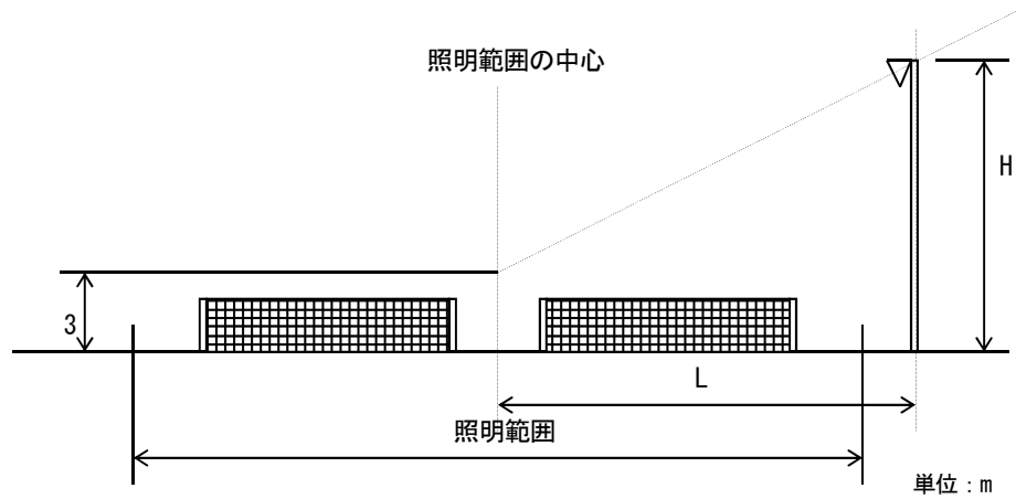
図－１０ 器具取付高さ
