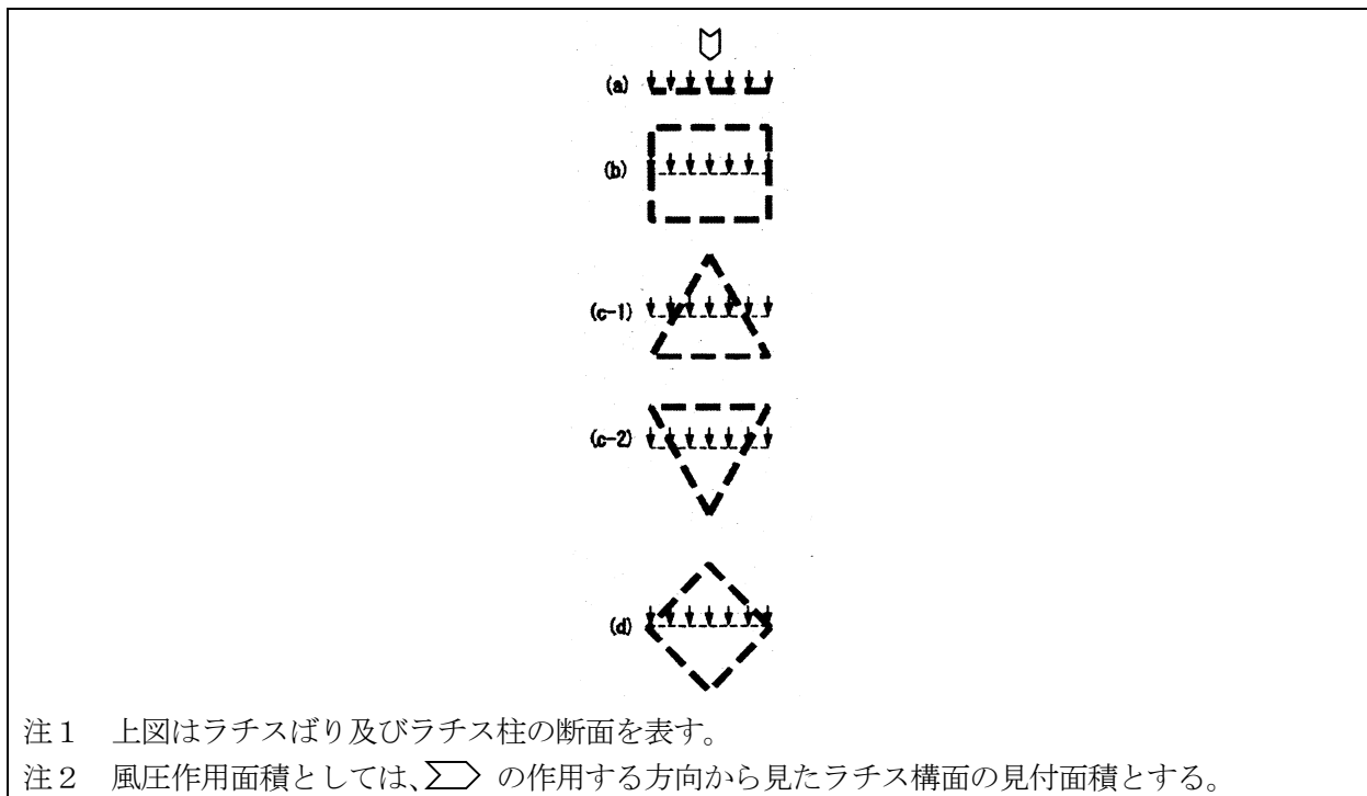
図五 ラチス構造物（表七を用いるものとする。）
