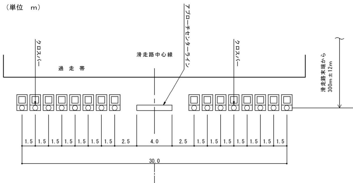
図 2 - 5 6 クロスバーの灯器配置
