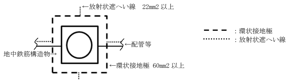
図 7-2 地中鉄筋構造物等への雷保護
