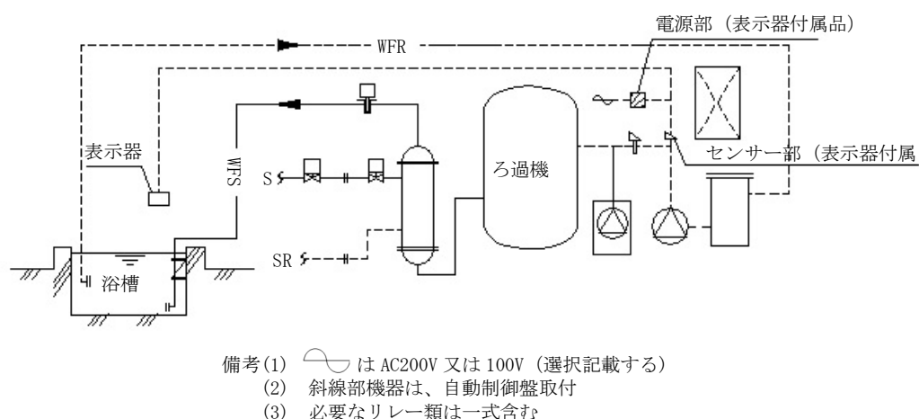
図３－２ 浴槽水温度表示システム図（参考）
