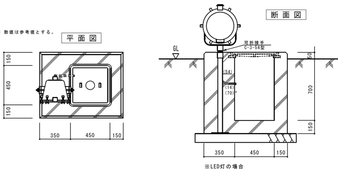
図 2－7 2 滑走路末端識別灯の灯器基礎
