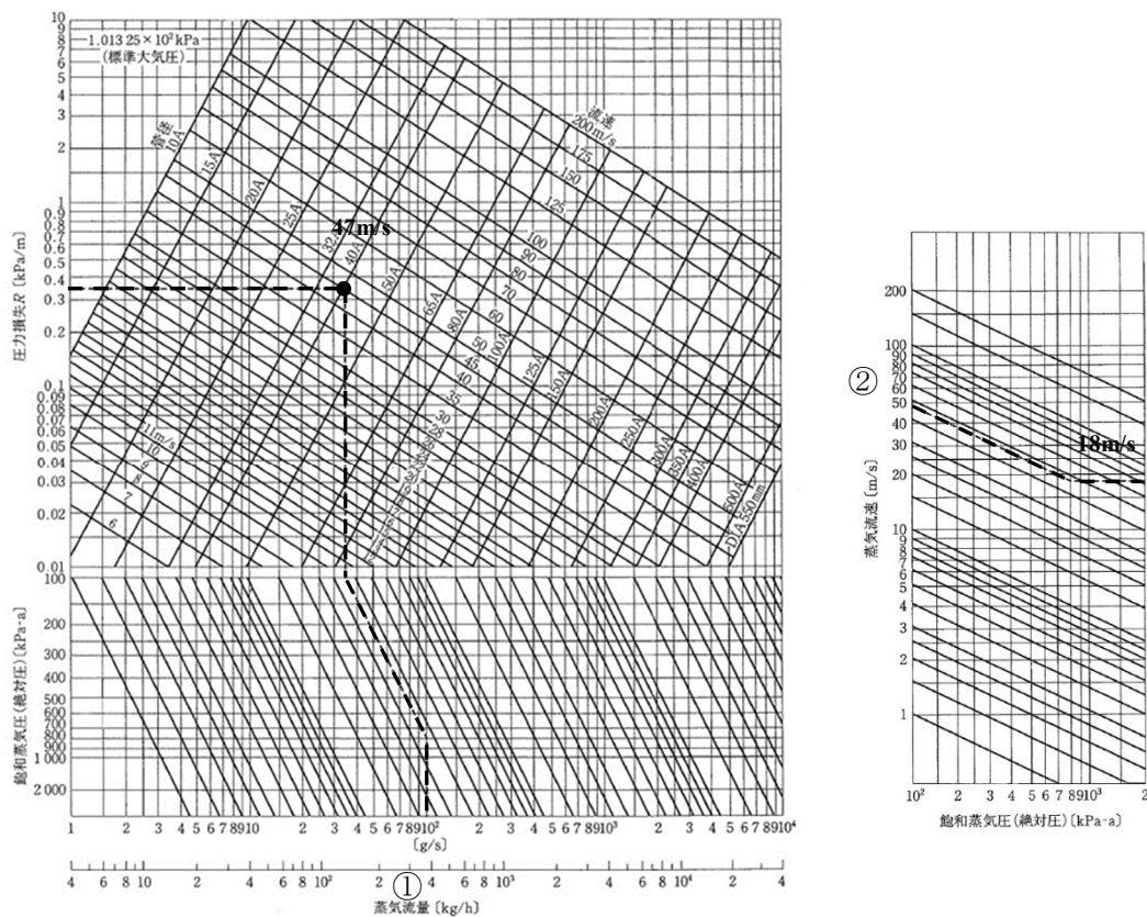
図 5 - 4 蒸気配管流量線図 (空気調和・衛生工学便覧第 14 版)
