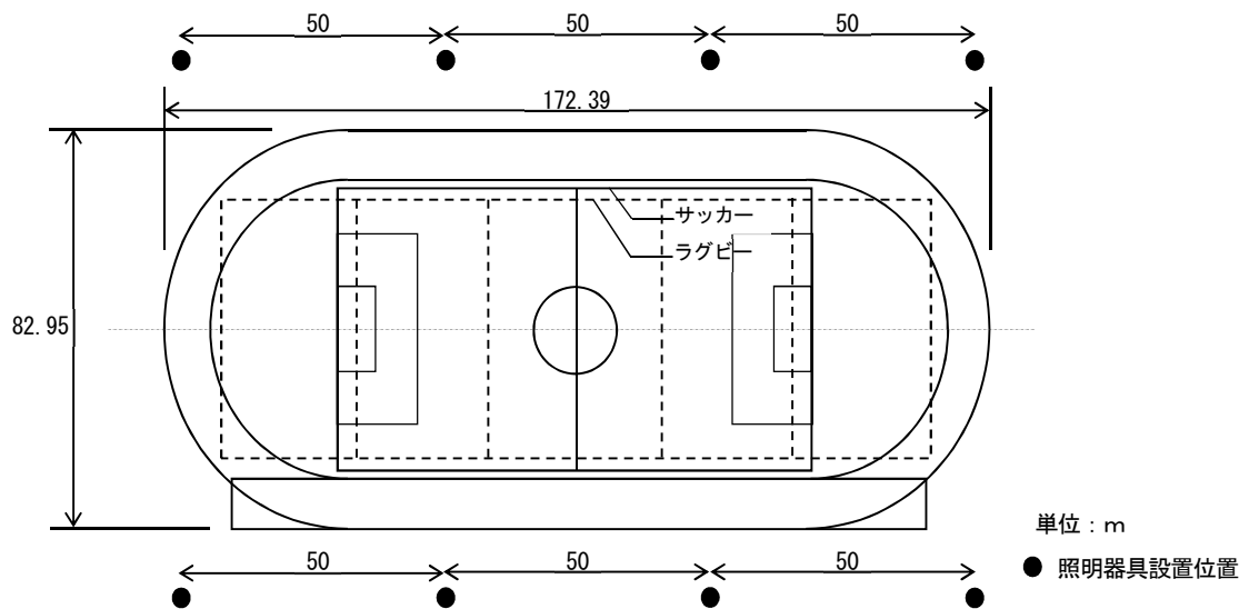
図-2 運動施設平面図
