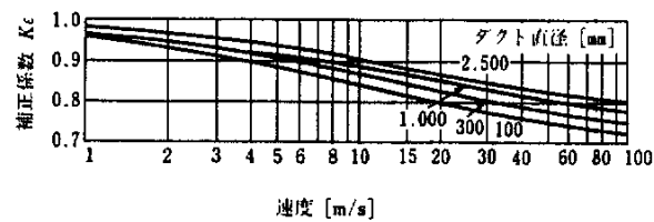
図 6 - 1 ( d ) 絶対粗さ ( \varepsilon=0.03\text{mm} ) に対する補正係数*
