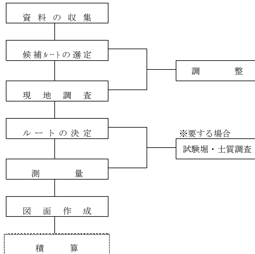
図2.1 線路土木設計の手順
