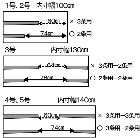
図3.1 ケーブル受け金物組み合わせ例
