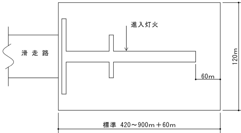
図2-54 灯火平面区域
