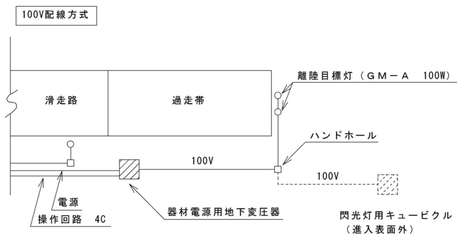
図 4-7 離陸目標灯の配電方式 (1)
