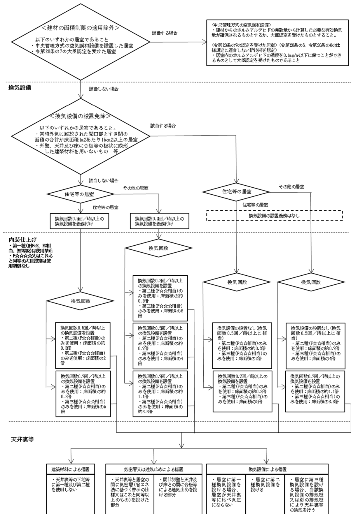
図4-1 建築材料と換気設備が相互に関する技術基準の全体フロー
