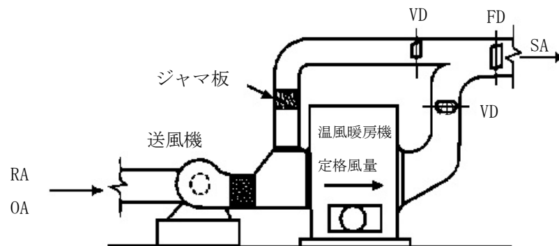
図 1-1 温風暖房機設置例
