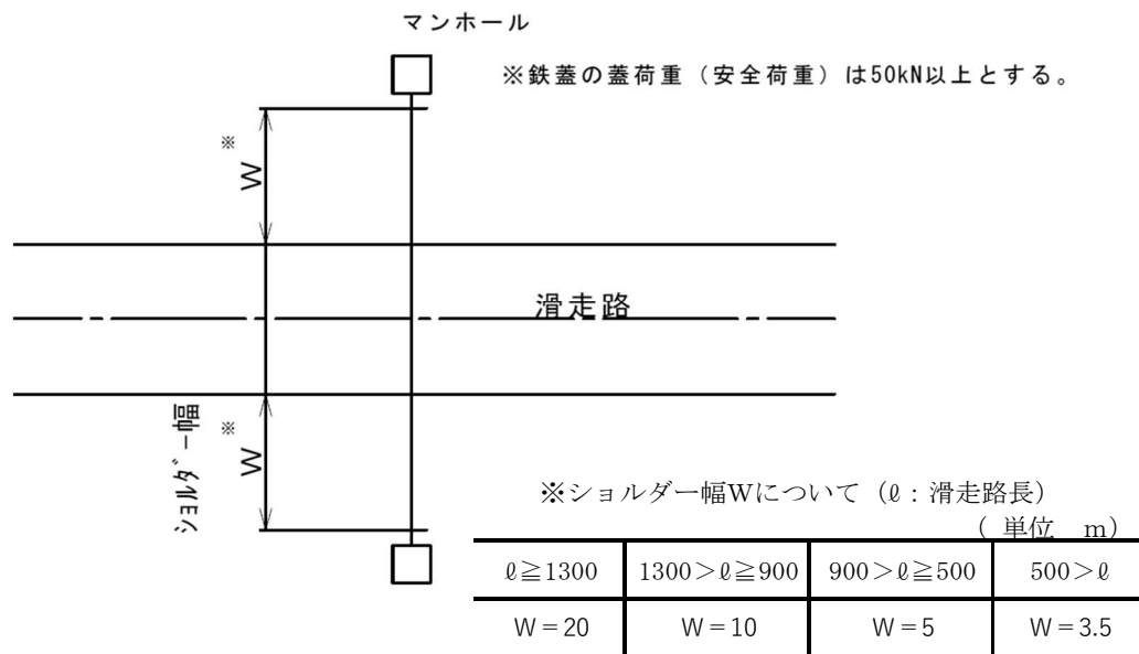
図4-1 滑走路下横断管路の設置位置
