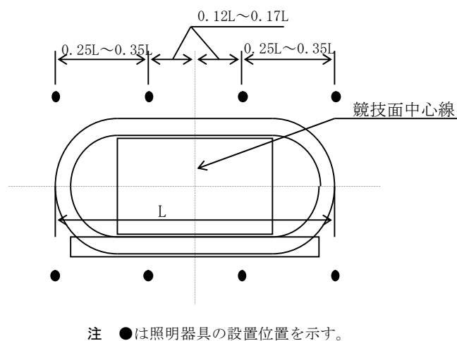
図9-8 陸上競技場及び複合競技施設（陸上競技場・サッカー場・ラグビー場）の照明器具の配置（8か所配置の場合）
