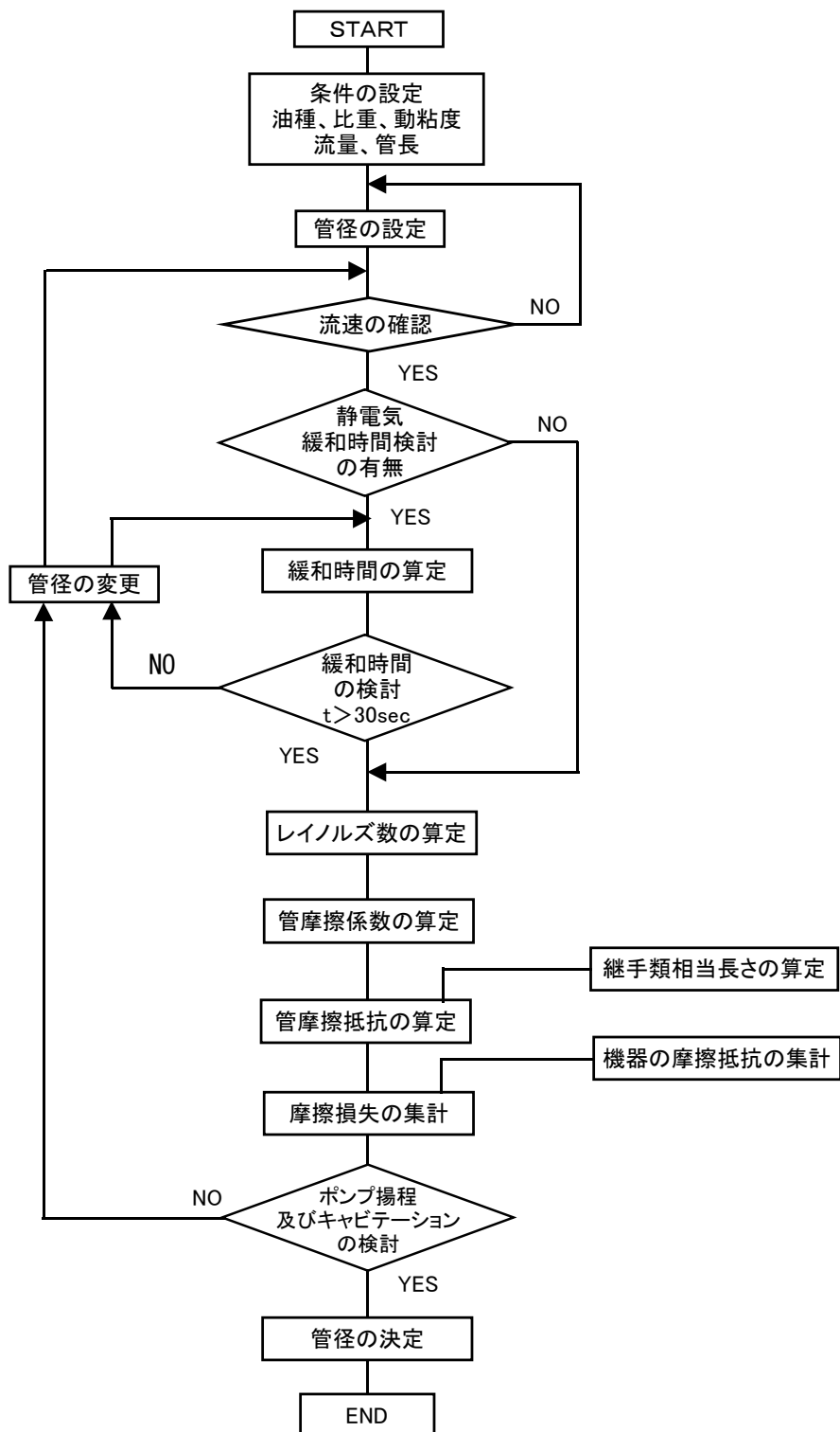
図3-2 配管の設計手順
