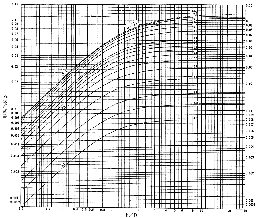
図 3 - 1 3 人体の等価球に対するふく射ヒーター設置面の形態係数
