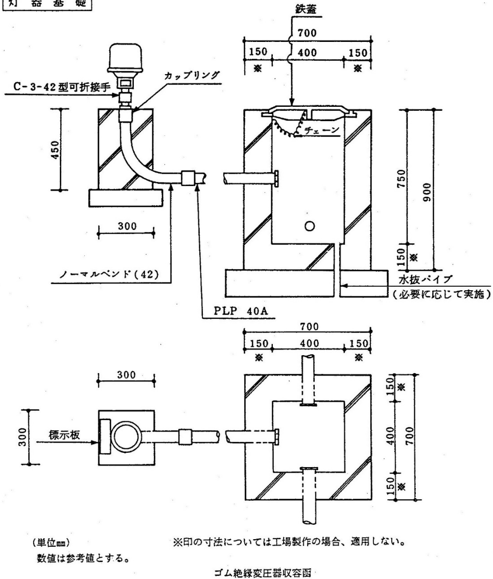
図 2-2 滑走路灯（露出型）の灯器基礎及びゴム絶縁変圧器収容函
