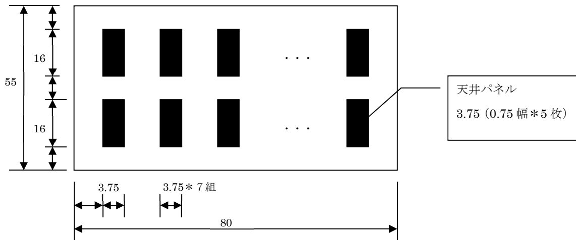
図 3 - 2 天井パネル配置計画例
