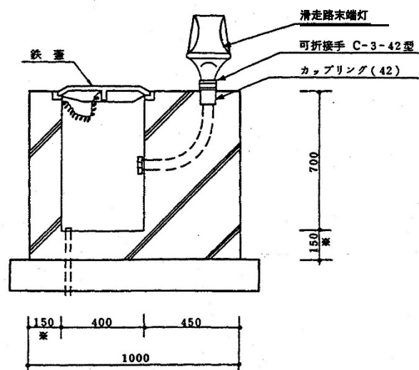
図 2 - 1 2 滑走路末端灯 (露出型) 基礎
