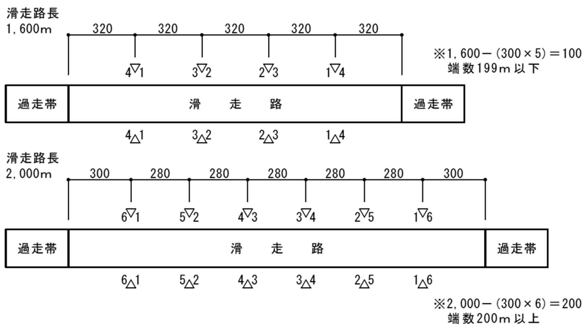
図 2 - 2 1 滑走路距離灯の灯器間隔調整
