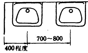
平面
