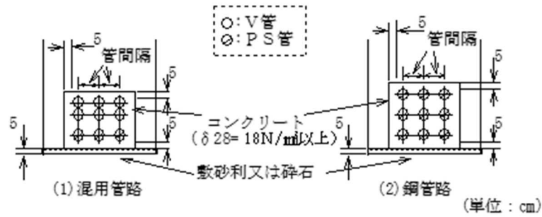
図2.4 コンクリート防護（注：条数は例）
