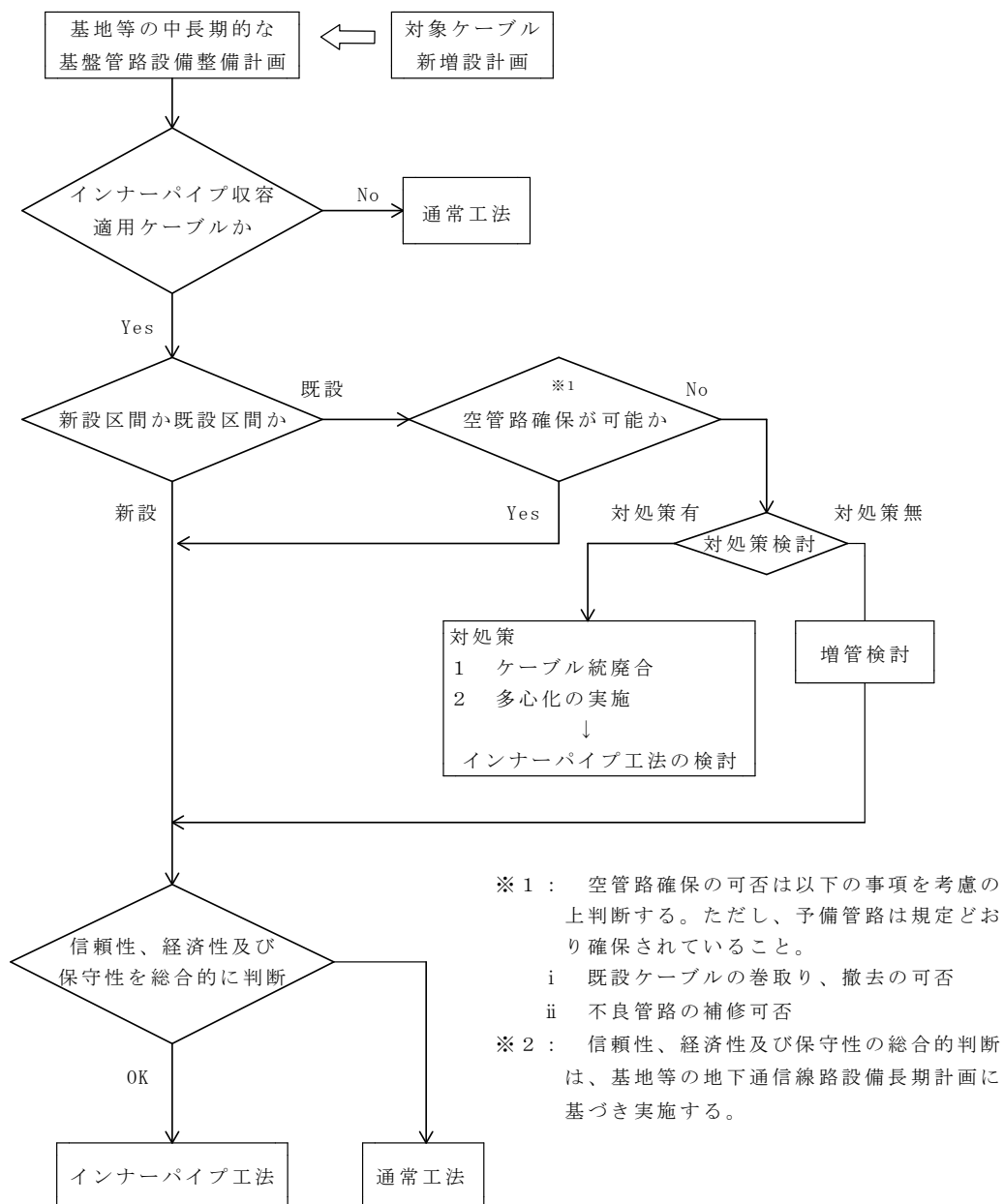
図 2.1 インナーパイプ工法適用検討の流れ
