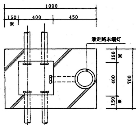
図 2 - 1 2 滑走路末端灯 (露出型) 基礎
