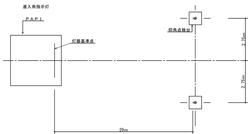
図 2-40 仰角点検台配置図
