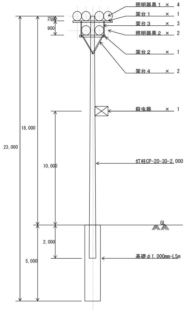
図－5 照明灯柱姿図
