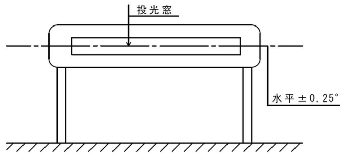
図2-33 光学系の許容差
