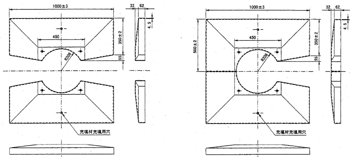
滑走路末端灯保護枠（FHB型用）
