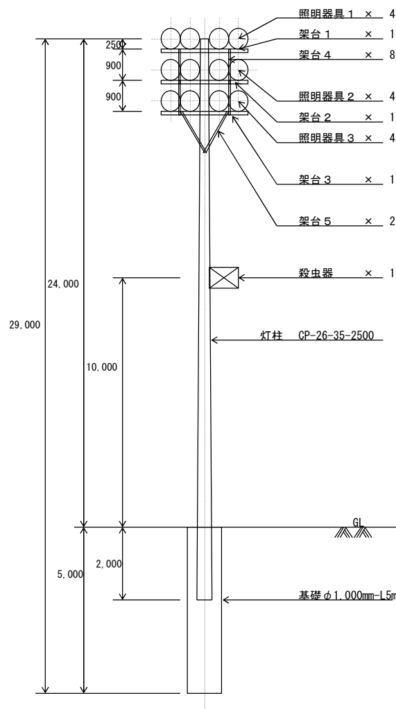
図－8 照明灯柱設備図
