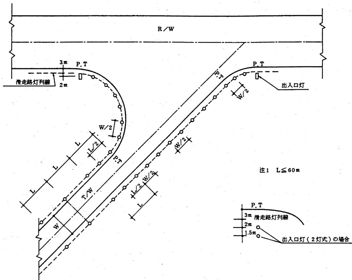
図 2-23 誘導路灯の配置 (1) (滑走路と交差する場合)
