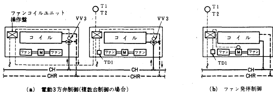
図 1-1 システム図
