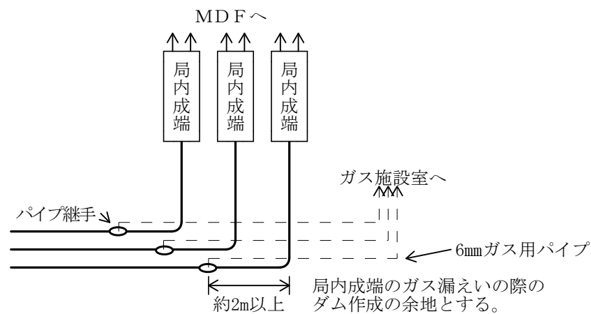
図2.12 ケーブルのガス用パイプ取付位置図
