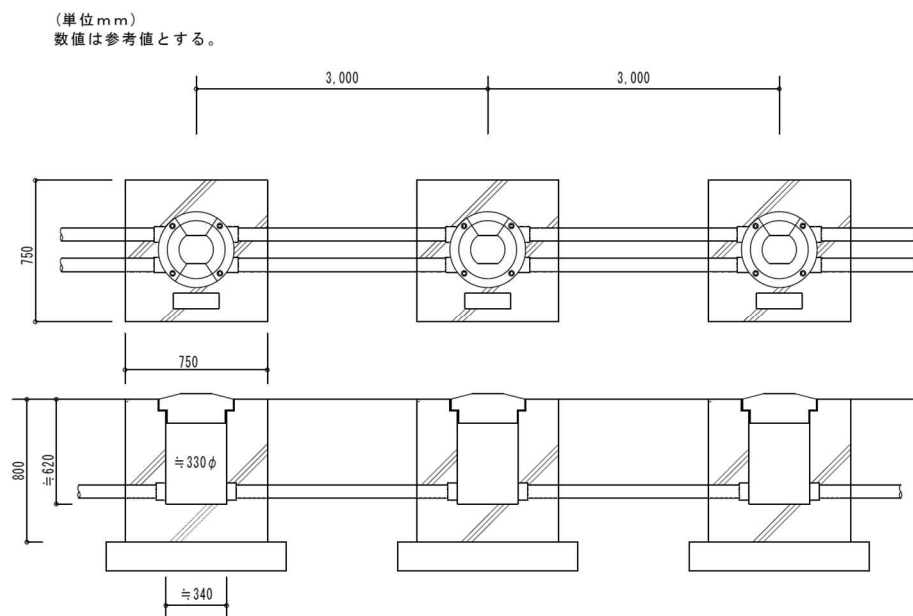
図 2 - 1 6 滑走路末端補助灯（埋込型）基礎
