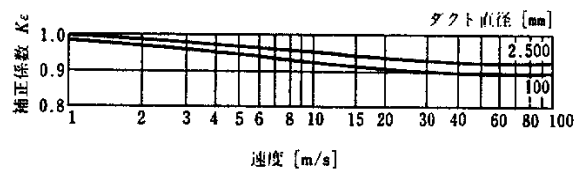
図 6 - 1 ( c ) 絶対粗さ ( \varepsilon=0.09\text{mm} ) に対する補正係数*
