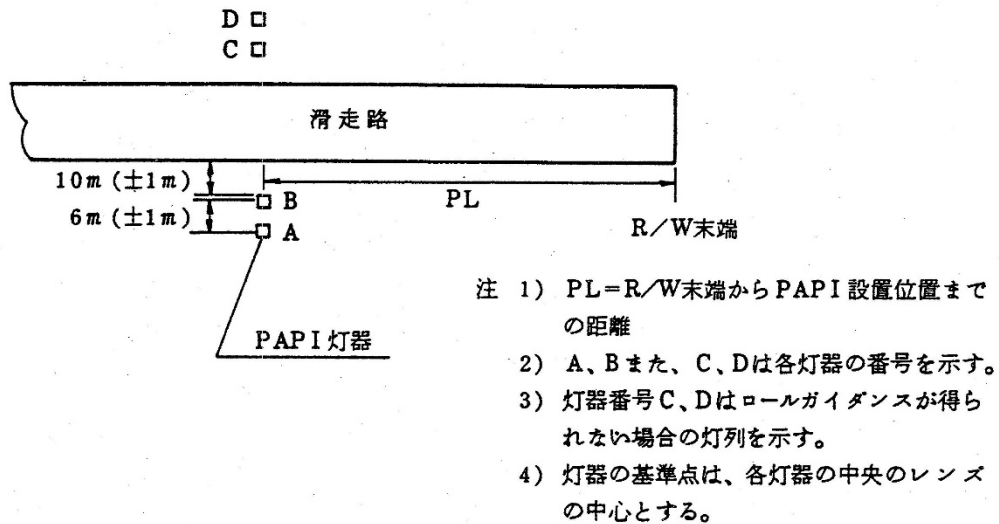
図 2 - 4 9 A P A P I 方式灯器配置図
