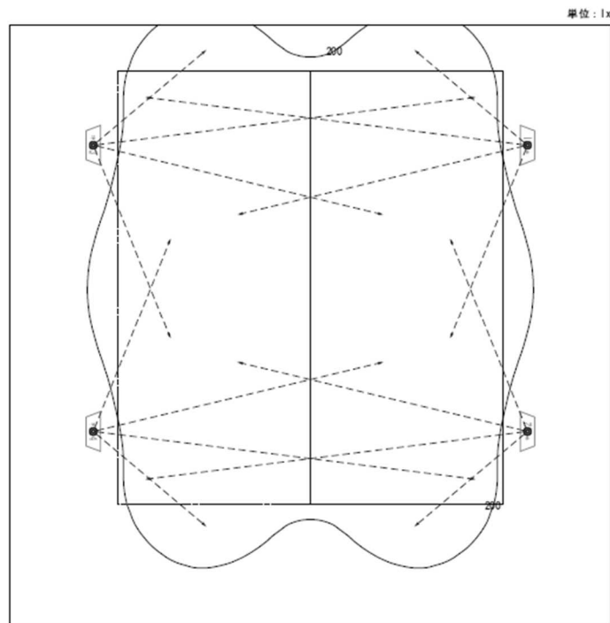
図－１１ 照度分布図
