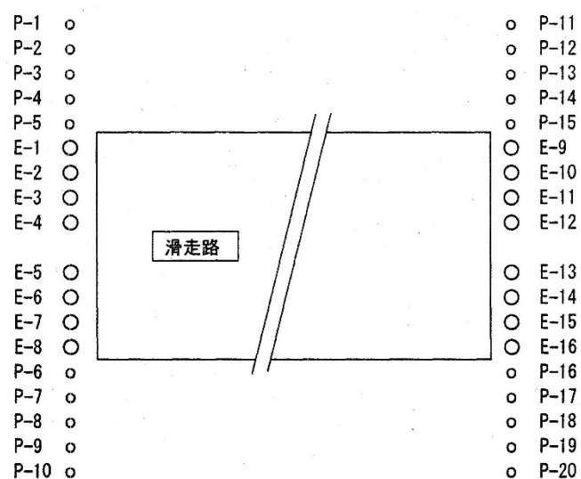
図 2-17 灯器番号例
