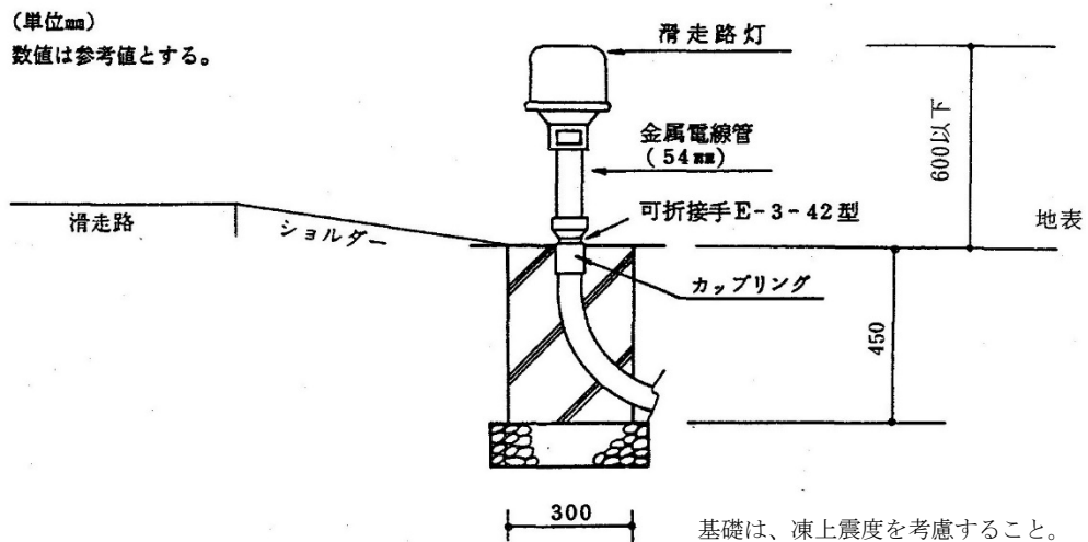
図 2-3 滑走路灯（露出型）の灯器基礎（積雪地）
