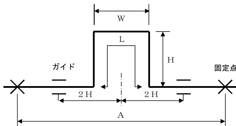
図 5 - 1 ループ式伸縮継手寸法図
