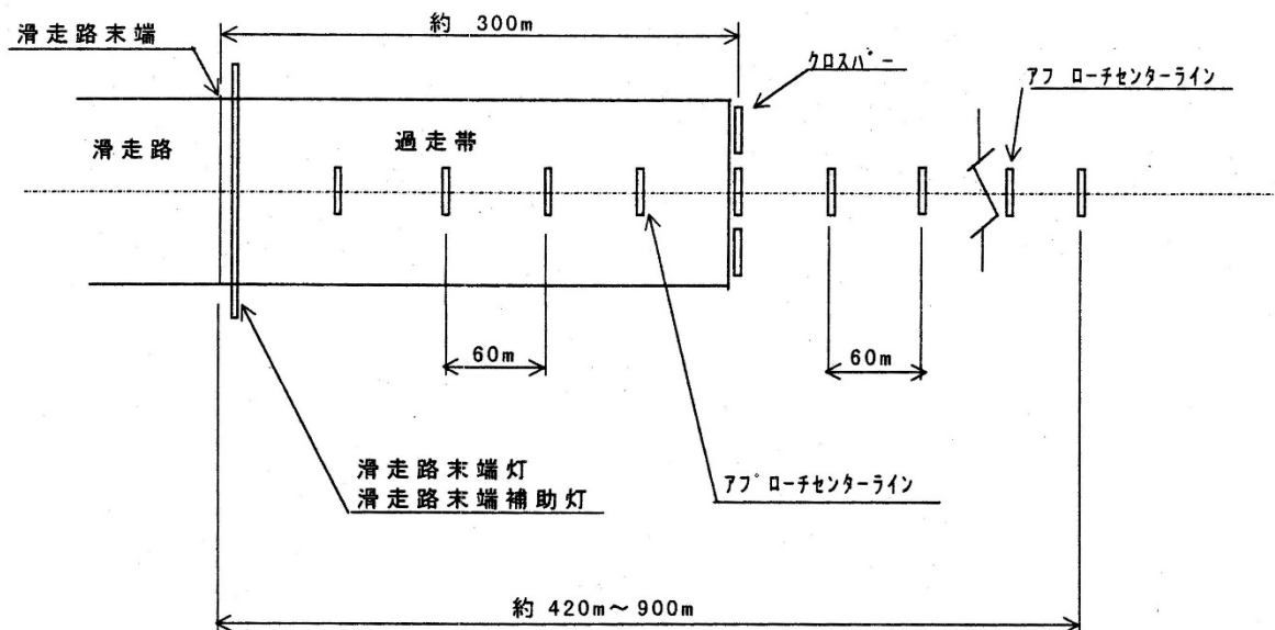
図2-69 進入灯の配置図（簡易式）
