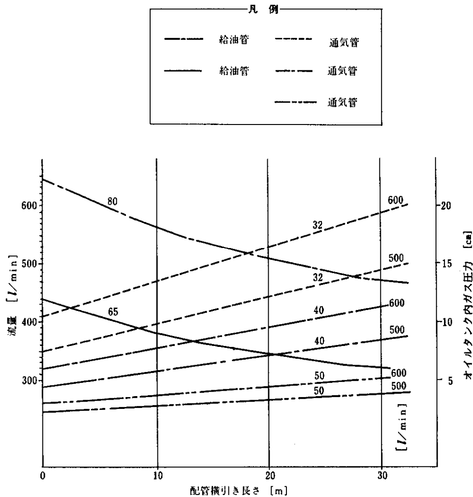
図 4-1 注油管・通気管選定図
