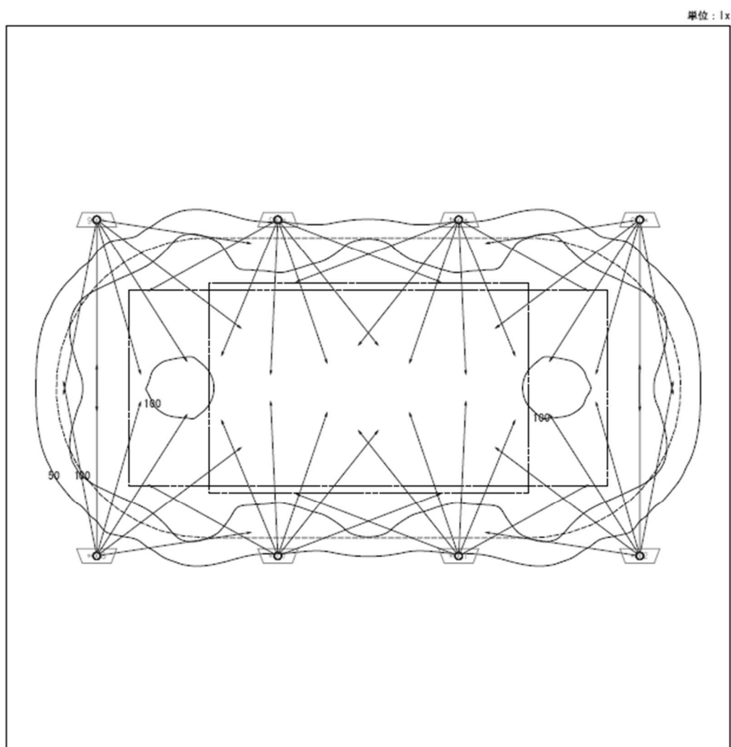
図－４ 照度分布図
