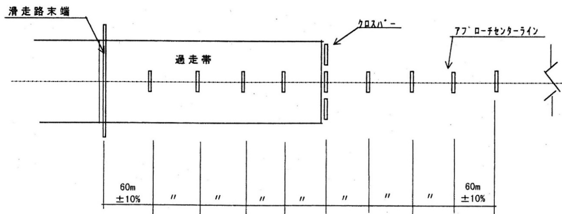
図2-70 灯列間隔の裕度（簡易式）
