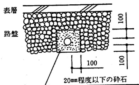
路盤内埋設配管参考図
