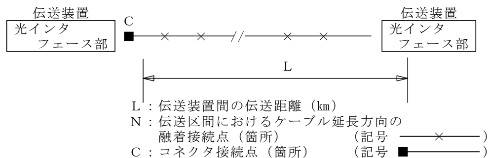
図6.1 伝送装置間のモデル
