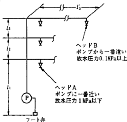
スプリンクラー系統図
