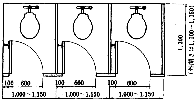
1 洋風便器
