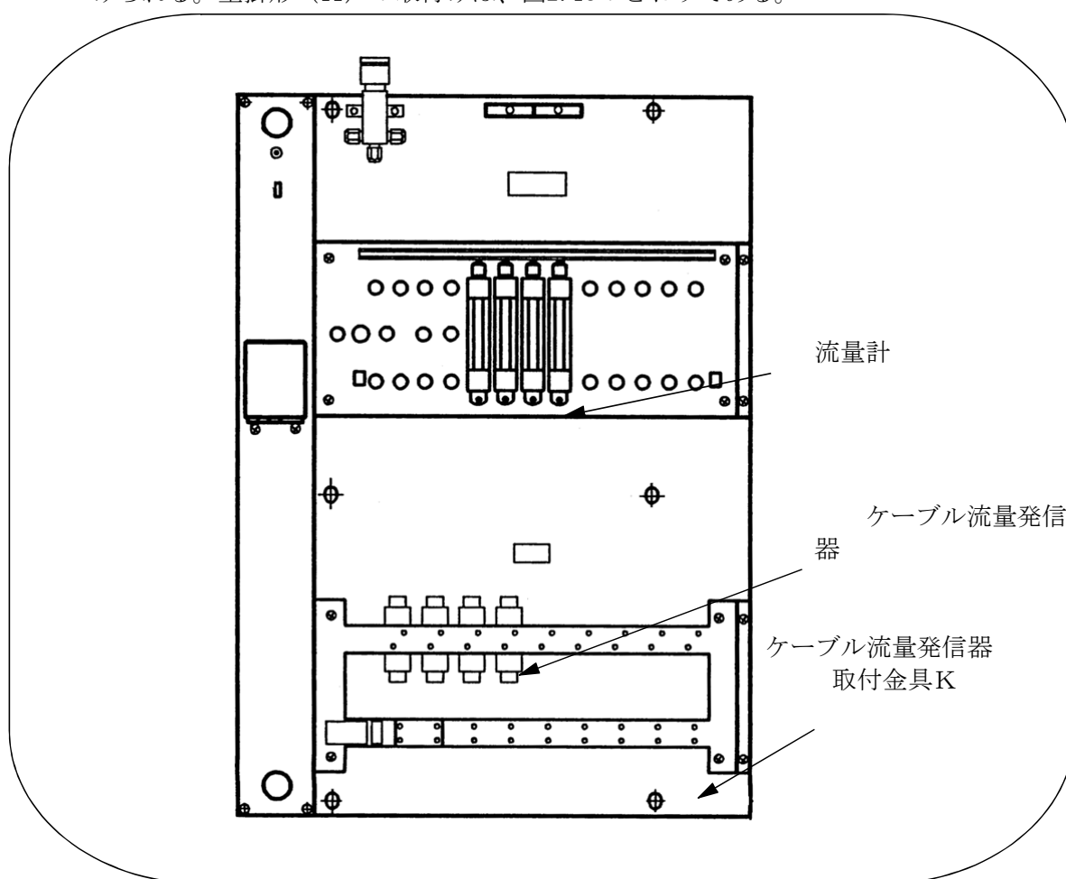
図2.13 流量監視器の壁掛形ガス分配装置への取付図
