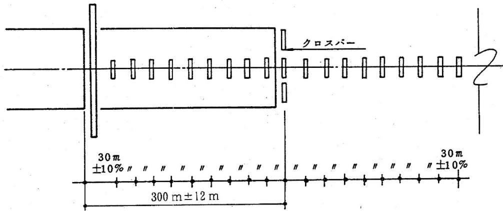
図 2-52 灯列間隔の裕度（標準式）
