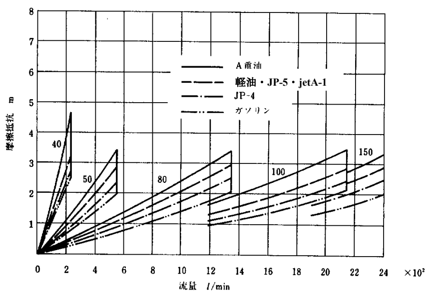
図 3 - 4 ストレーナの摩擦抵抗
