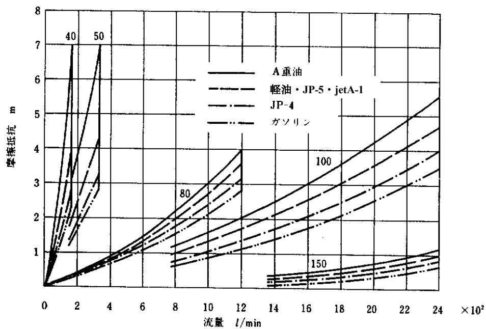
図 3 - 3 流量計の摩擦抵抗
