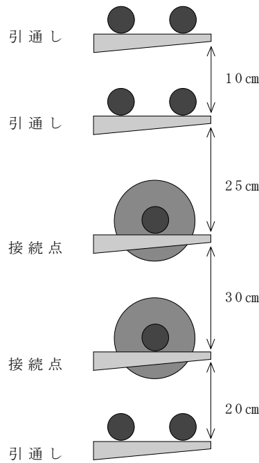
図 3.2 ケーブル受け金物の取付間隔
