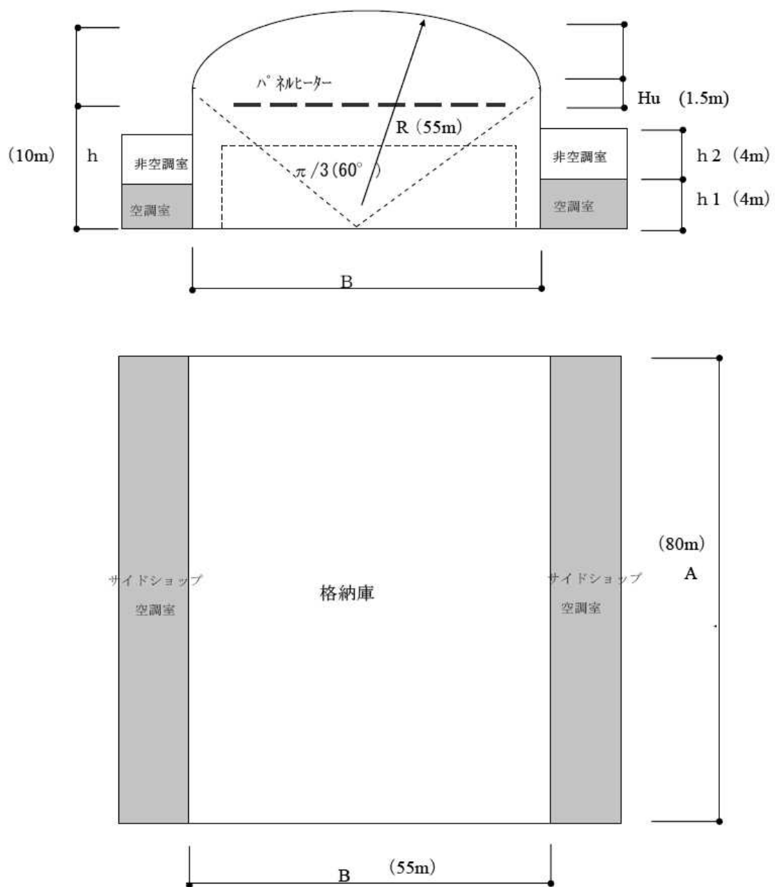
図 3 - 1 格納庫平面図および断面図
