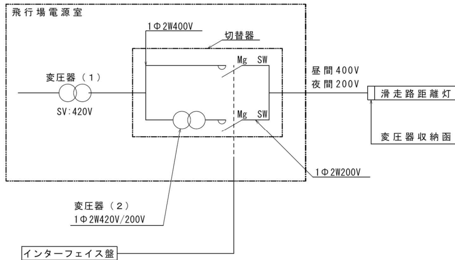
図 4-1 1 滑走路距離灯の配電系統
