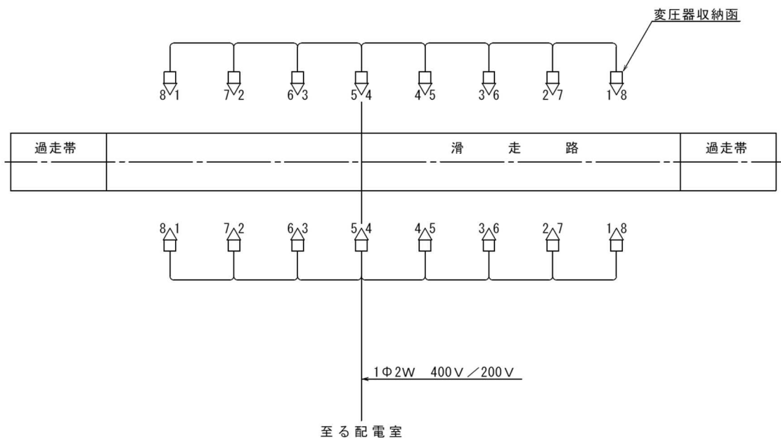
図4－12 滑走路距離灯の標準配線
