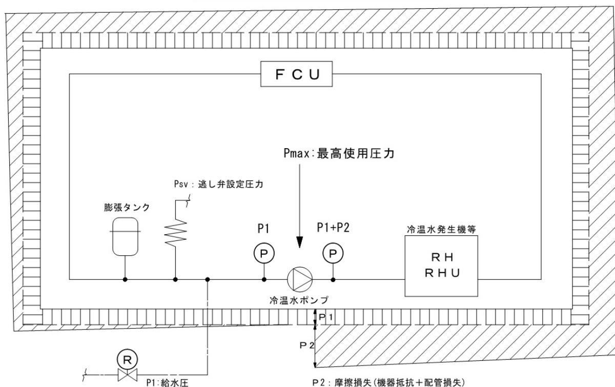
図5-1 配管圧力図
