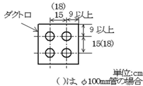
図2.9 管路相互の中心間隔
