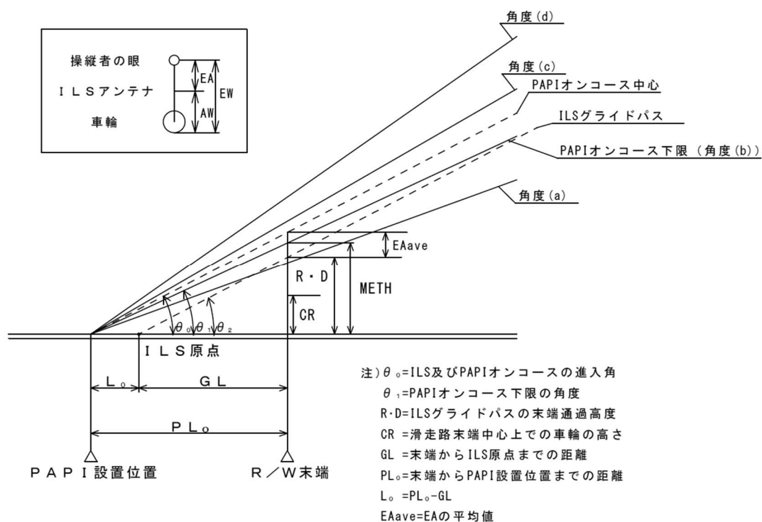
図 2-34 PAPI 設置位置関係図
