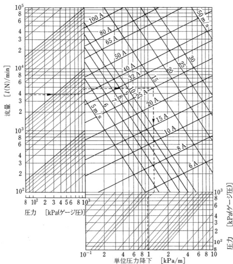
図5-7 配管用炭素鋼鋼管圧縮空気流量線図（空気調和・衛生工学便覧第14版）
