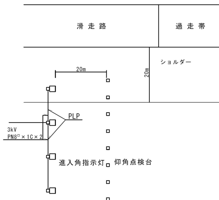
図 4 - 1 6 進入角指示灯 (PAPI) の配線
