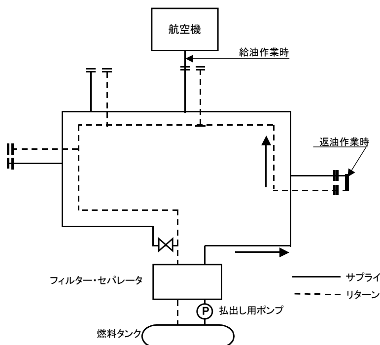
図3-1 航空機直接給油システム系統図
