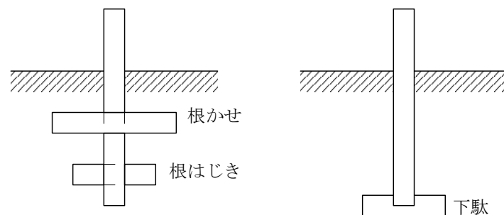
図3.3 根かせ、根はじき及び下駄
