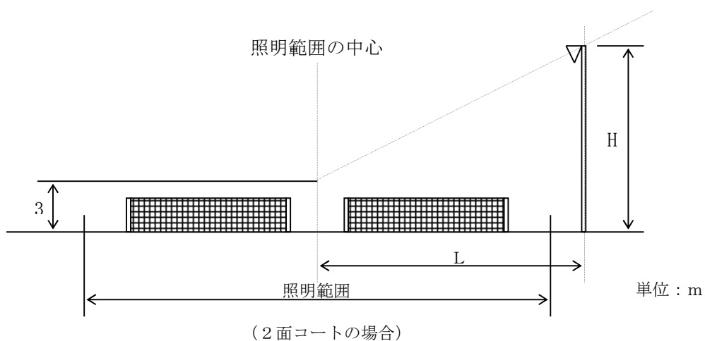
図9-4 テニスコートの照明器具取り付け高さ（2面コートの例）
