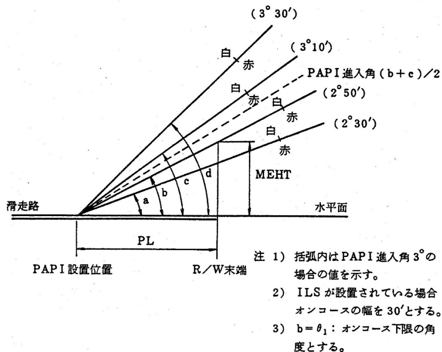
図 2-39 PAPI 設定仰角
