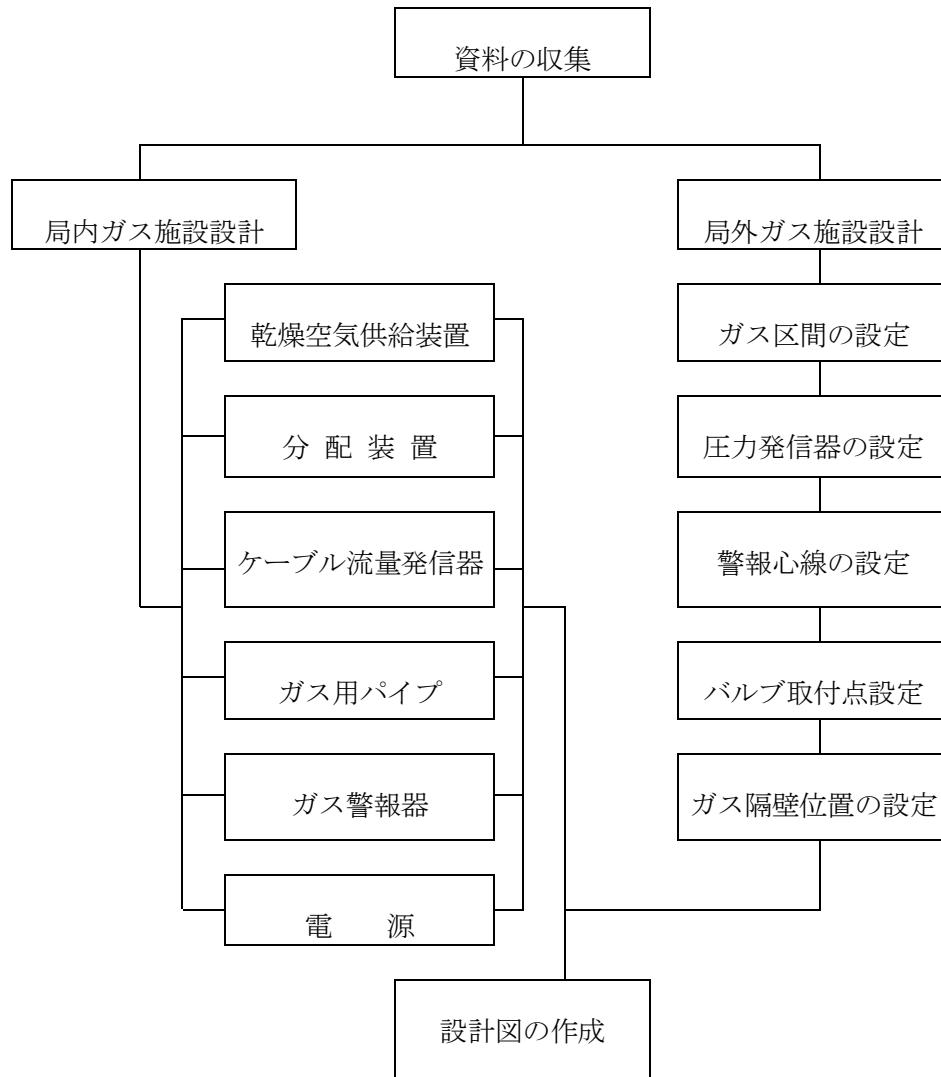
図2.10 ガス施設構成と設計手順
