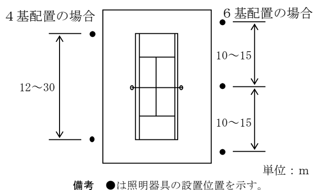
図9-3 テニスコートの照明配置
