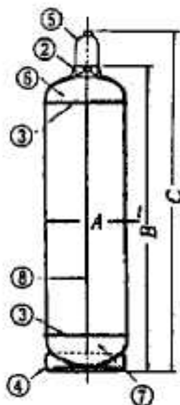
50kg L P ガス容器の寸法
