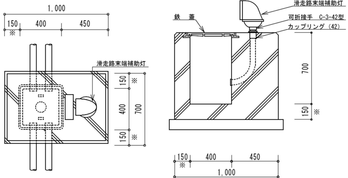
図2-14 滑走路末端補助灯（露出型）基礎
