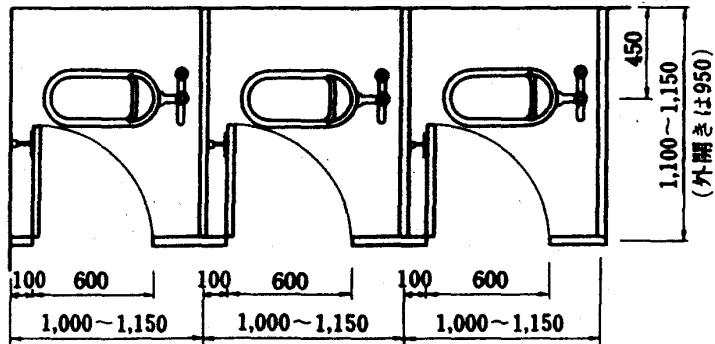
4 和風大便器
