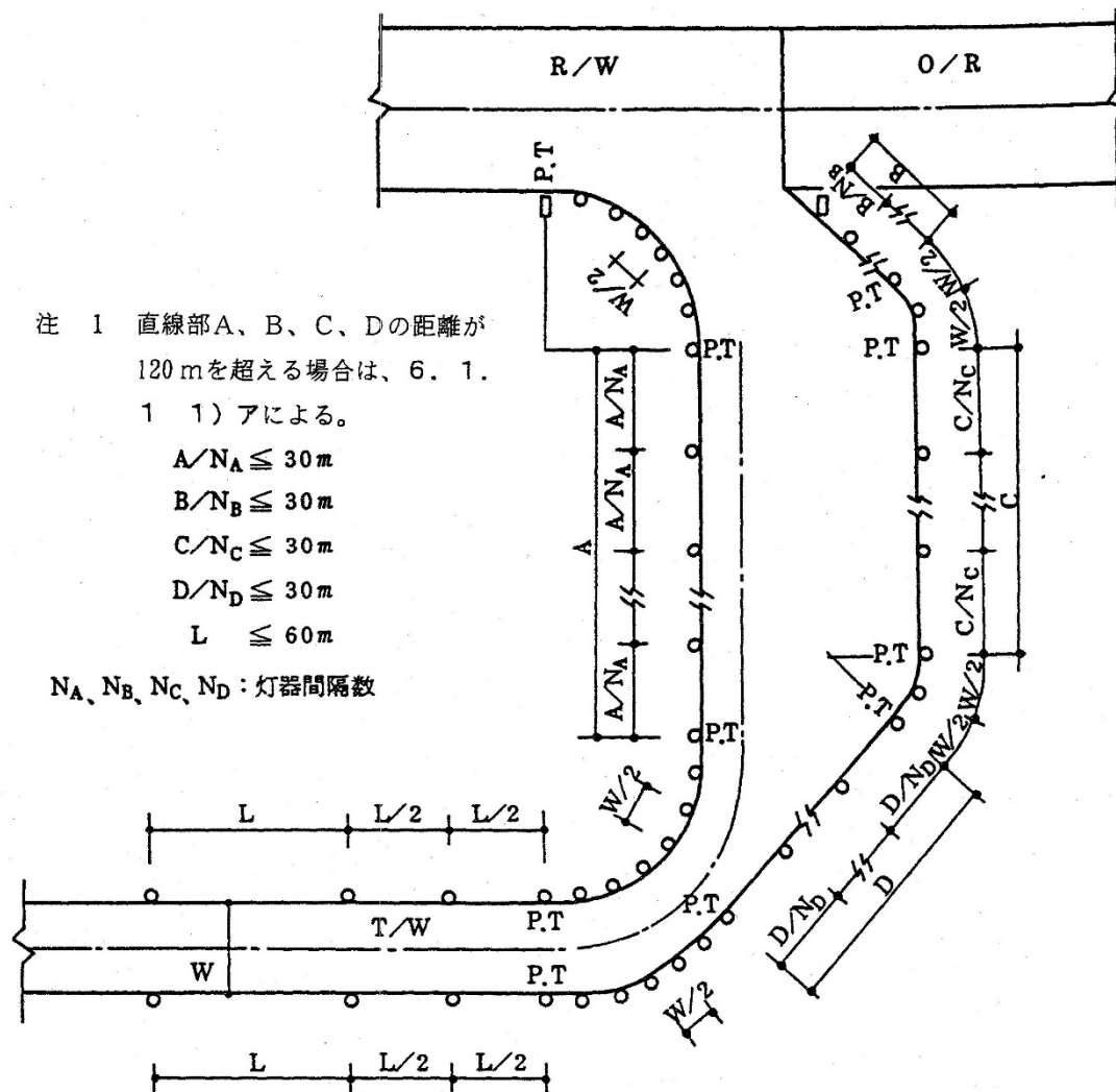
図 2-28 誘導路灯の配置 (6) (ウォームアップエプロンの場合)
