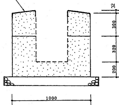
図 2 - 1 1 積雪地における埋込灯器周りの保護板参考図
