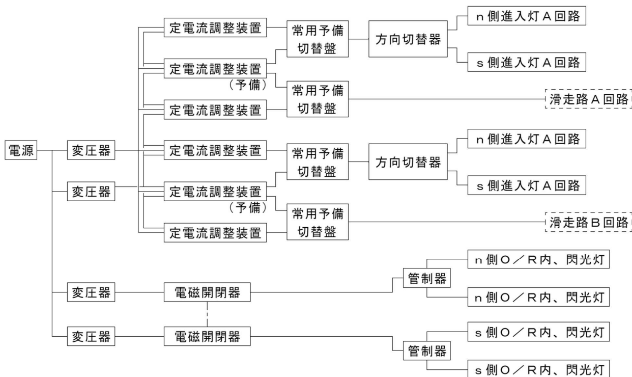
図 4-19 進入灯、連鎖式閃光灯配電方式
