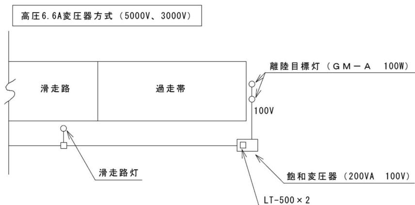
図 4-8 離陸目標灯の配電方式 (2)
