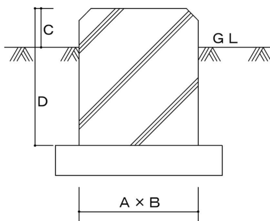
図 2-74 着陸方向指示灯及び風向灯の灯器基礎
