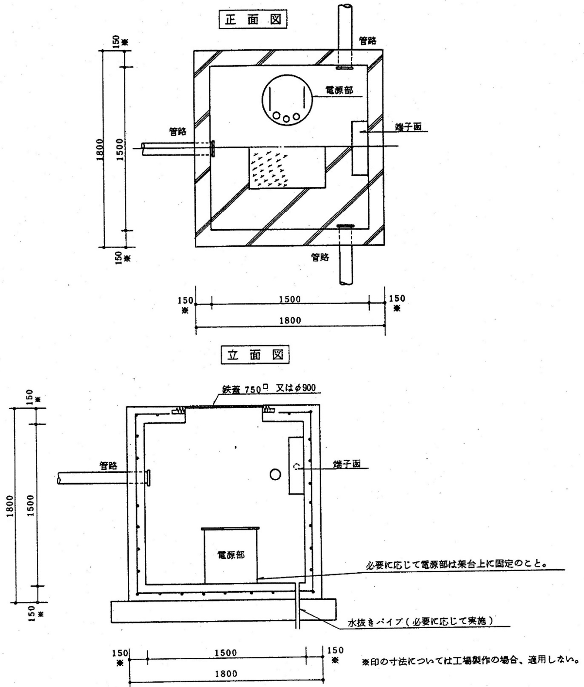
図 4 - 2 6 埋込型連鎖式閃光灯 (SFL) 用電源部收容マンホール (参考例)
