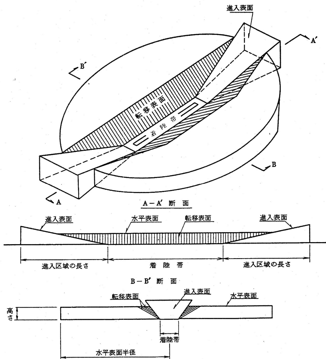
図2 進入表面等
