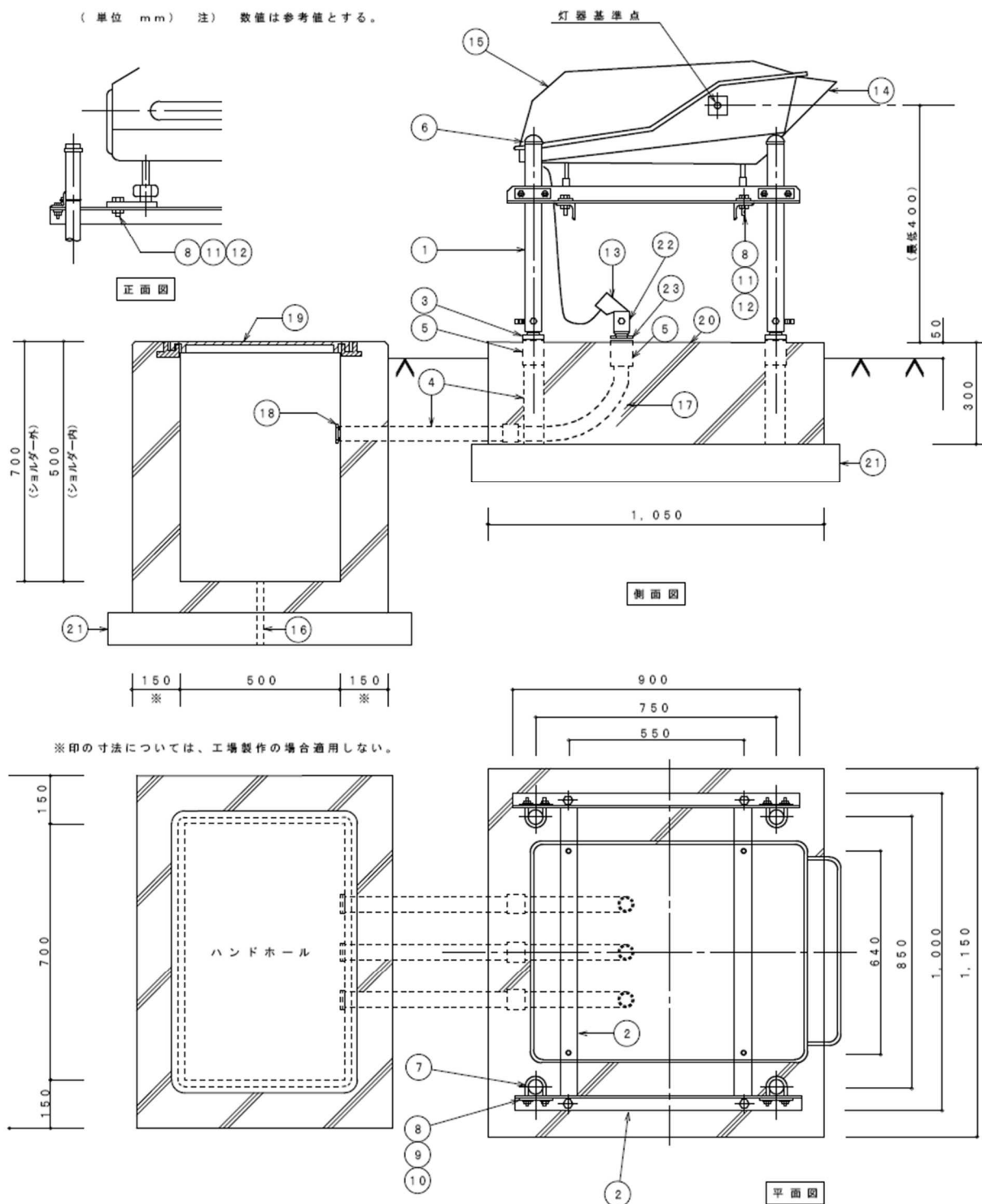
図 2-43 進入角指示灯（電球式）の灯器基礎
