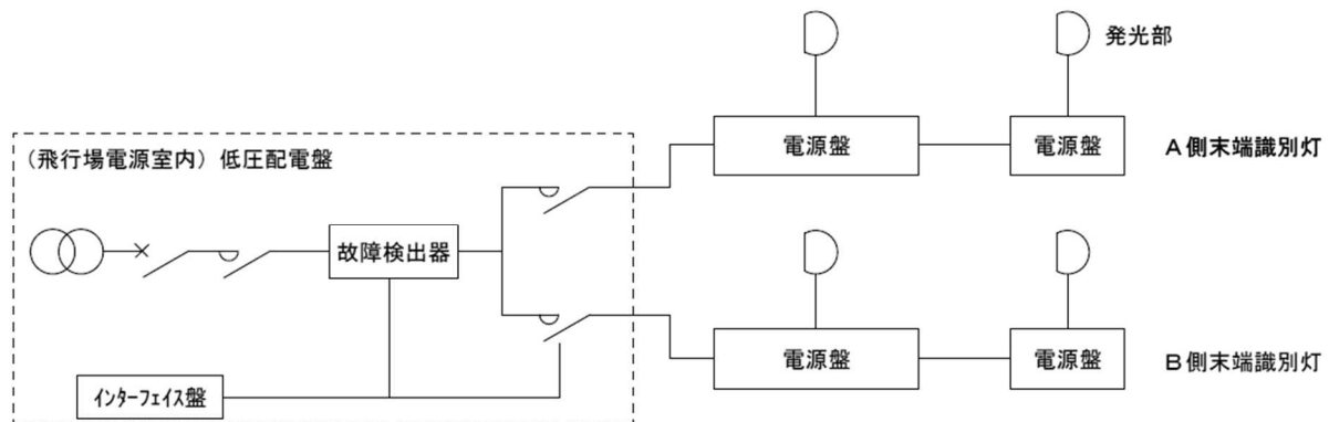
図 4-27 滑走路末端識別灯配線系統図
