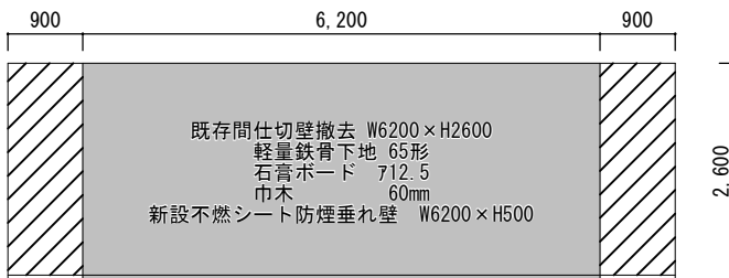
d 展開図
