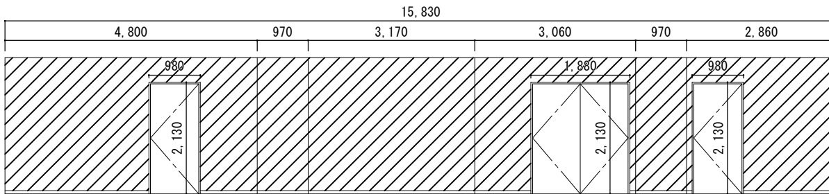
A 展開図
