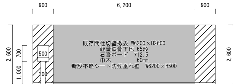
B 展開図
