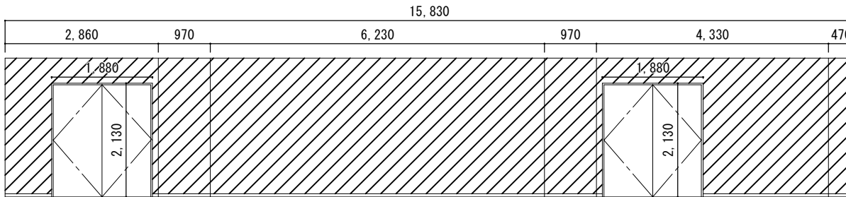
C 展開図
