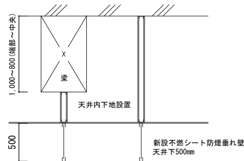
新設不燃シート防煙垂れ壁 詳細図
