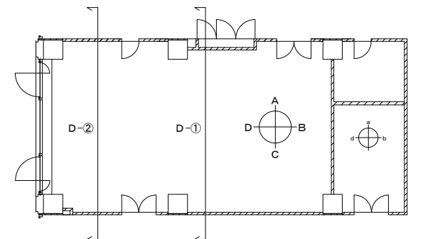
展開平面図 S=1/X
