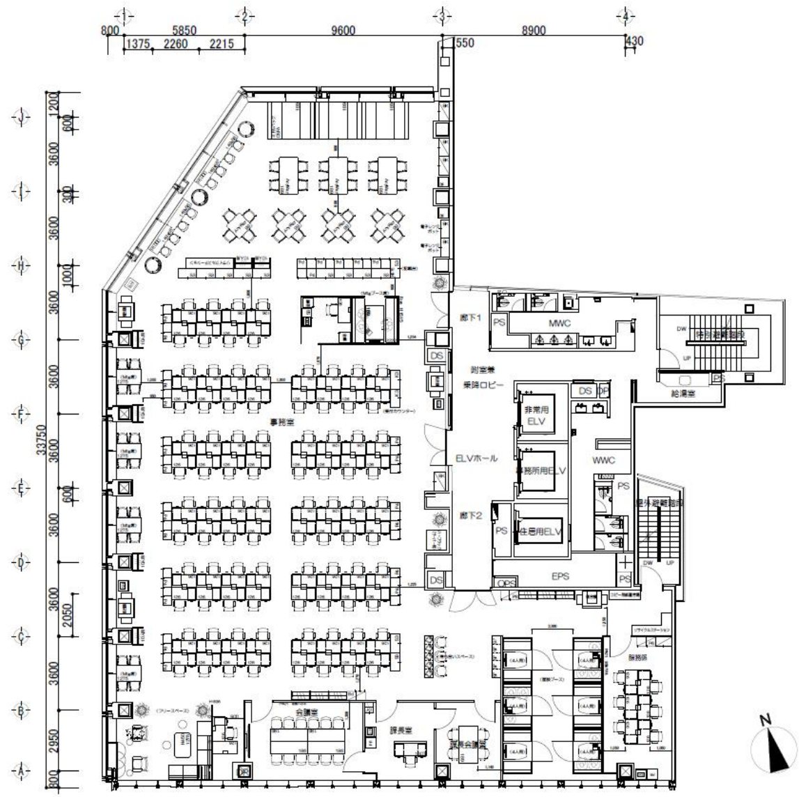
別図第6 部外不動産3階レイアウト移転後(秘書課)
