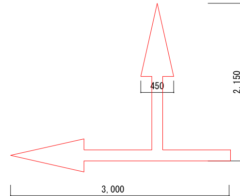
路面標示図 矢印④
