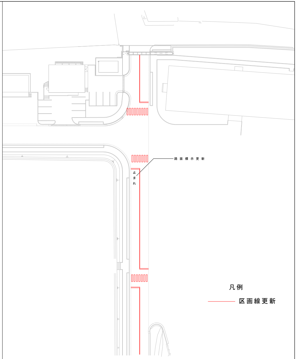
詳細図I S=1/800 図面番号 10/11
