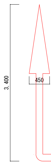
路面標示図 矢印①
