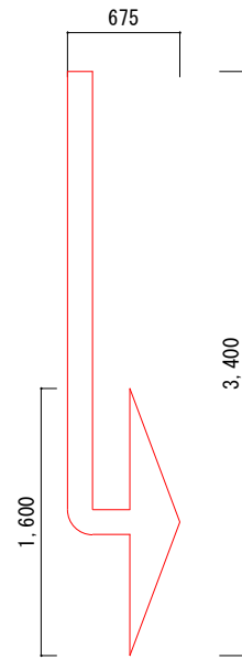
路面標示図 矢印②
