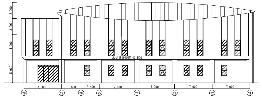
西側立面図
