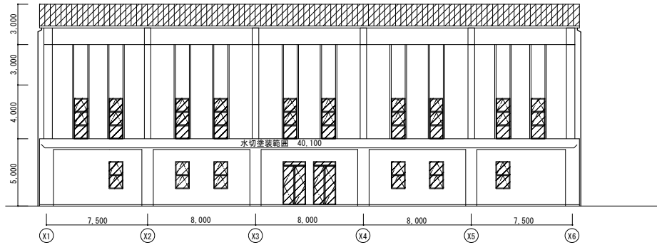
南側立面図
