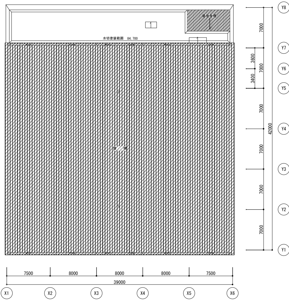
市ヶ谷体育館 屋根伏せ図 S=1:400
