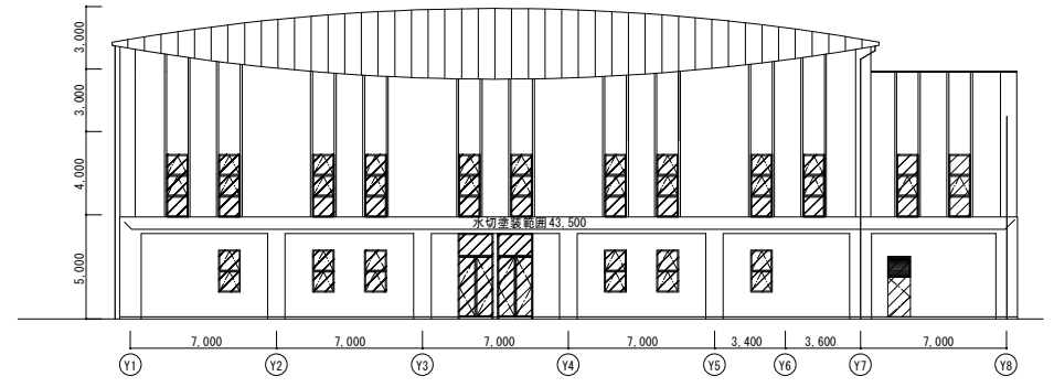
東側立面図
