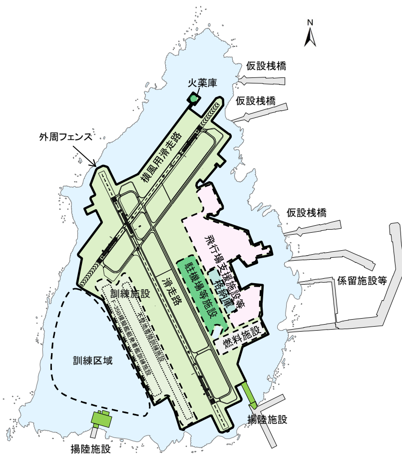
施設全体配置図
