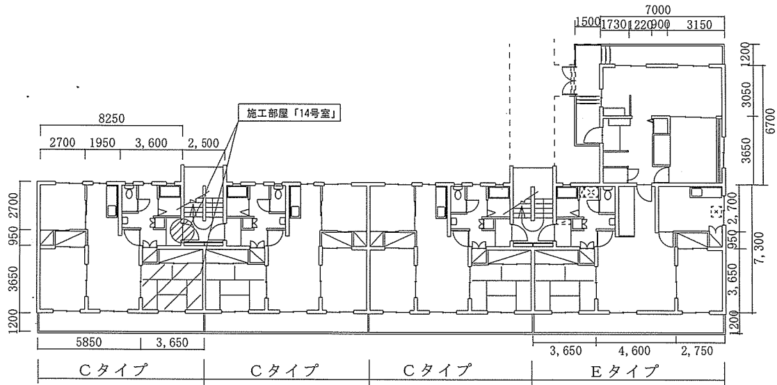
1階平面図
