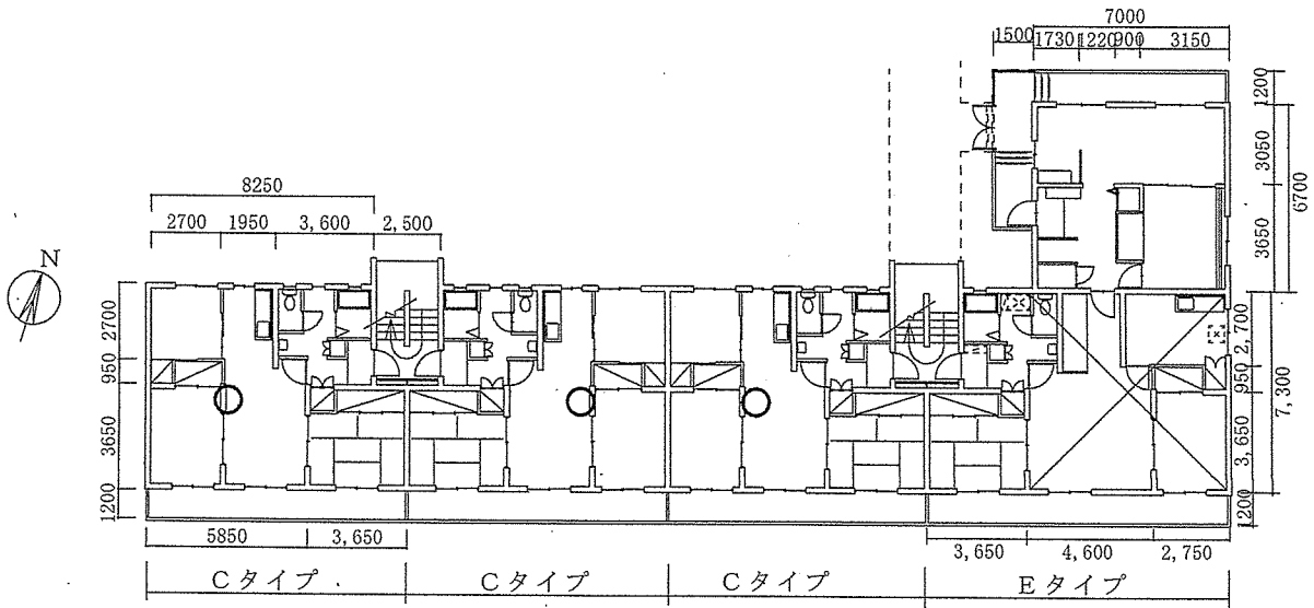
1階平面図
