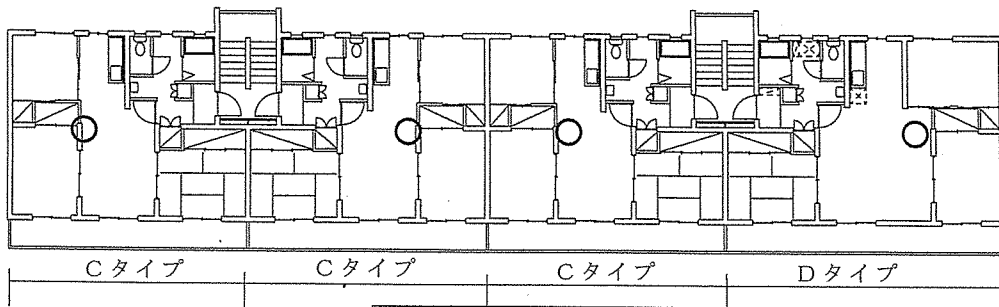
2階～5階平面図
