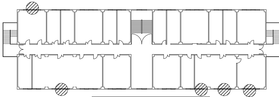
241号建物 2階平面図 S=1/x
