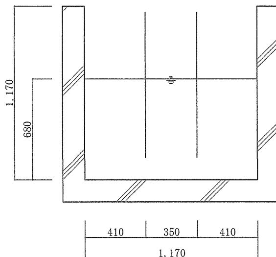
油分離槽① A-A' 断面図
