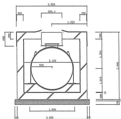
車両整備工場燃料地下タンク断面図② 1 / 80
