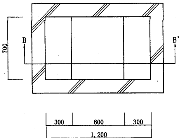
油分離槽③ 平面図
