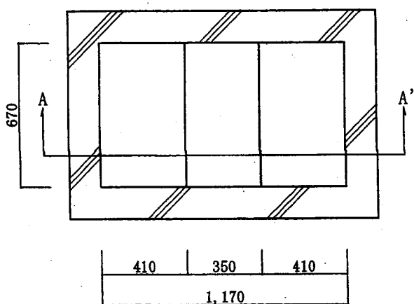
油分離槽① 平面図
