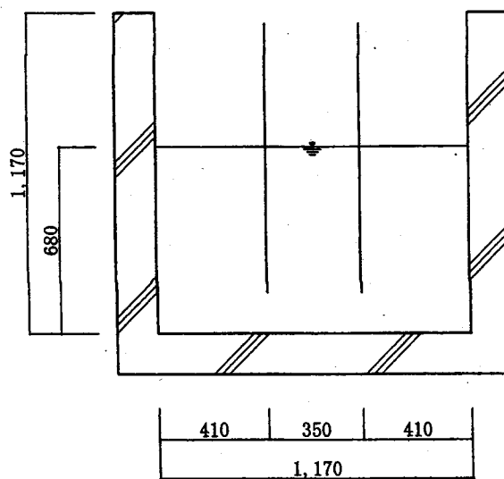
油分離槽① A-A' 断面図
