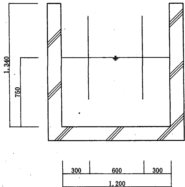
油分離槽③ B-B' 断面図
