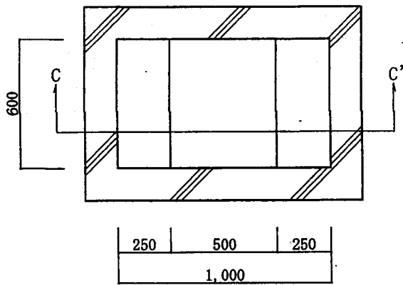
油分離槽② 平面図
