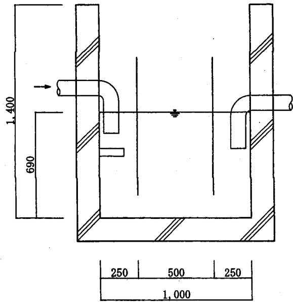
油分離槽② C-C' 断面図
