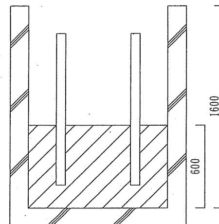
断面図
