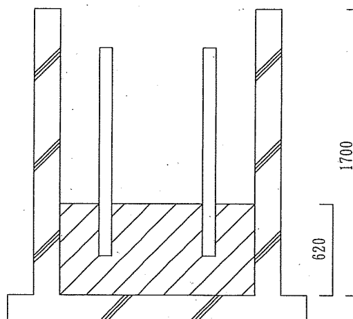
断面図
