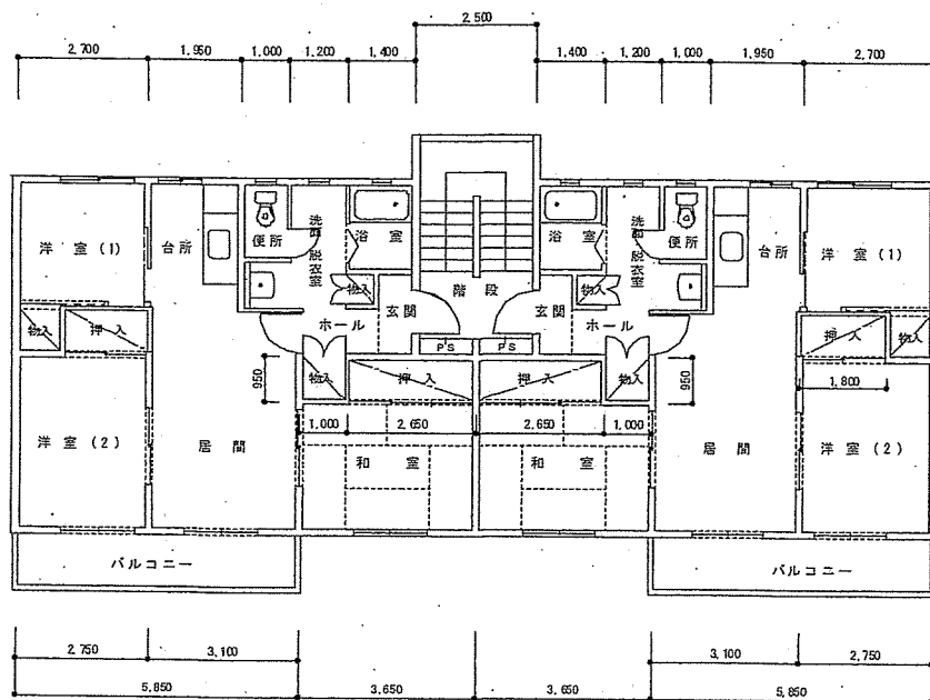
宿舎平面図 3LK S=1/X
