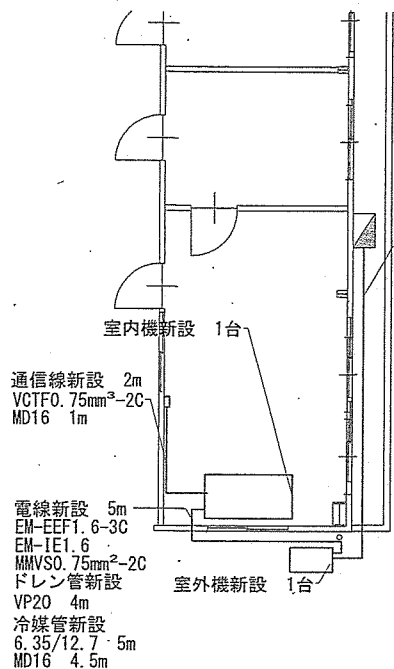
【新設 機械】平面詳細図 S=1/100
