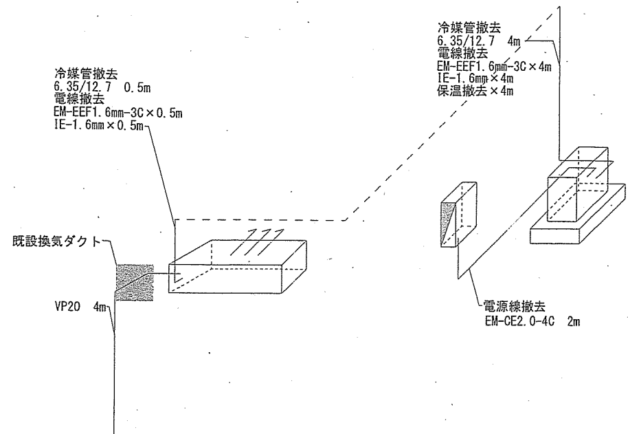
【撤去】配管系統図=1/50
