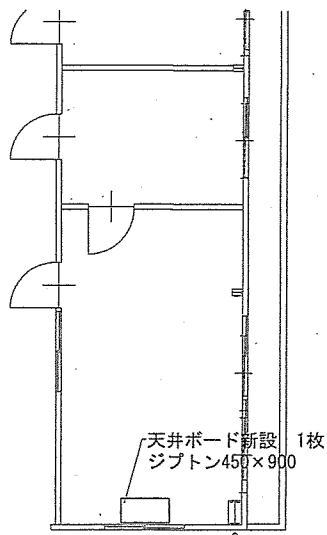
【撤去 建築】平面詳細図 S=1/100
