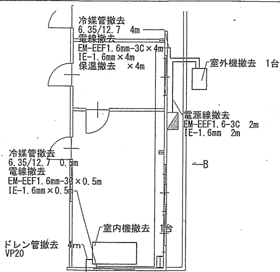
【撤去 機械】平面詳細図 S=1/100
