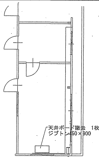
【撤去 建築】平面詳細図 S=1/100
