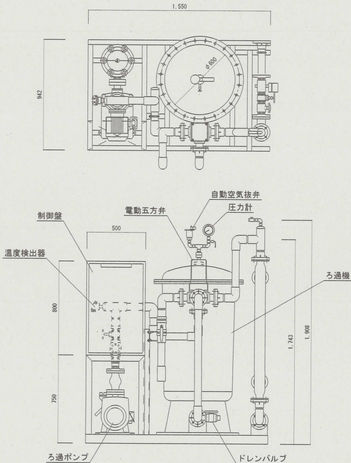
浴槽循環ろ過装置外形図
