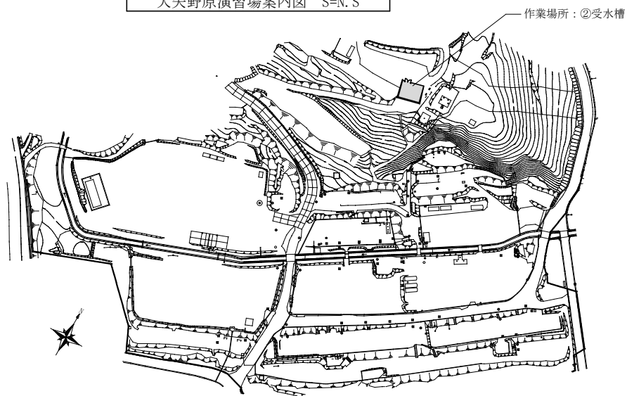
大矢野原演習場配置図 S=1/3,000
