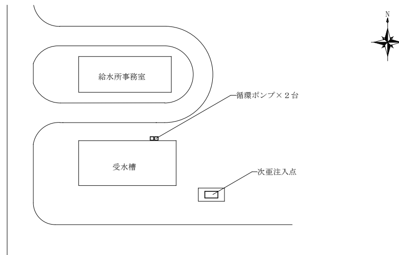
給水所平面図 S=1/600
