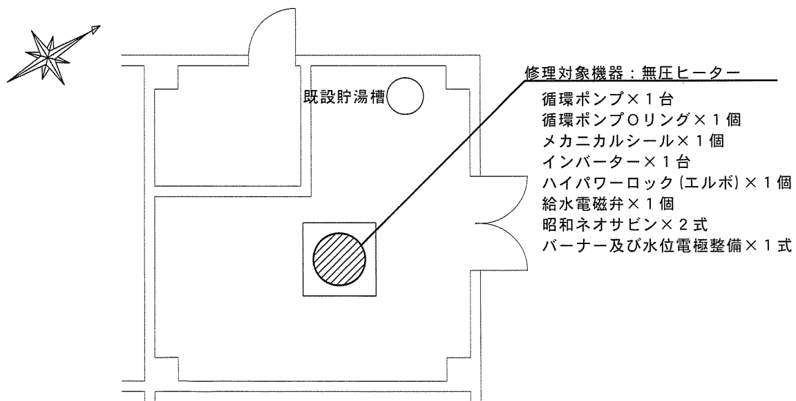
機械室平面図 S=1/100
