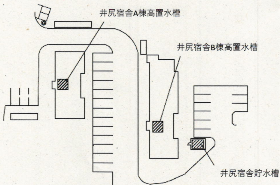
井尻宿舎配置図 1/400
