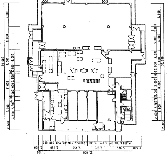
食堂平面図 1:400
