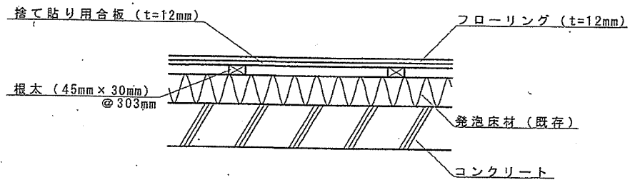
施工図
