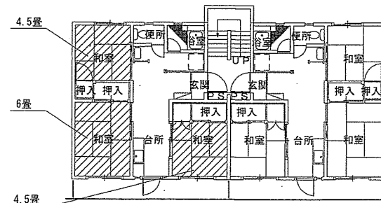
2、6号棟平面図 S=1:250
