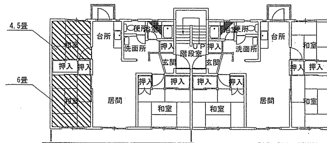
4号棟平面図 S=1:250
