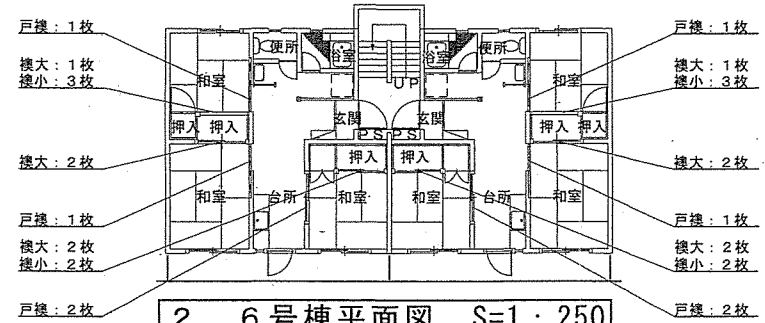
2、6号棟平面図 S=1:250
