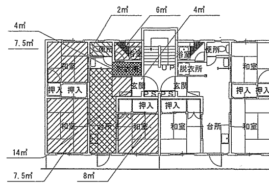
2、6号棟平面図 S=1:250
