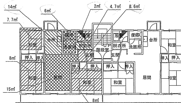
4号棟平面図 S=1:250
