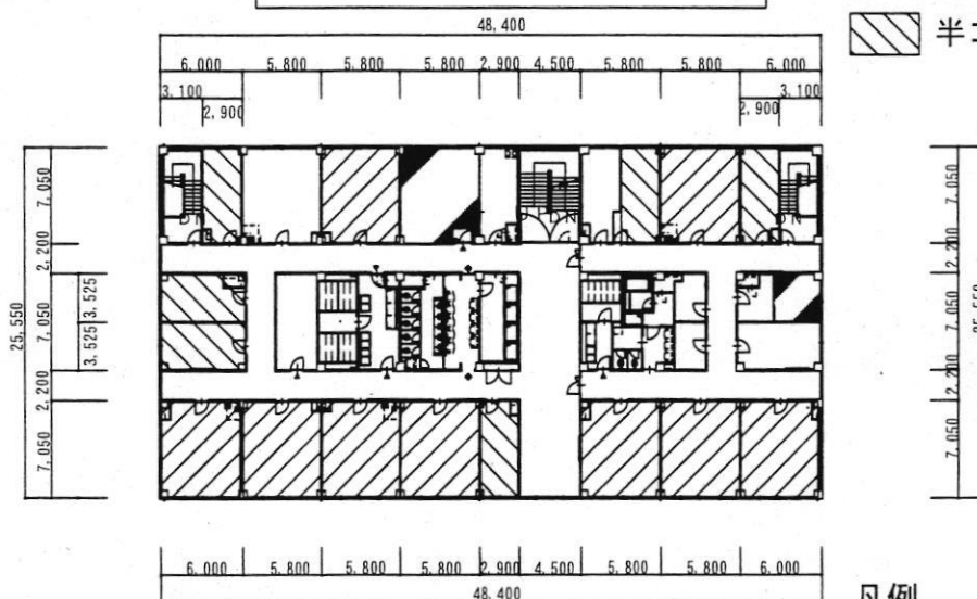
125号建物3階平面図 S=1 : 600
