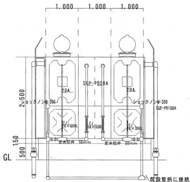
受水槽立面図 S=1:50
