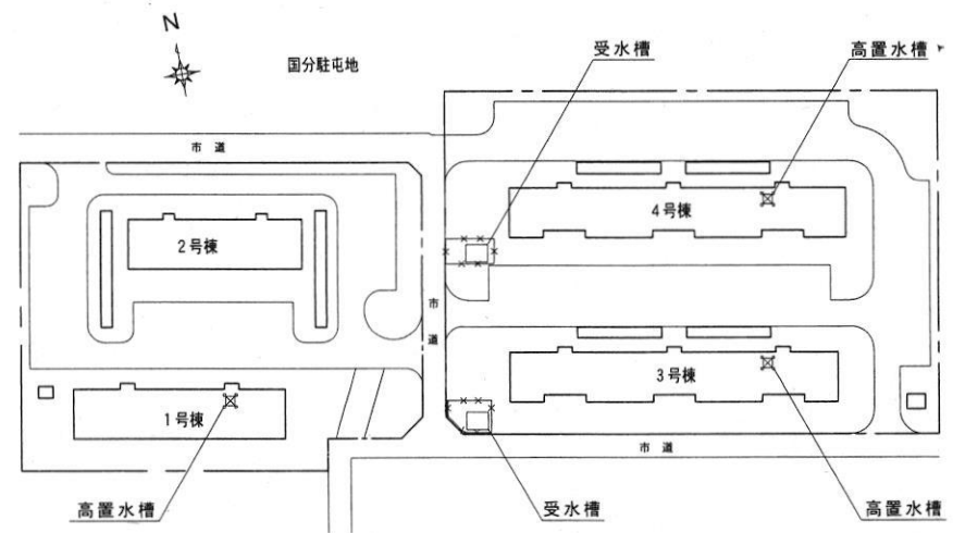
福島宿舎配置図 1:1,000
