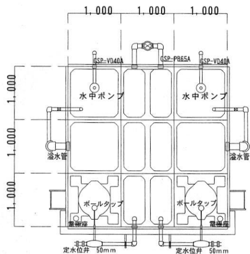
受水槽上部図 S=1:50
