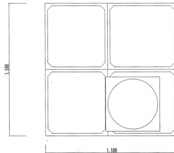
高置水槽上部図 S=1:20
