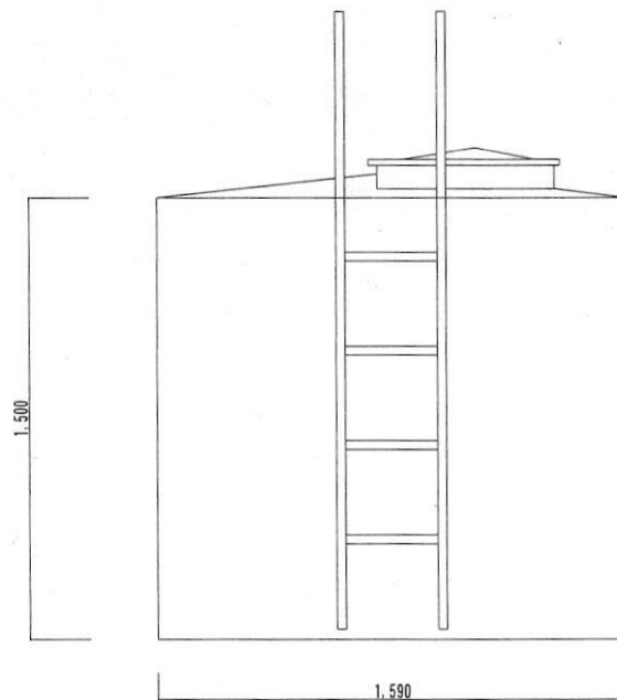
高置水槽立面図 S=1:20
