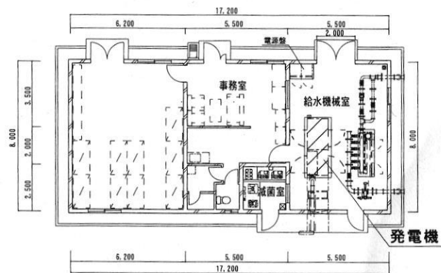
135号建物平面図 S=1:200
