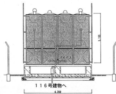
受水槽立面図 (S=1:100)
