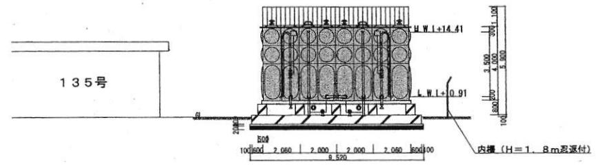
135号建物受水槽立面図 S=1:200
