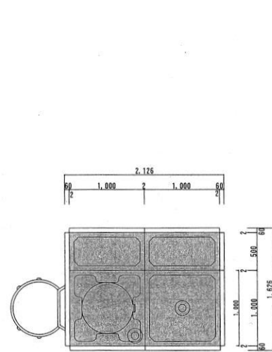
116号建物高置水槽平面図 S=1:50
