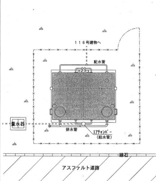
受水槽平面図 (S=1:100)
