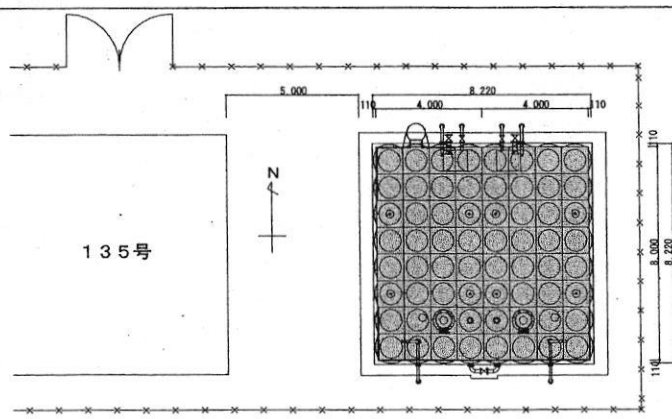
135号建物受水槽平面図 S=1:200
