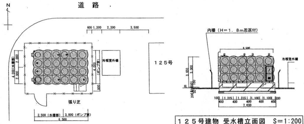
125号建物 受水槽平面図 S=1:200
