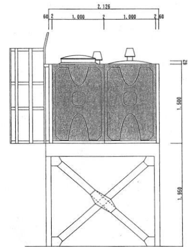
116号建物高置水槽立面図 S=1:50
