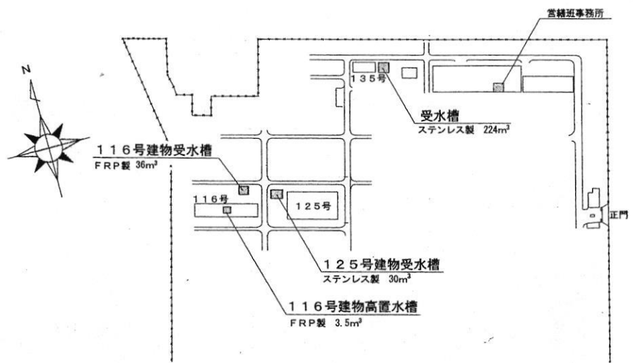
配置図 S = 1 : X
