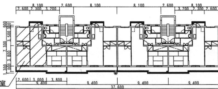
広瀬宿舎2階平面図 S=1:400
