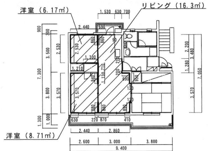
標準詳細図 S=1:200
