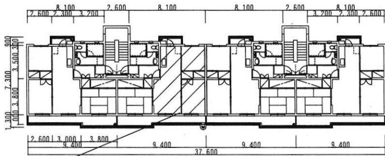
広瀬宿舎1階平面図 S=1:400
