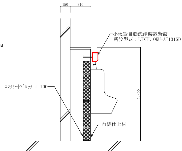
施工後 S=1/30
