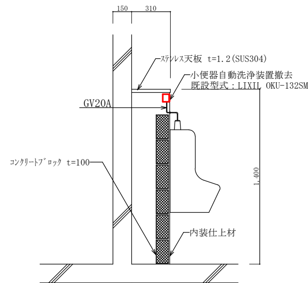
施工前 S=1/30
