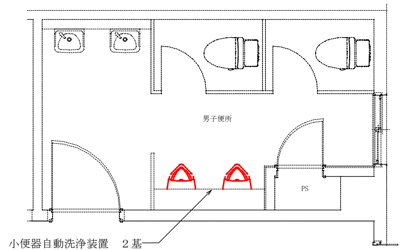
男子便所 詳細図 S=1/50
