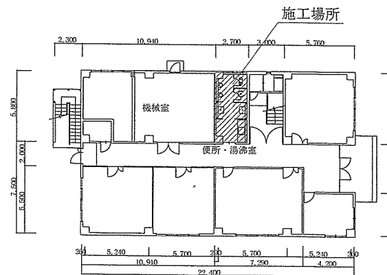
長崎合同庁舎 1階平面図 1/300
