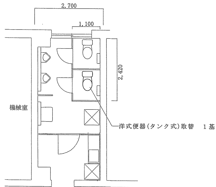
1階男子便所 施工平面図 1/60
