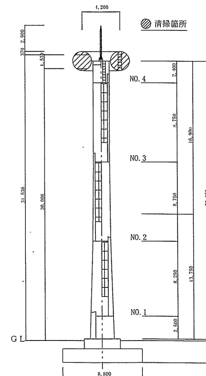
断面図 S=1:300
