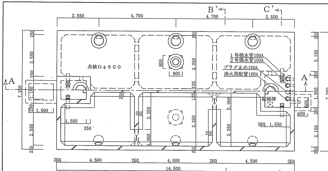
駐屯地受水槽 平面図 1/100
