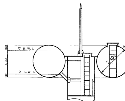
高架水槽断面図 S=1:100
