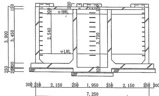
C-C' 断面図 1/100
