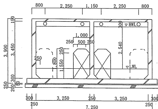
B-B' 断面図 1/100
