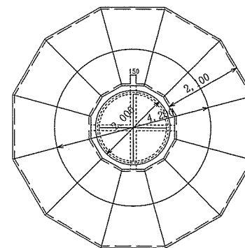
高架水槽平面図 S=1:100
