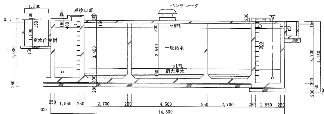
A-A' 断面図 1/100
