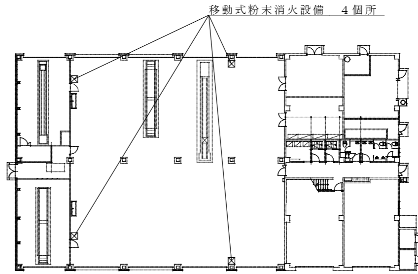
147号建物 S=1:450
