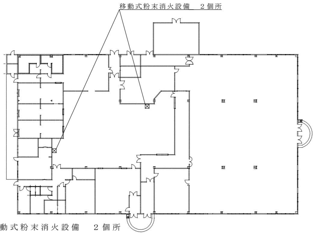
108号建物 S=1:500
