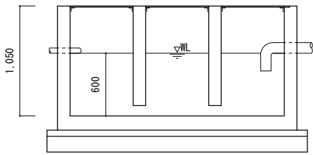
No.5 油分離槽
