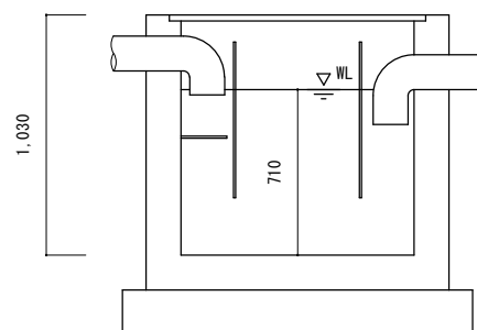
No.2 油分離槽
