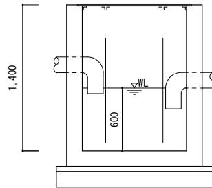
No.9 油分離槽
