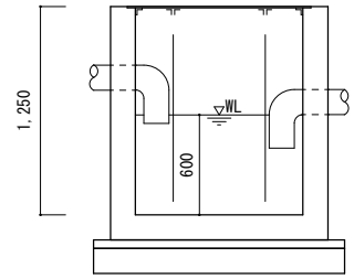
No.6 油分離槽
