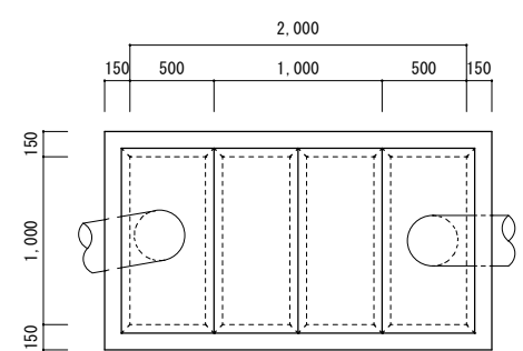
No.2 油分離槽
