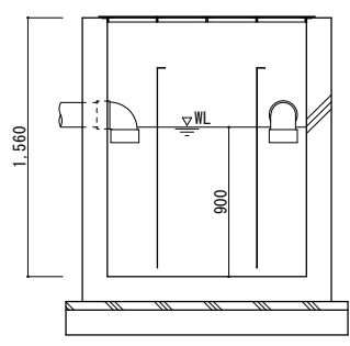
No.1 油分離槽
