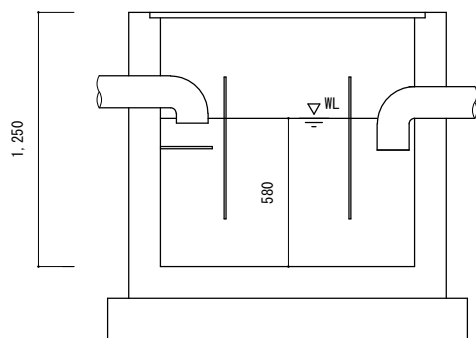
No.5 油分離槽
