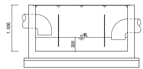
No.4 油分離槽
