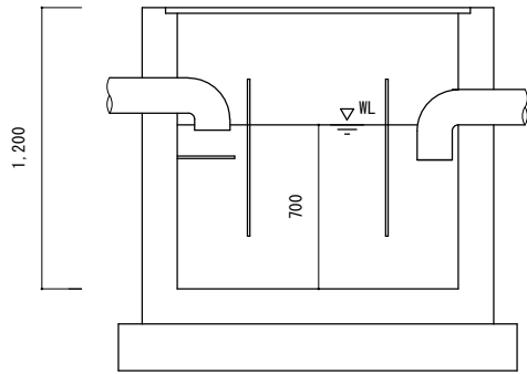
No.3 油分離槽
