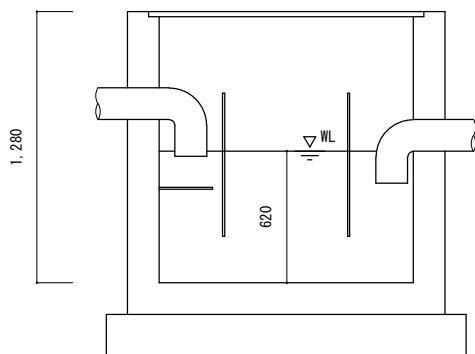
No.1 油分離槽
