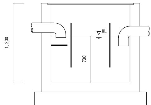
No.4 油分離槽
