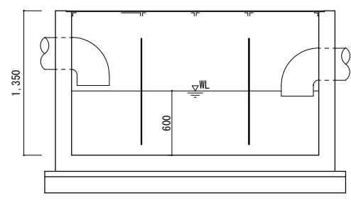
No.2 油分離槽
