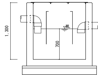
No.10 油分離槽
