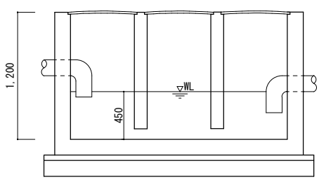
No.3 油分離槽
