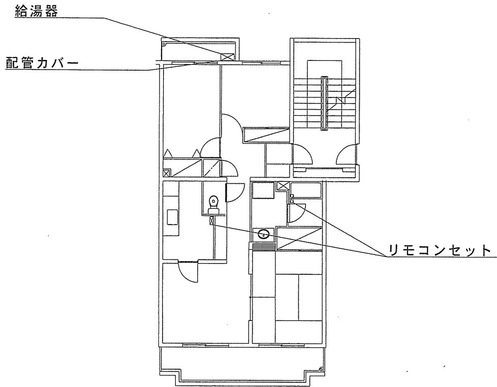
6号棟標準平面図 S = 1 : X
