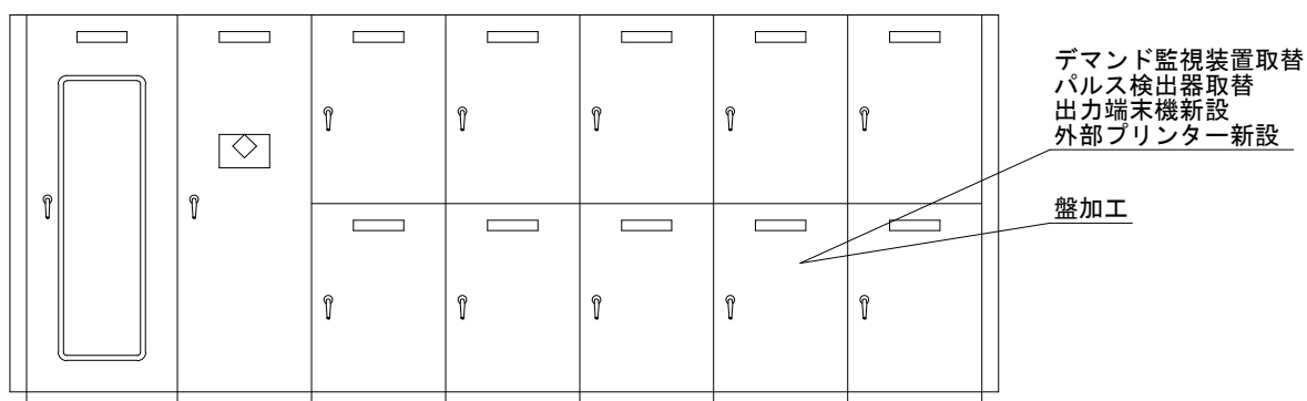
受電所屋内キュービクル 正面図 S = 1 / 50
