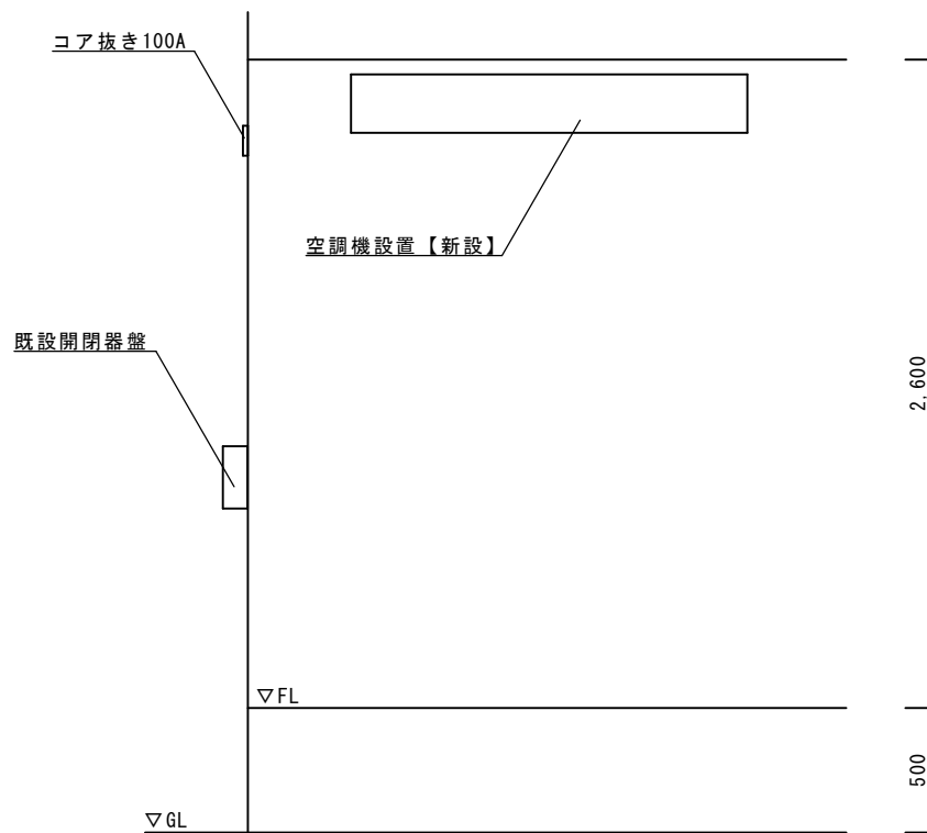
施工場所⑤ 取付詳細図
