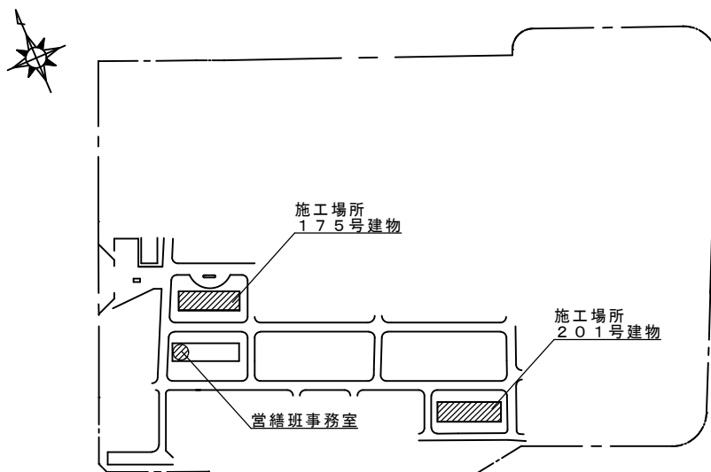
配置図
