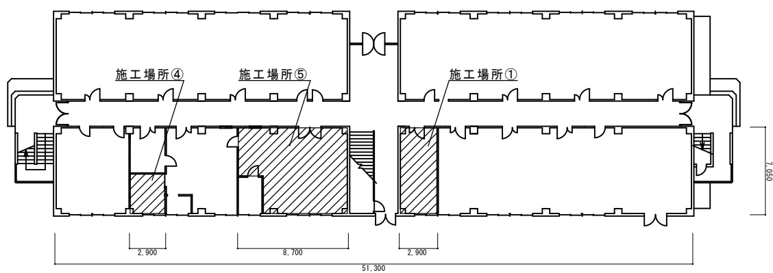
175号建物1階平面図
