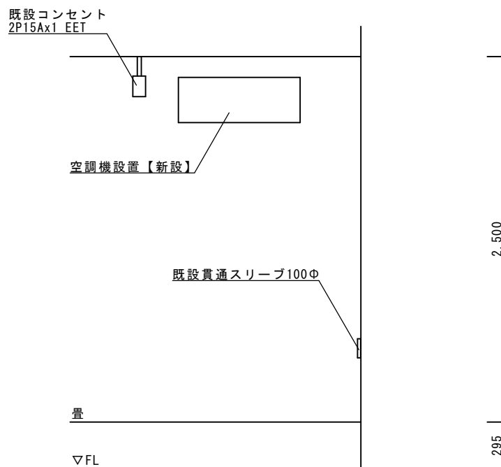
施工場所④ 取付詳細図
