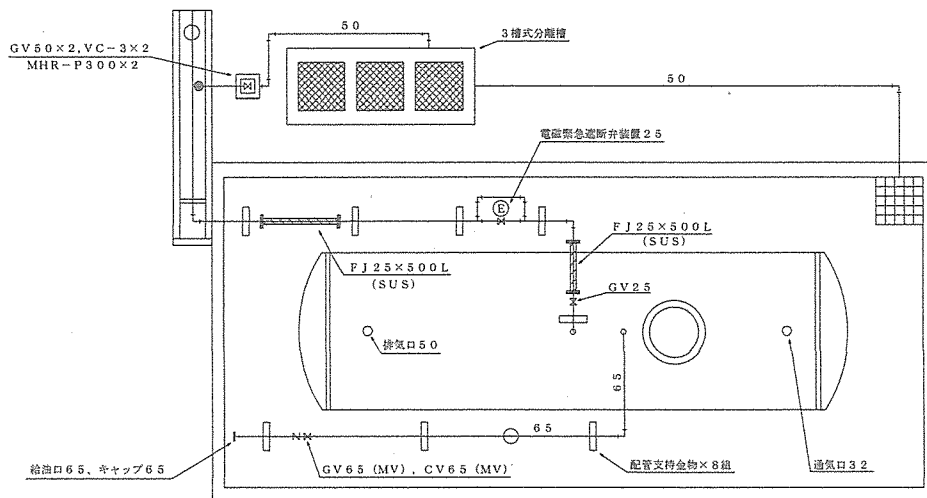
地上タンク平面図 S=1/N
